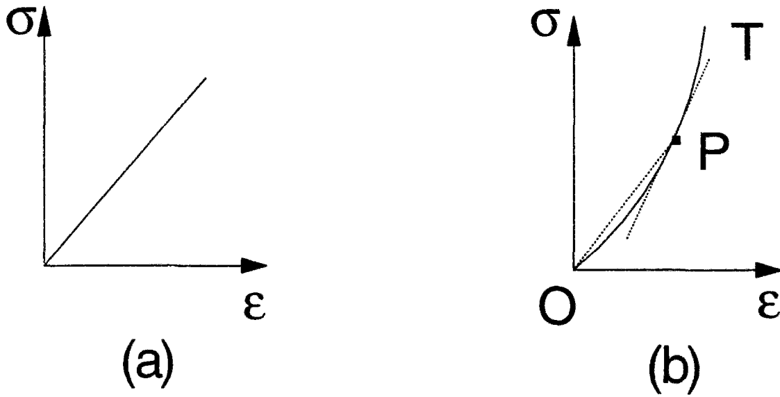
Figure 1.1: Courbes contraintes-déformations pour: a) matériau élastique linéaire, b) matériau élastique non-linéaire (Fjaer et al [1992])
