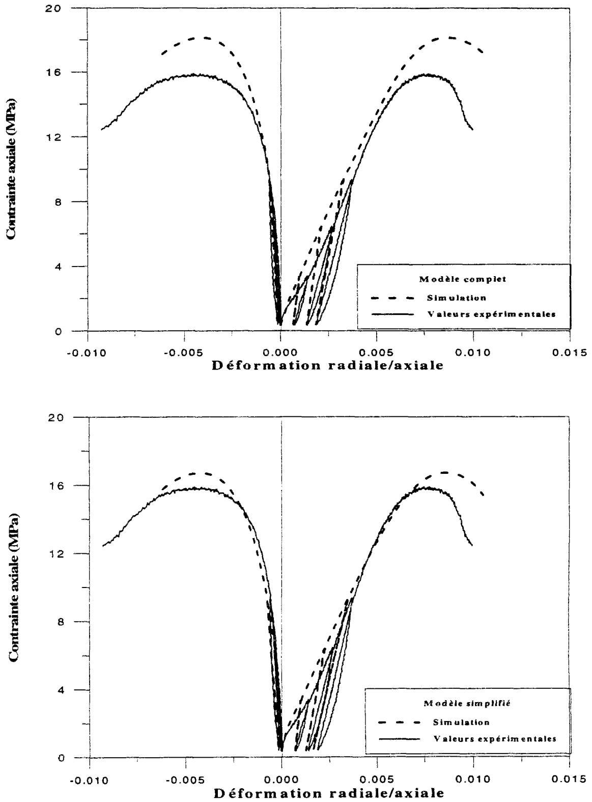
Figure 3.18: Simulation d'un essai de compression confiné à 0.4 MPa à partir des modèles complet et simplifié avec G=1825 MPa
