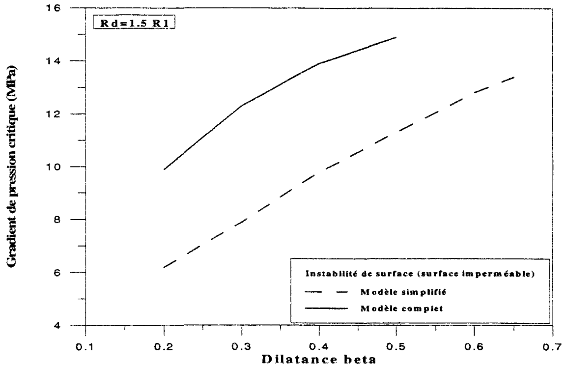
Figure 5.15: Représentation de la variation du gradient de pression critique par rapport à la dilatance
