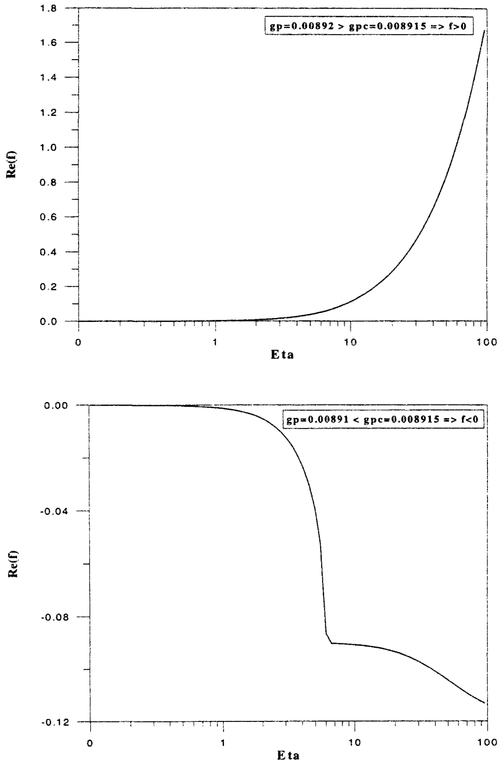
Figure 5.11: Représentation de l'évolution du coefficient de croissance f en fonction de \eta pour \beta \neq \mu (modèle simplifié)
