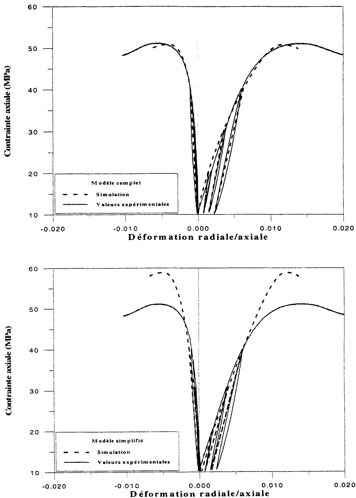
Figure 3.22: Simulation d'un essai de compression confiné à 10.3 MPa à partir des modèles complet et simplifié avec G=2840 MPa
