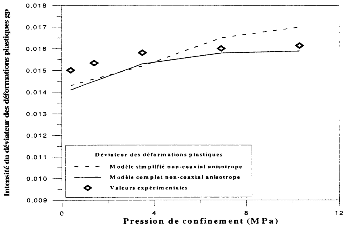
Figure 4.7: Représentation de l'évolution de (\theta_B, g_B^D) en fonction de la pression de confinement
