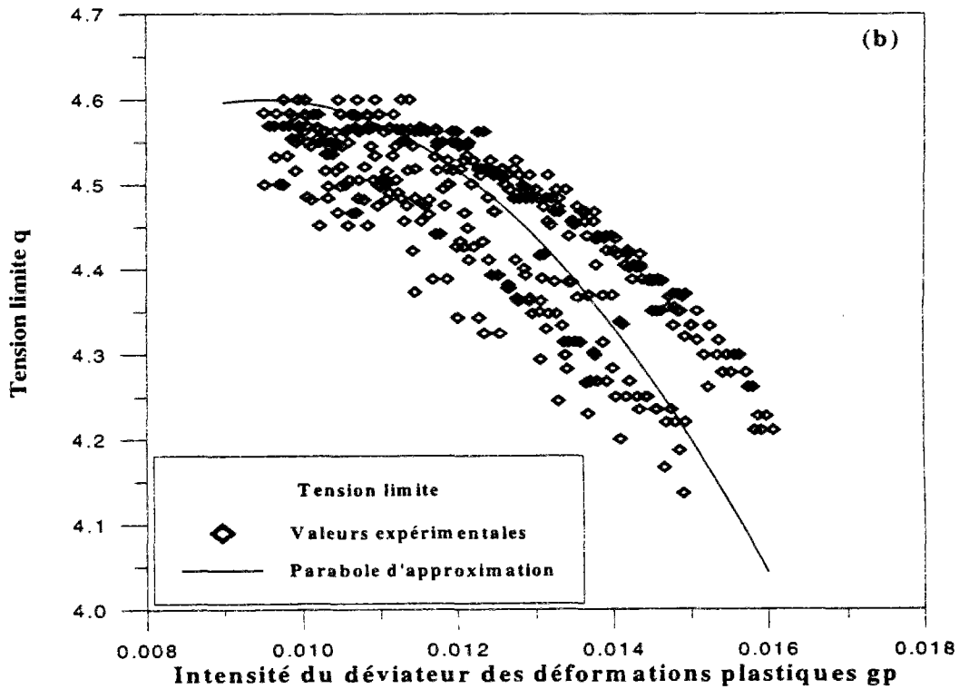
Figure 3.15: (a) Représentation des déformations radiales obtenues à partir de deux jauges perpendiculaires l'une par rapport à l'autre, (b) Evaluation du paramètre q par rapport aux déformations plastiques en régime radoucissant pour différentes pressions de confinement.
