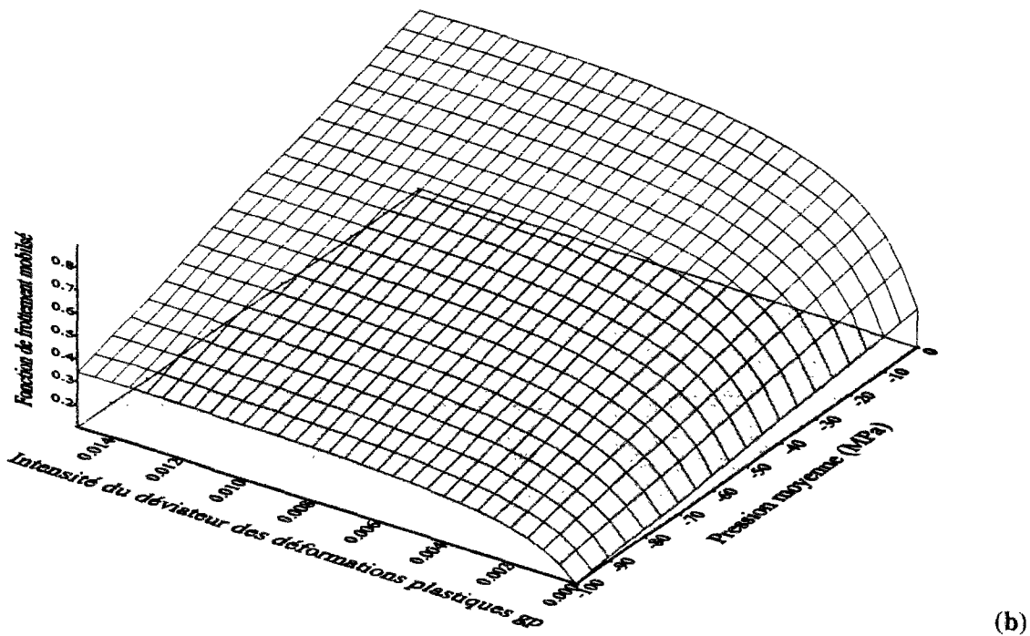
Figure 3.11: Représentation de la procédure de calage de la fonction de frottement pour différents essais en extension triaxiale: (a) \mu_e^0(g^P) = \mu_e(g^P, p) / \epsilon_e(p) , (b) \mu_e(g^P, p) pour les confinements 40, 45, 52.5 et 60 Mpa
