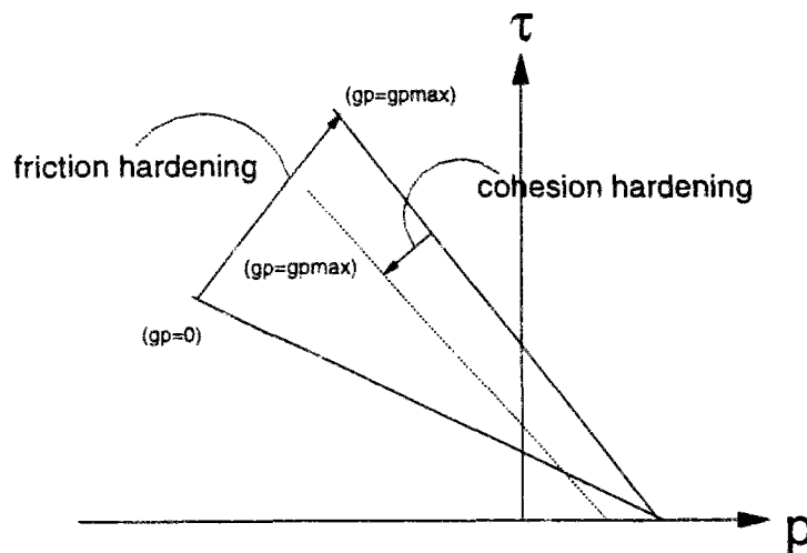
Figure 1.3: Critère de plasticité dans le plan (p, \tau) , écoulement isotrope et cinématique (Sulem et al [1995a])
