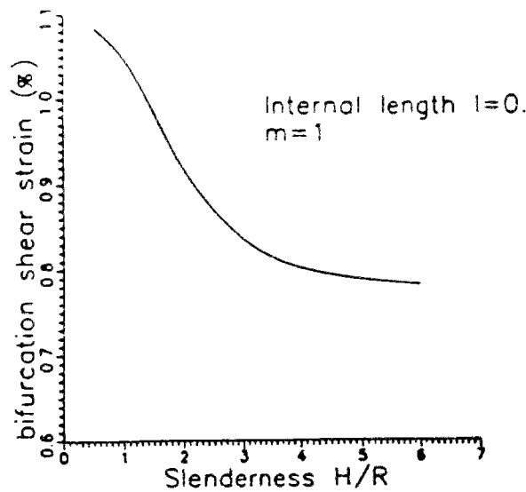
Figure 1.14: Effet de l'élanement sur la stabilité de l'échantillon. (Sulem et Vardoulakis [1990])
