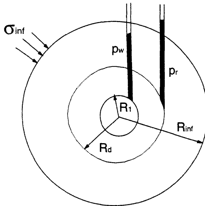
Figure 5.1: Illustration des contraintes autour d'un forage en phase de creusement ( p_r=p_w=constante ) (Sulem et Vardoulakis [1989])
