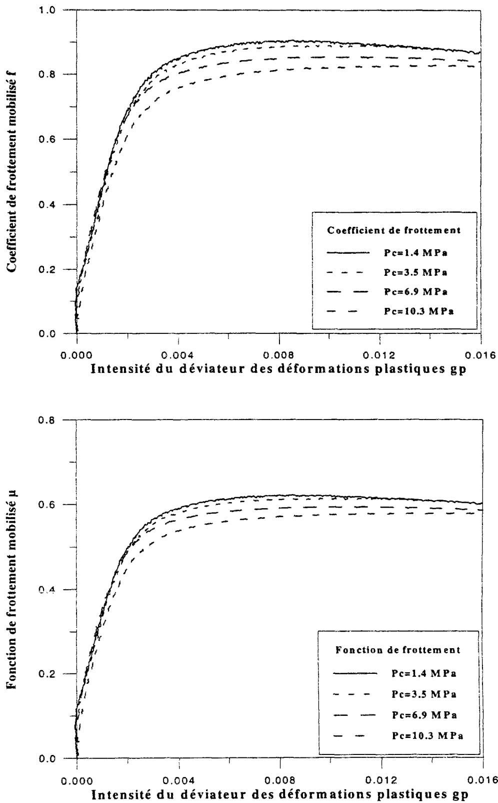
Figure 3.8: Evaluation du coefficient et de la fonction de frottement mobilisés pour différents confinements en compression triaxiale
