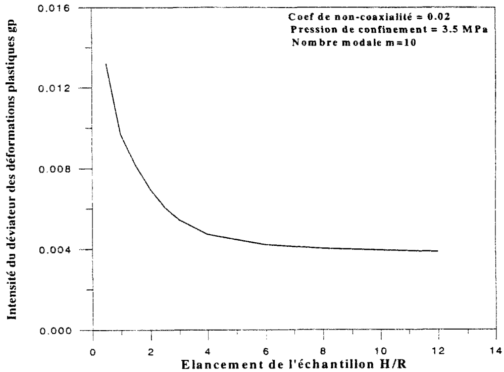
Figure 4.10: Représentation de l'intensité du déviateur des déformations plastiques g^p à la bifurcation en fonction du nombre modal m et de l'élanement de l'échantillon H/R (modèle simplifié)
