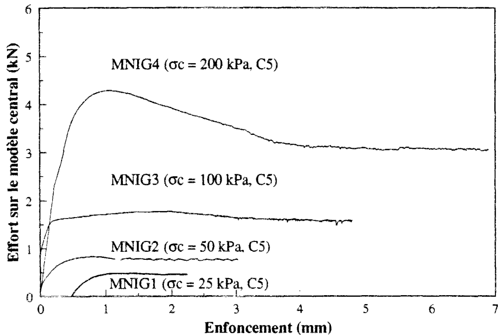
Figure 1 Influence de la contrainte de consolidation sur la réponse des cellules à 5 modèles : cas des modèles à fût rugueux et pointe conique
