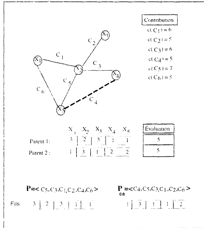
FIG. 5.3 – Exemple: Différentes Priorités pour Crossover
