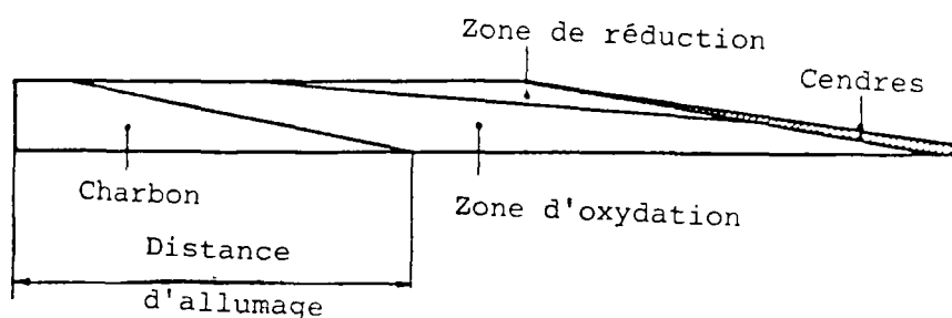
Figure 2-3 : Couche du charbon
