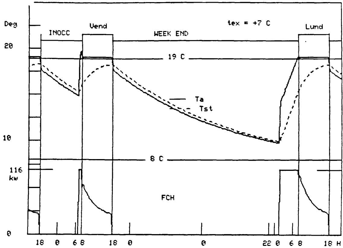
Figure 11-10 : Commande optimale avec compensation de la température extérieure : T_{ex} = 7^\circ\text{C}
