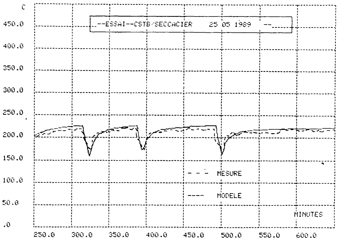
Figure 4-7 : Température des fumées (régime cyclique)
