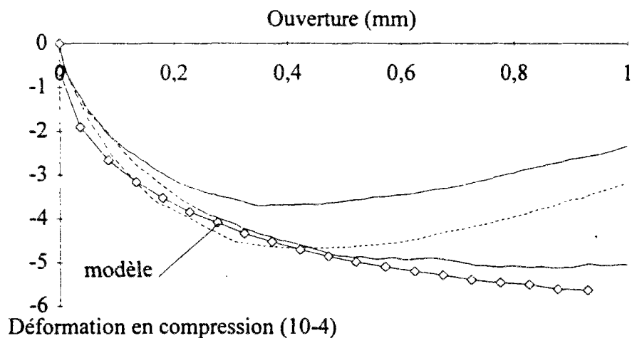
Figure 3.14 - Prédiction de la déformation en compression à 0,5 cm de la face supérieure. Prismes en béton B25BE40L, de dimensions 14 x 14 x 56 cm, entaillés de 1 cm dans la section médiane. Jauges de 60 mm.
