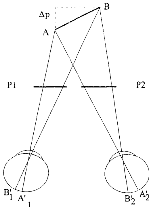
Figure 4.2.13 - Principe de la vision en relief (d'après [Desrues 1983]).
