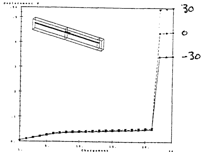
Figure 38 : Déplacement longitudinal v (mm) dans l'acier le long de la dalle pour des états successifs de chargement
