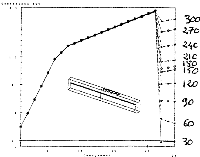
Figure 39 : Contrainte longitudinale \sigma_{VV} (MPa) dans le béton le long de la dalle pour des états successifs de chargement
