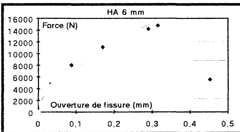
Figure 6 : Simulation de l'essai de traction sur un rond cranté de 6 mm
