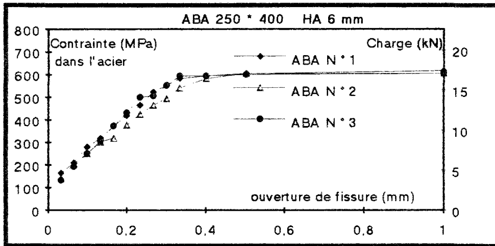
Figure 2 : Essai ABA sur HA 6 mm
