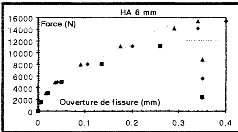
Figure 5 : Simulation de l'essai de traction sur un rond cranté de 6 mm
