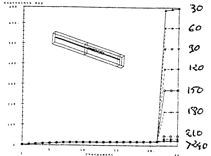
Figure 40 : Contrainte longitudinale \sigma_{VV} (MPa) dans l'acier le long de la dalle pour des états successifs de chargement
