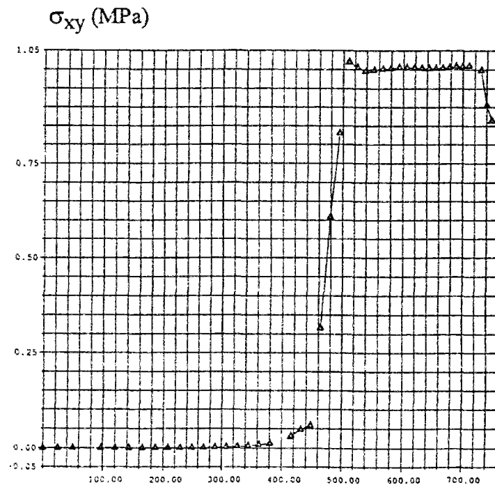
demi-longueur (mm) entre deux fissures Figure 22 : second chargement (abaissement de température dans le béton) \Delta\theta = 30 \text{ K}
