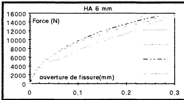
Figure 4 : Simulation de l'essai de traction sur un rond cranté de 6 mm
