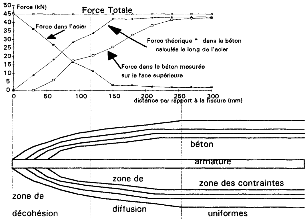
Figure 30 : Représentation de la force dans le béton, dans l'acier le long de la dalle pour le chargement provoquant la rupture du béton
