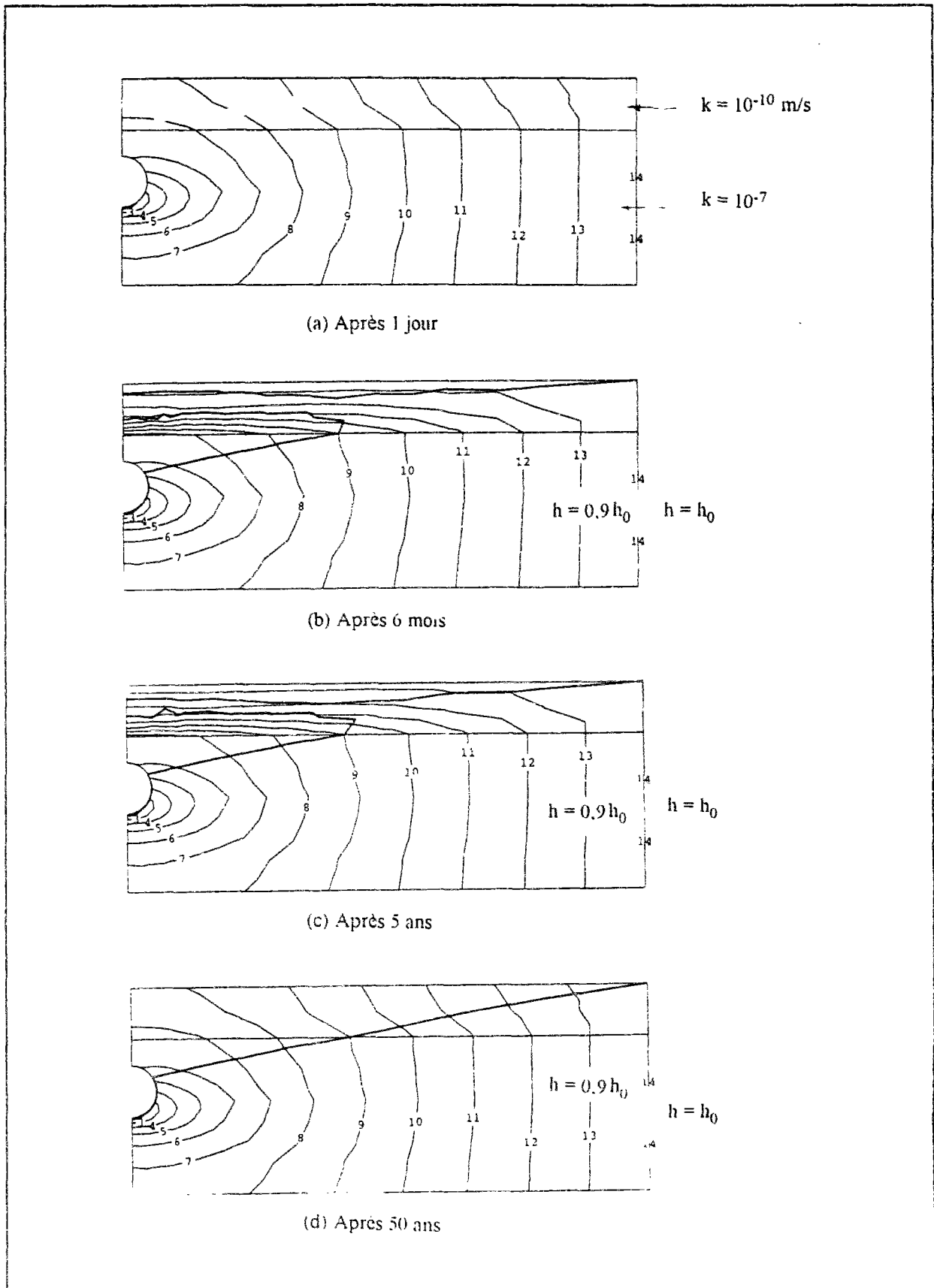
Figure II.51 : Evolution du régime hydraulique de l'écoulement vers un tunnel situé dans un massif surmonté par une couche moins perméable.
