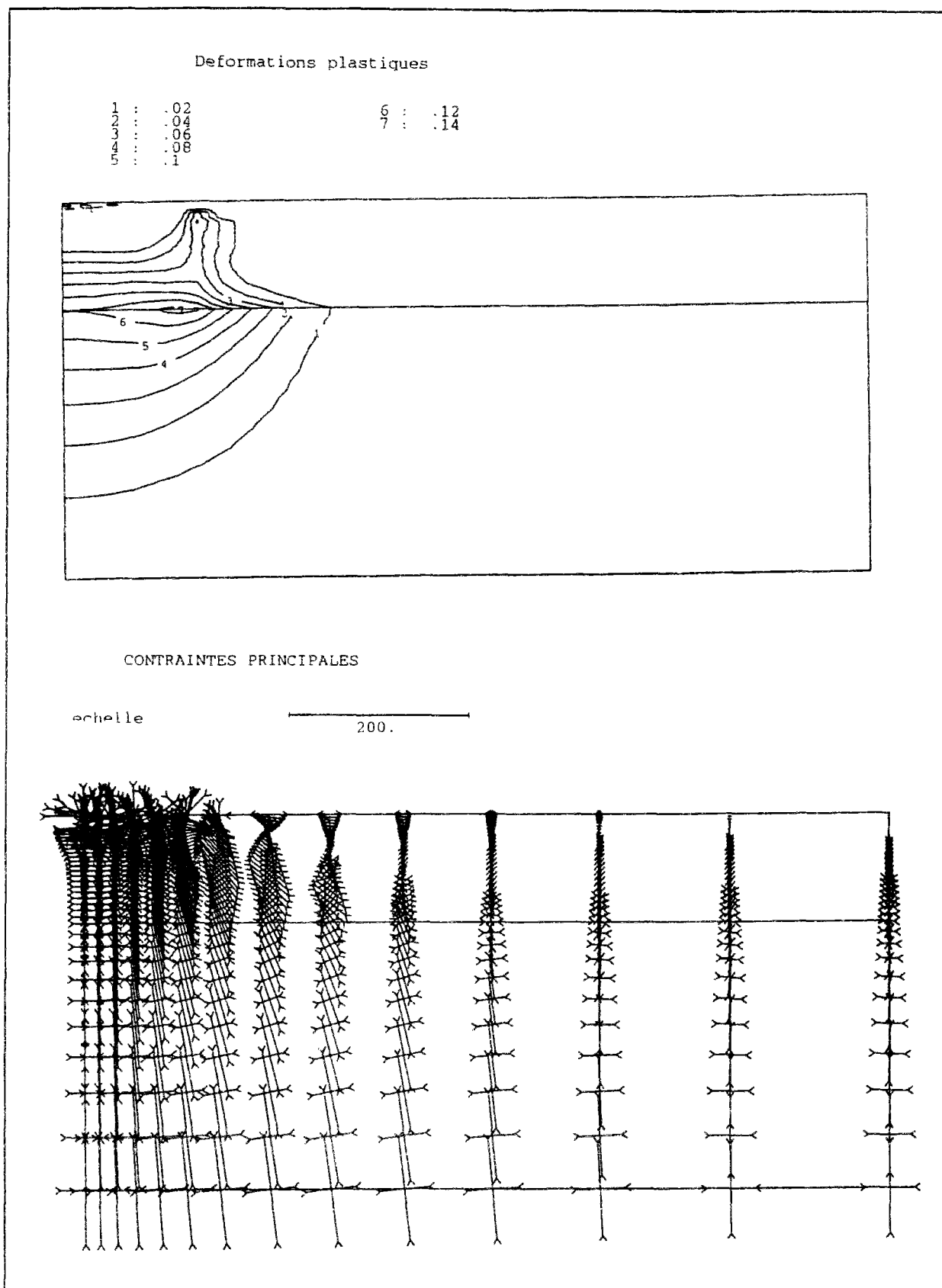
Figure C.3.3 : Résultats obtenus en termes de déformations plastiques (volumiques) et en termes de contraintes principales, par un calcul mécanique avec le modèle MELANIE pour l'exemple de la fondation.
