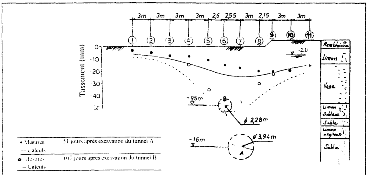
Figure IV.27 : Evolution de la cuvette de tassement de surface obtenue par Ohta et al. (1985).
