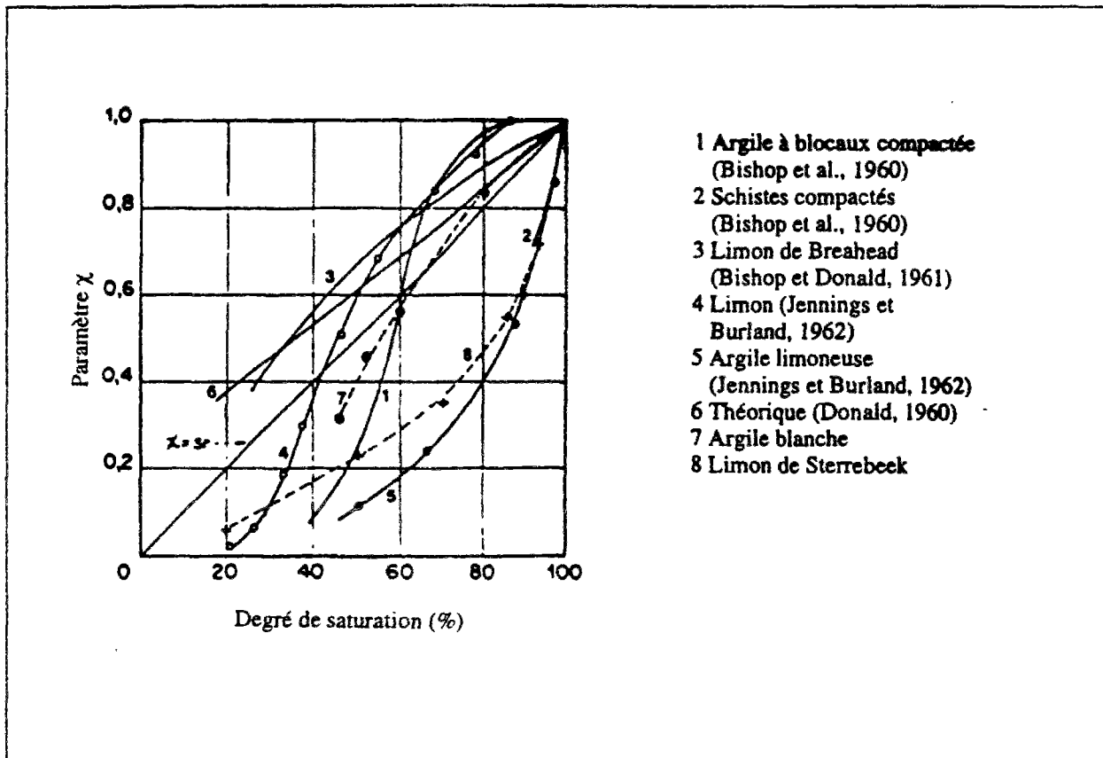
Figure C.4.1 : Variation du coefficient \chi de Bishop avec le degré de saturation pour différents matériaux (Zerhouni, 1991)
