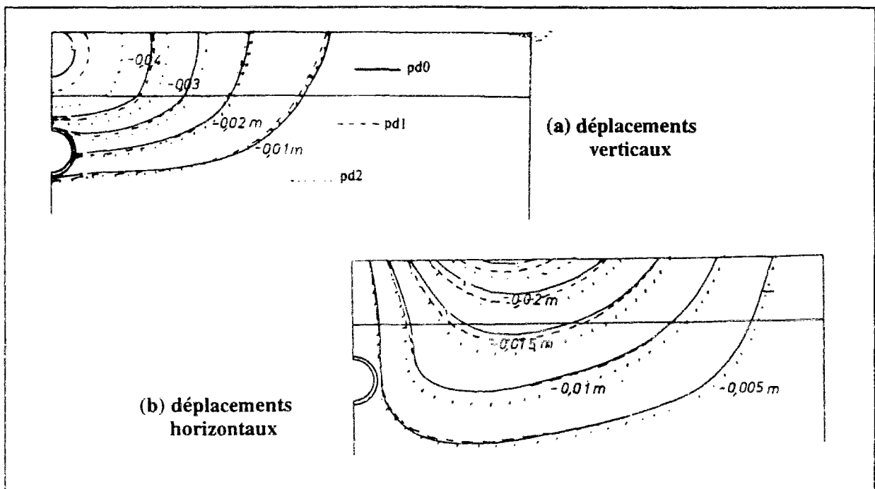
Figure VII.19a : Comparaison des tassements et des déplacements horizontaux à long terme autour du tunnel pour trois distributions verticales différentes de E'_h , E'_v et G'_{vh} .
