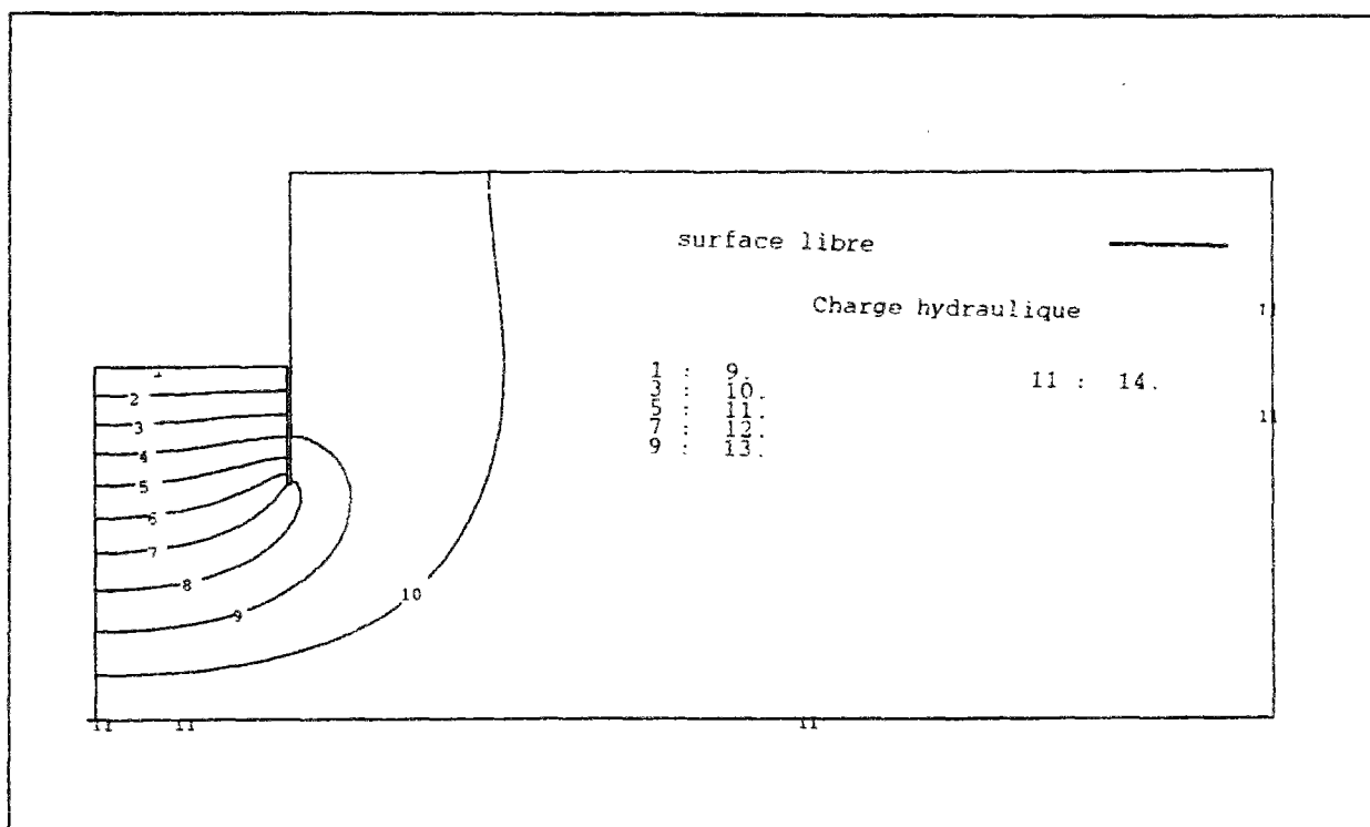
Figure C.3.4 : Résultats obtenus en termes d'équipotentiels obtenu par un calcul hydraulique dans un milieu indéformable pour le problème de la palplanche.
