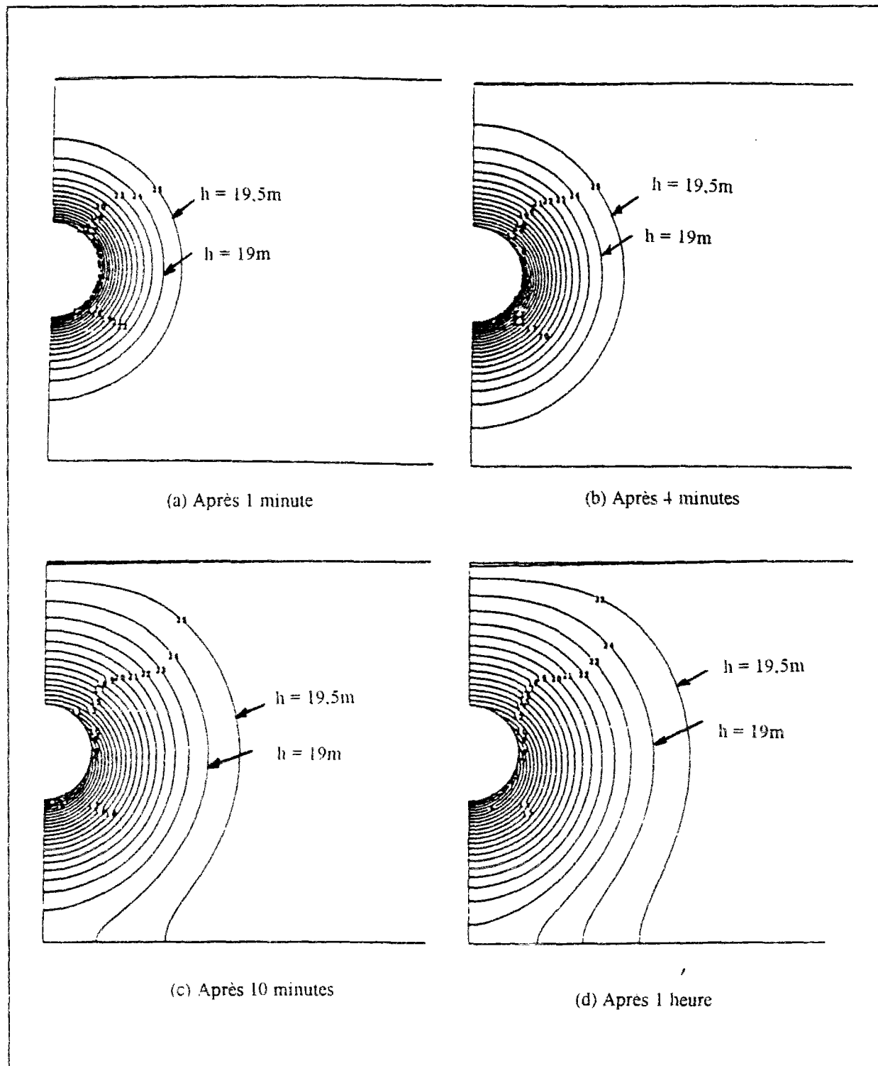
Figure II.45a : Evolution à court terme du réseau d'équipotentiellles autour d'un tunnel perméable (extrait du modèle).
