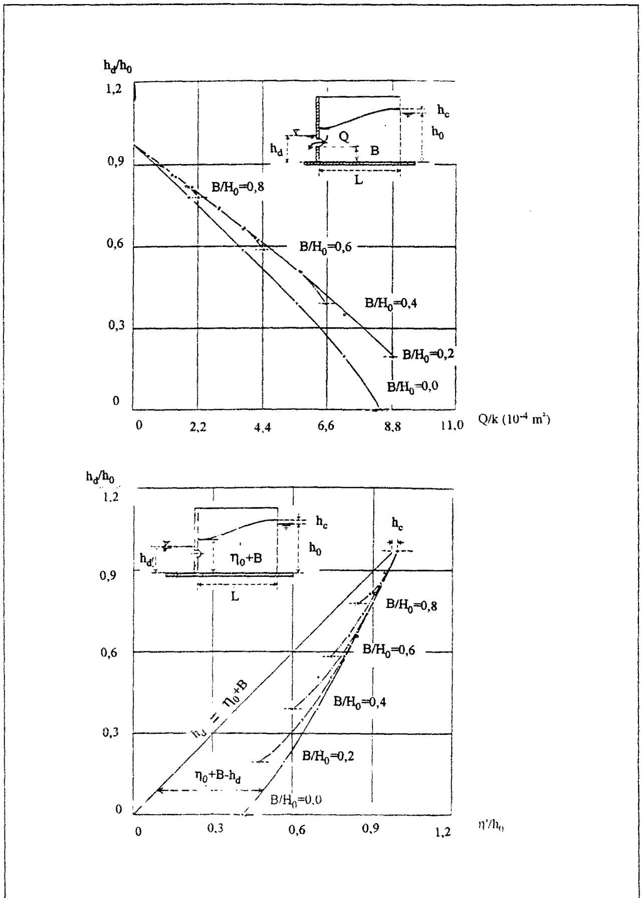
Figure I.24 : Méthode de Zeller (1954).
