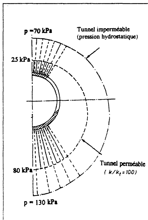
Figure II.28 : Distribution des pressions qui se développent sur le revêtement.
