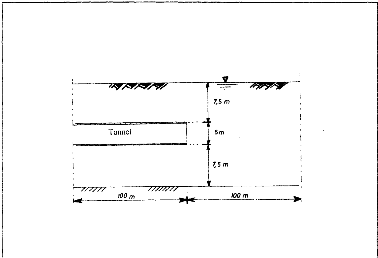
Figure II.40 : Configuration considérée dans l'analyse en coupe longitudinale.
