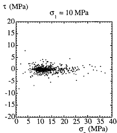
Figures IV-6-a IV-6-b : Contrainte tangentielle en fonction de la contrainte normale sur les joints
