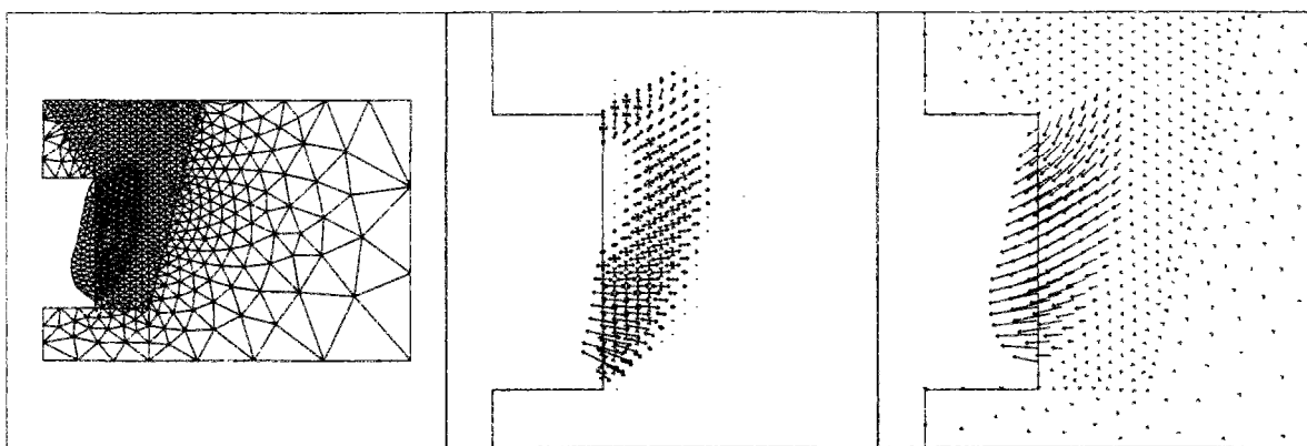
Figure 4-71. Maillage déformé, vitesses de déformation et vitesses de déplacement.
