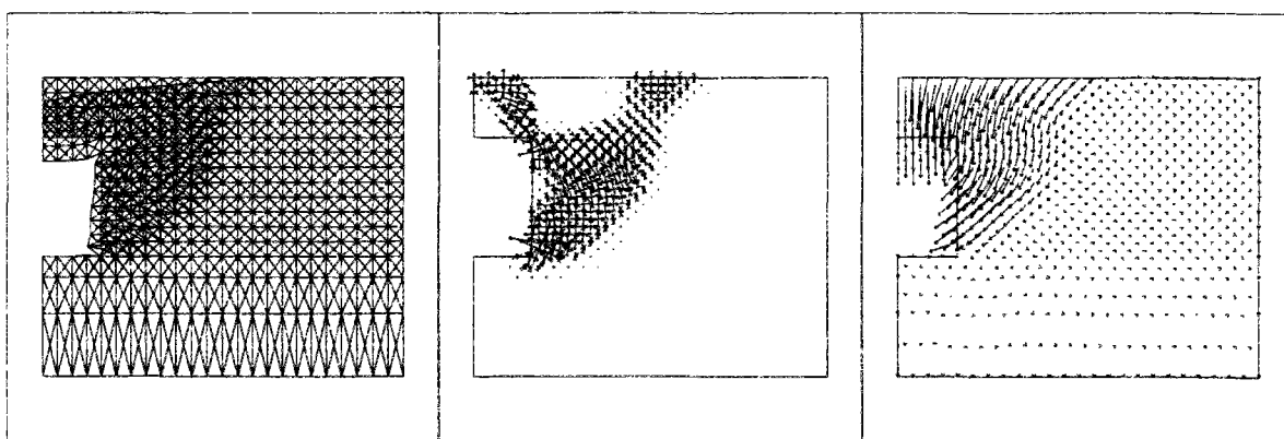
Figure 4-39. Maillage déformé, vitesses de déformation et vitesses de déplacement pour le cas de chargement n° 1 ( C/D=0,5 ).
