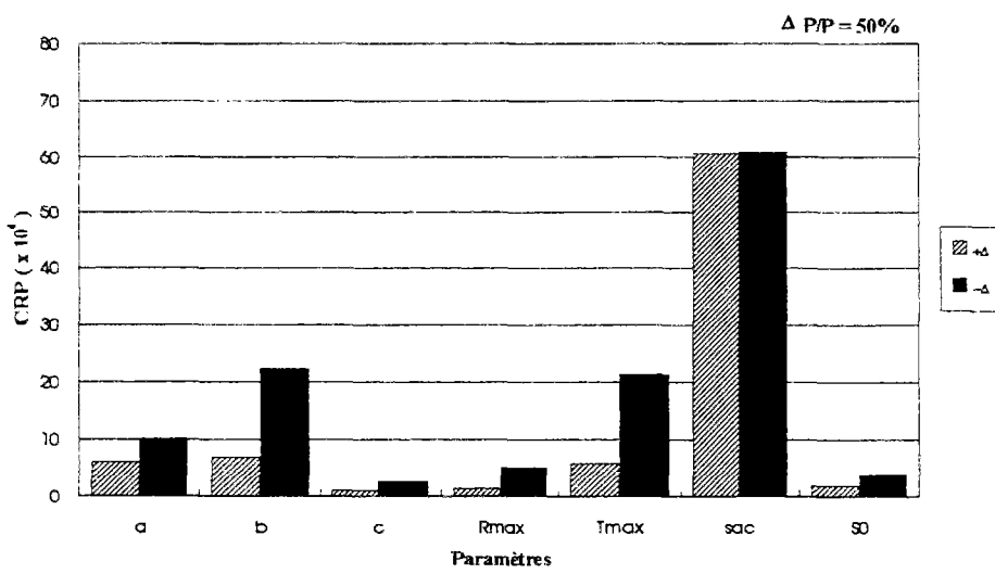
Figure A3.5: Illustration du coefficient de sensibilité du débit total CRP pour différentes perturbations des valeurs des paramètres
