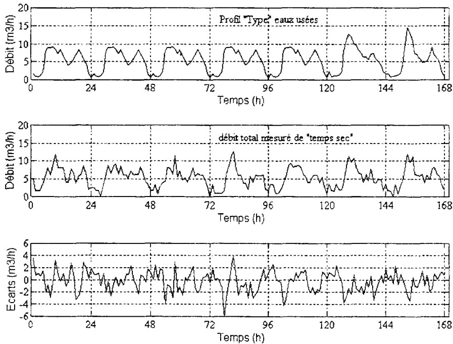
Figure 6.11: exemple des erreurs commises lors de l'estimation des eaux usées.
