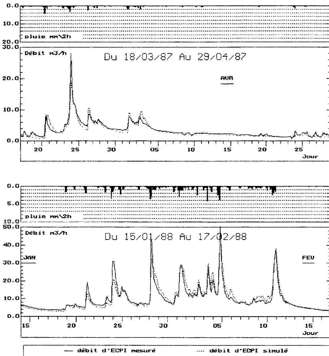
Figure 4.25 : représentation du débit mesuré et simulé obtenus en utilisant les paramètres issus du calage avec les débits inférieurs à 20 m 3 /h.
