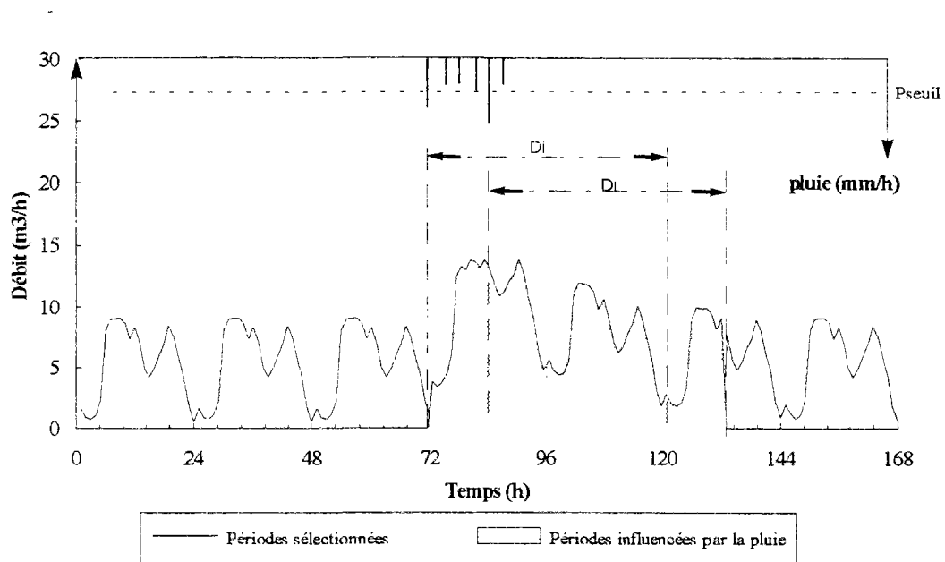
Figure 5.1: Illustration des critères de sélection des périodes représentatives des apports d'EU
