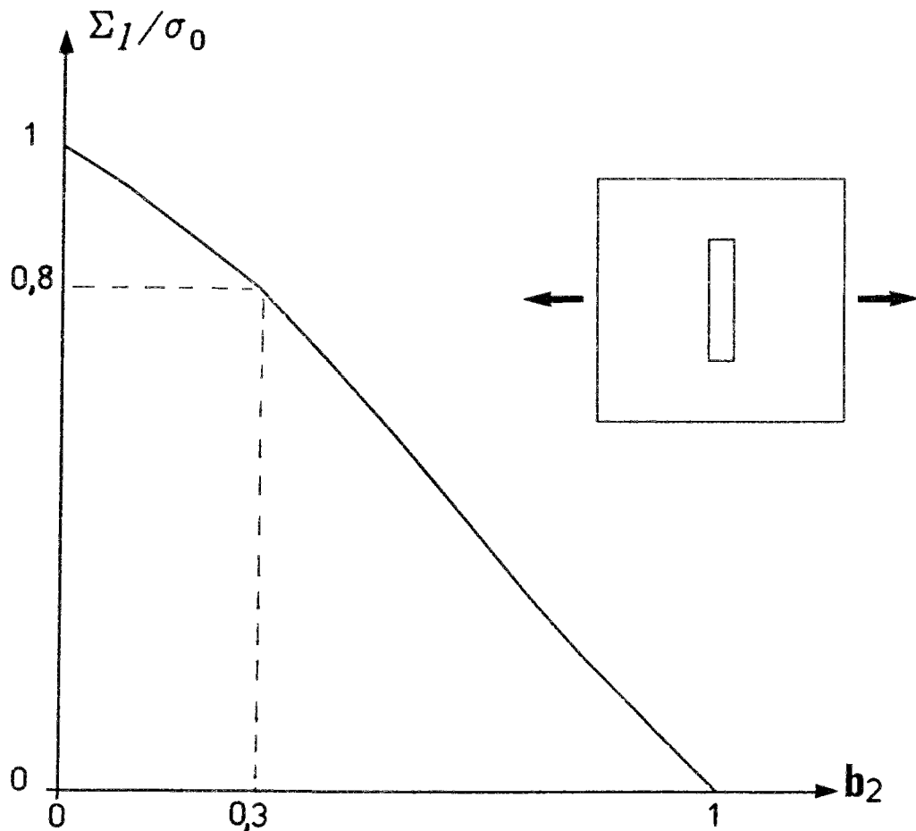
Figure 5 : variations de \Sigma_1/\sigma_0 en fonction b_2 .
