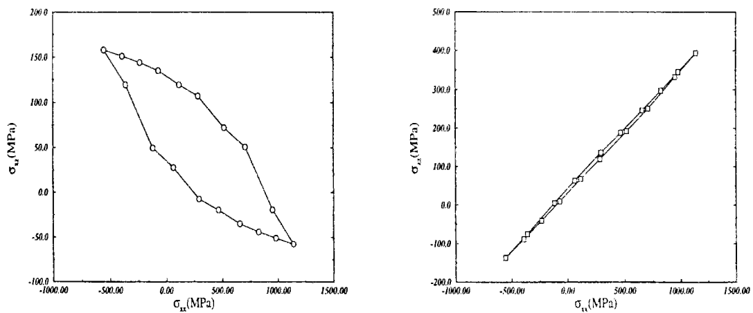
Figure 2.15: Cycle de contraintes au bord critique en glissement partiel P = 100\text{ N} et S_{max} = 600\text{ MPa} en fretting-fatigue
