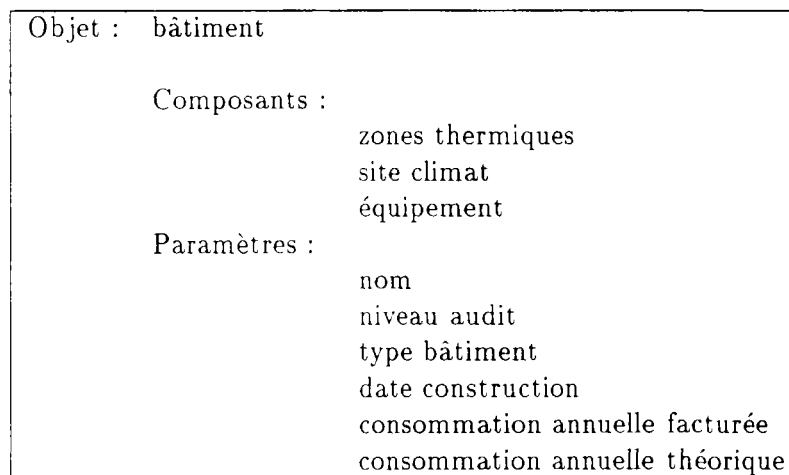
Figure II.1: L'objet bâtiment chauffé et occupé
