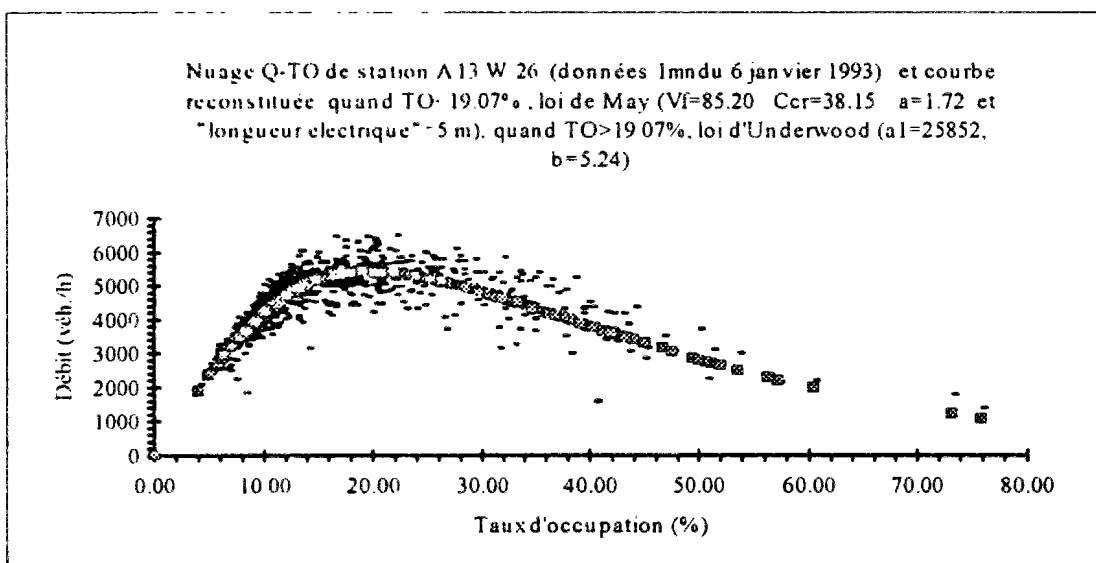
Fig.5.5 : Exemples de reconstitution du diagramme fondamental avec les données 1mn
