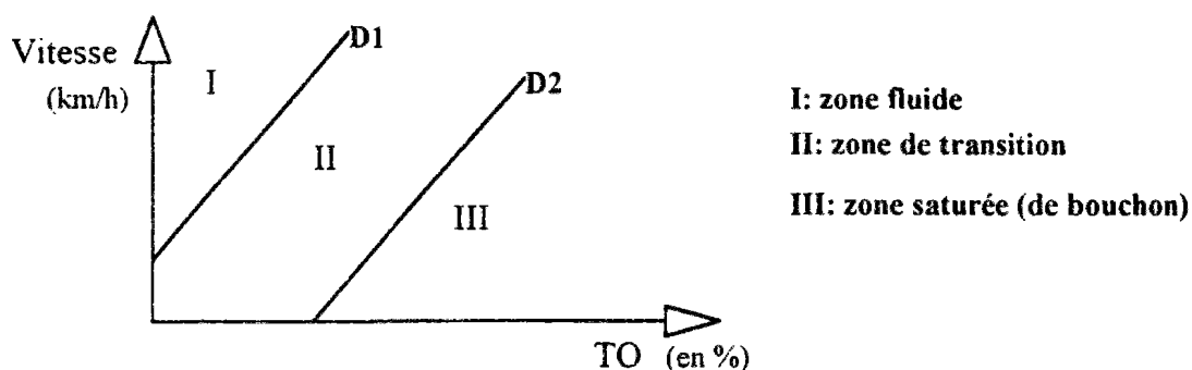
Fig.6.3 : Découpage des états du trafic en 3 zones sur le plan Vitesse - Taux d'occupation pour le déroulement d'un algorithme de DAB
