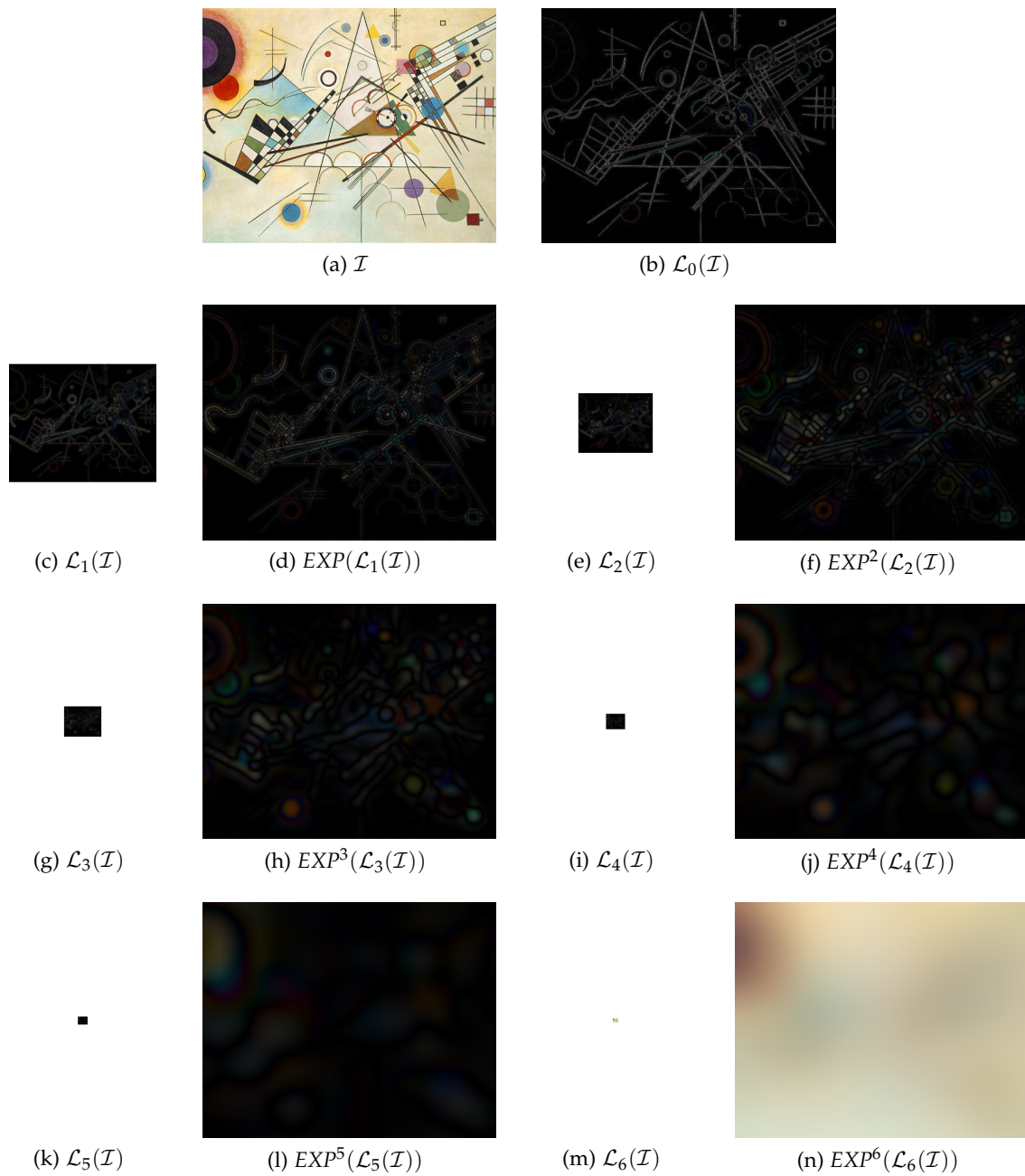
FIGURE 8.12 – Pyramide laplacienne de 7 niveaux d'une image 2D.
