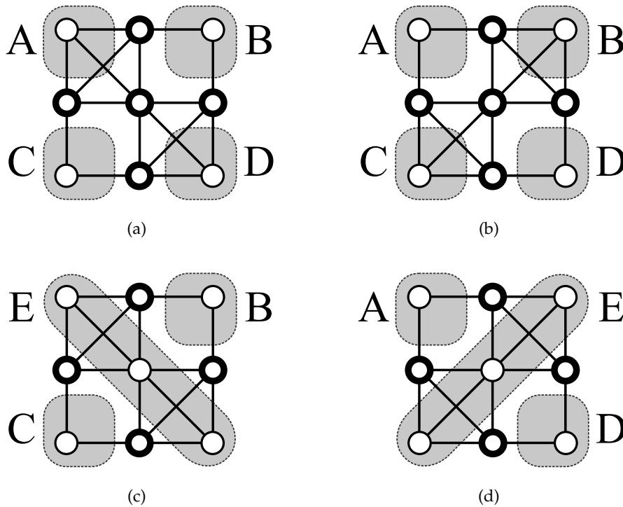
FIGURE 2.16 – (a,b) Ensemble frontière de sommets K (en gras) sur les deux grilles de fusion parfaite 2D, respectivement G_1 et G_2 . (c) K (en gras) après fusion des régions A et C sur G_1 ; (c) K (en gras) après fusion des régions B et D sur G_2 .
