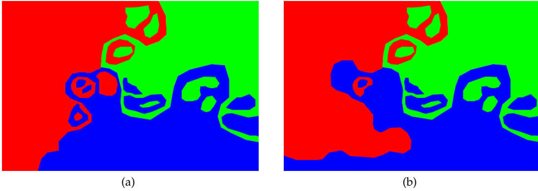
FIGURE 6.9 – (a) Etiquetage des pixels d'une image avec trois étiquettes (rouge, verte et bleue). (b) Etiquetage des pixels après une opération de (rouge,bleue)-swap (la région étiquetée verte n'a pas été modifiée).
