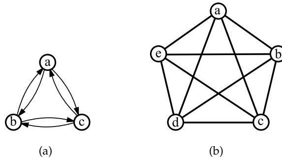
FIGURE 1.8 – (a) Graphe complet orienté à 3 sommets. (b) Graphe complet non-orienté à 5 sommets.
