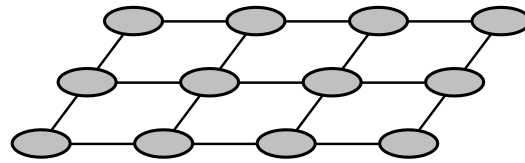
FIGURE 6.1 – Graphe non-orienté G = (\mathcal{P}, \mathcal{V}) équivalent à un champ de Markov.
