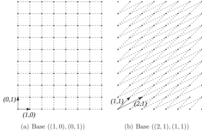
FIG. 1.3 – Exemples de repères pour les grilles
