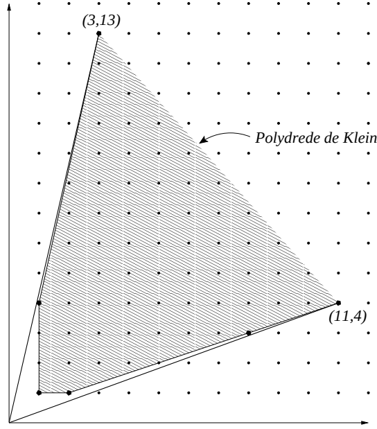
FIG. 1.12 – Exemple de polyèdre de Klein
