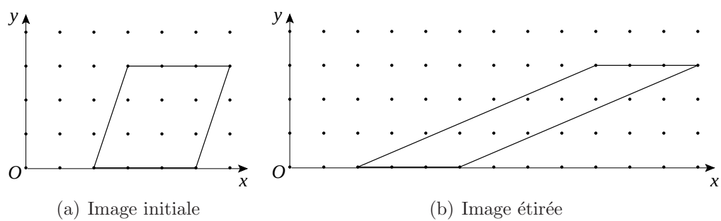
FIG. 1.4 – Exemple de transvection horizontale de coefficient 2
