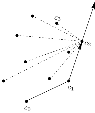
FIG. 1.14 – Exemple d'itération de la méthode du gift wrapping
