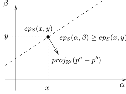
FIG. 4.1 – Un sous-gradient de ep_S
