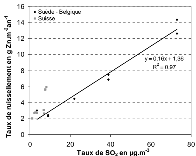
Figure 25 : Relation empirique entre taux de ruissellement du zinc et niveau de SO_2
