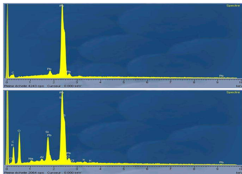
Figure 84 : Spectres EDS du plomb neuf, avant exposition (en haut) et après exposition (en bas)
