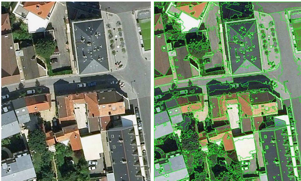
Figure 118 : Segmentation de l'image en régions de radiométries homogènes – Photo InterAtlas 2005
