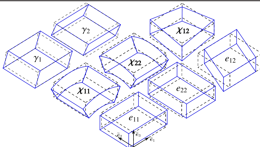
Figure 1.1 – Les déformations volumiques associées aux déformations généralisées (le gauchissement n'est pas représenté pour \gamma )
