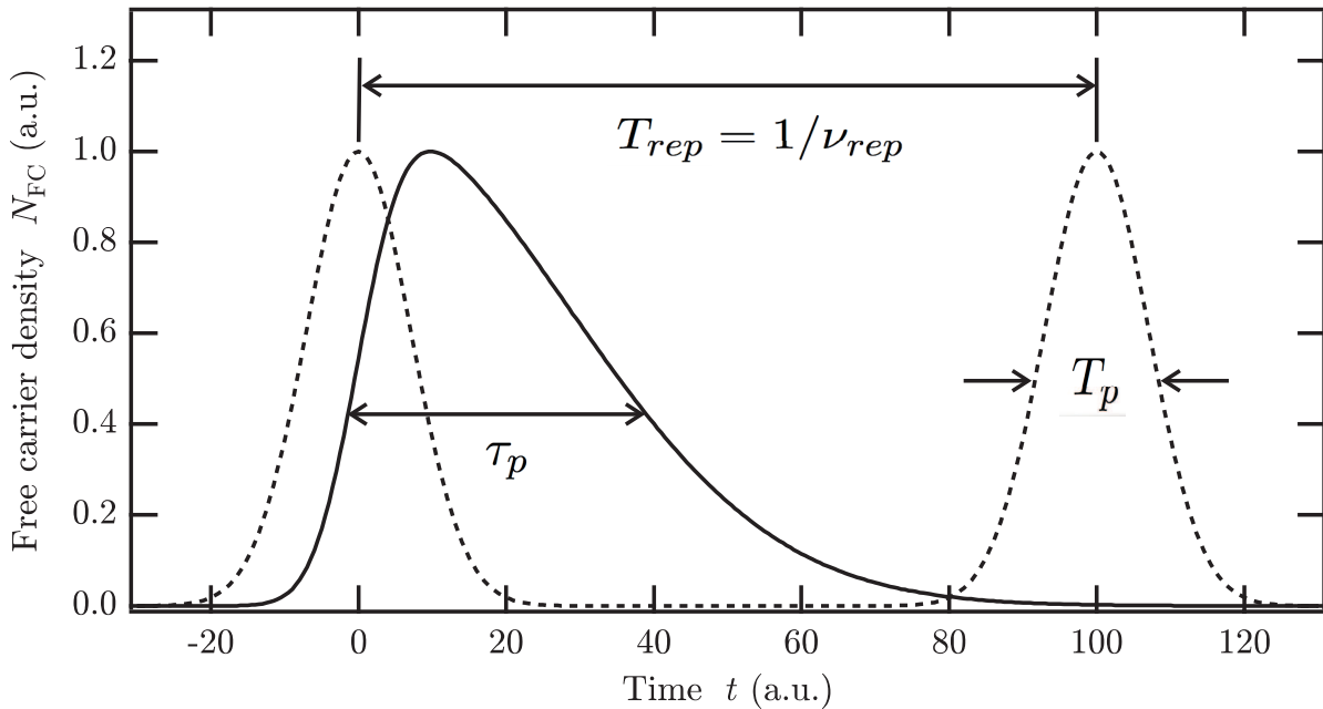
Figure 1.3. Représentation graphique de l'évolution temporelle de la densité de porteurs libres (trait continu) générés par absorption à deux photons d'impulsions (pointillés) délivrées par un laser avec une fréquence de répétition \nu_{\text{rep}} . Le temps de vie des porteurs est \tau_p et T_p représente la durée caractéristique d'une impulsion (la largeur totale à 1/e par exemple).
