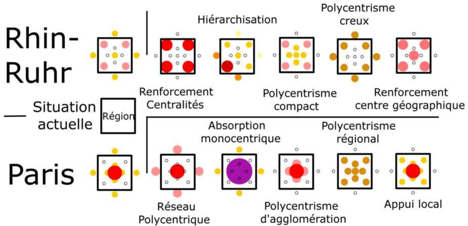
FIG. 6.18 – Scénarios d'évolution des régions Rhin-Ruhr (haut) et Ile-de-France (bas). Du blanc au violet : population du pôle.
