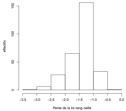
histogramme pour le pas de grille : 6,4 km
