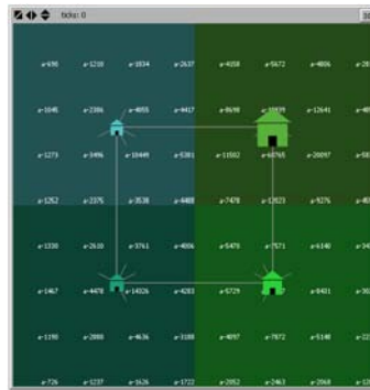
FIG. 6.20 – Description de la ville virtuelle : une métropole polycentrique
