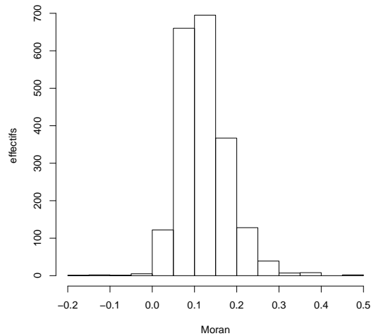
Histogramme : indice de Moran
