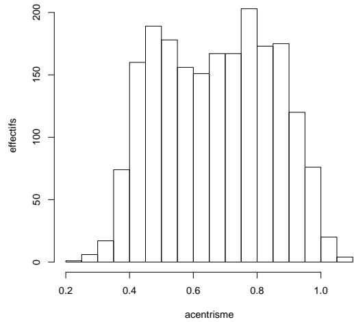
Histogramme : acentrisme
