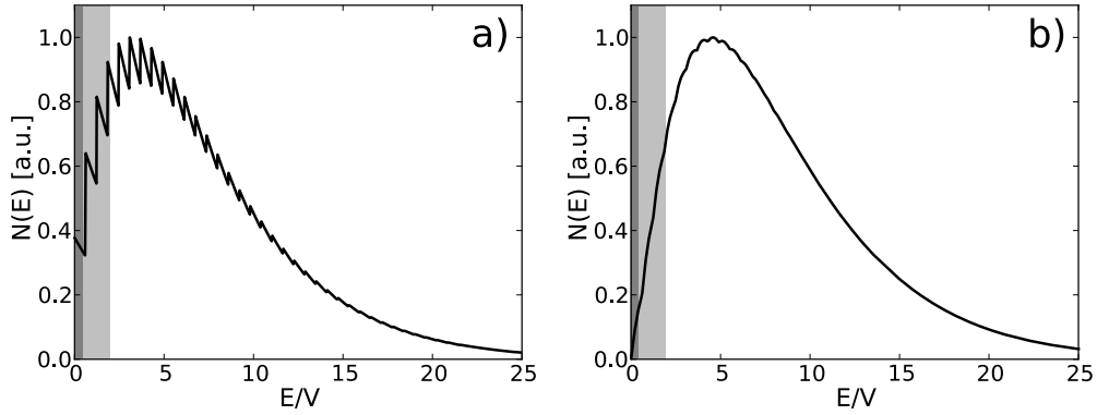
FIGURE 7.13 – Distribution d'énergie du nuage thermalisé. a) Nuage à 200 nK dans le piège 2D avant d'allumer le désordre. b) Nuage à 205 nK en présence du désordre de profondeur 53 nK. Les régions grisées correspondent à des régimes d'expansion subdiffusive (gris clair) et piégé à temps long sous le seuil de percolation (gris foncé).
