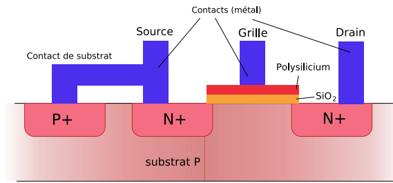
FIGURE 5.1 – Représentation schématique d'un MOSFET. Le transistor est constitué de deux électrodes reliées par une interface entre un semi-conducteur et une couche d'oxyde isolante. En présence d'un champ électrique appliqué via la grille de polysilicium, des porteurs de charge s'accumulent à cette interface, confinés en deux dimensions. La valeur du champ électrique permet de contrôler leur densité. Source : Wikipedia commons.
