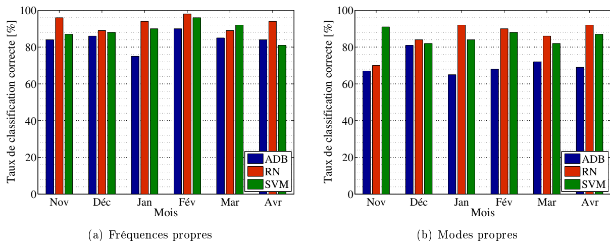
FIGURE 6.48 – Méthodes de classification supervisée appliquées aux paramètres modaux transformés en histogrammes (filtre linéaire ; analyse mois par mois ; 30% entr., 10% val., 60% test ; valeurs en %).
