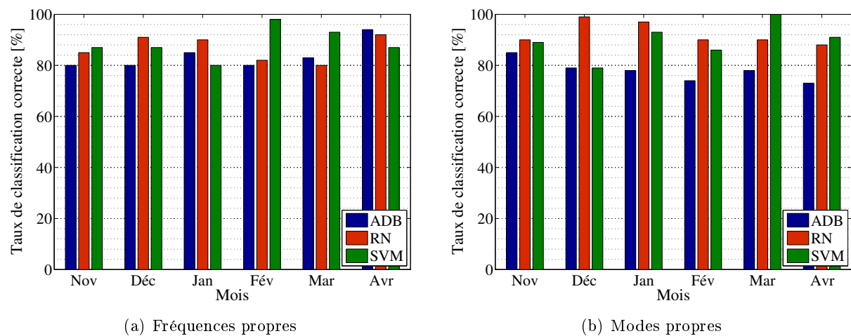
FIGURE C.29 – Méthodes de classification supervisée appliquées aux paramètres modaux transformés en intervalles (filtre linéaire ; analyse mois par mois ; 50% entr., 10% val., 40% test ; valeurs en %).
