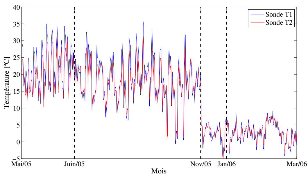
FIGURE 5.41 – Variation des températures au cours du temps pour les sondes T1 et T2.
