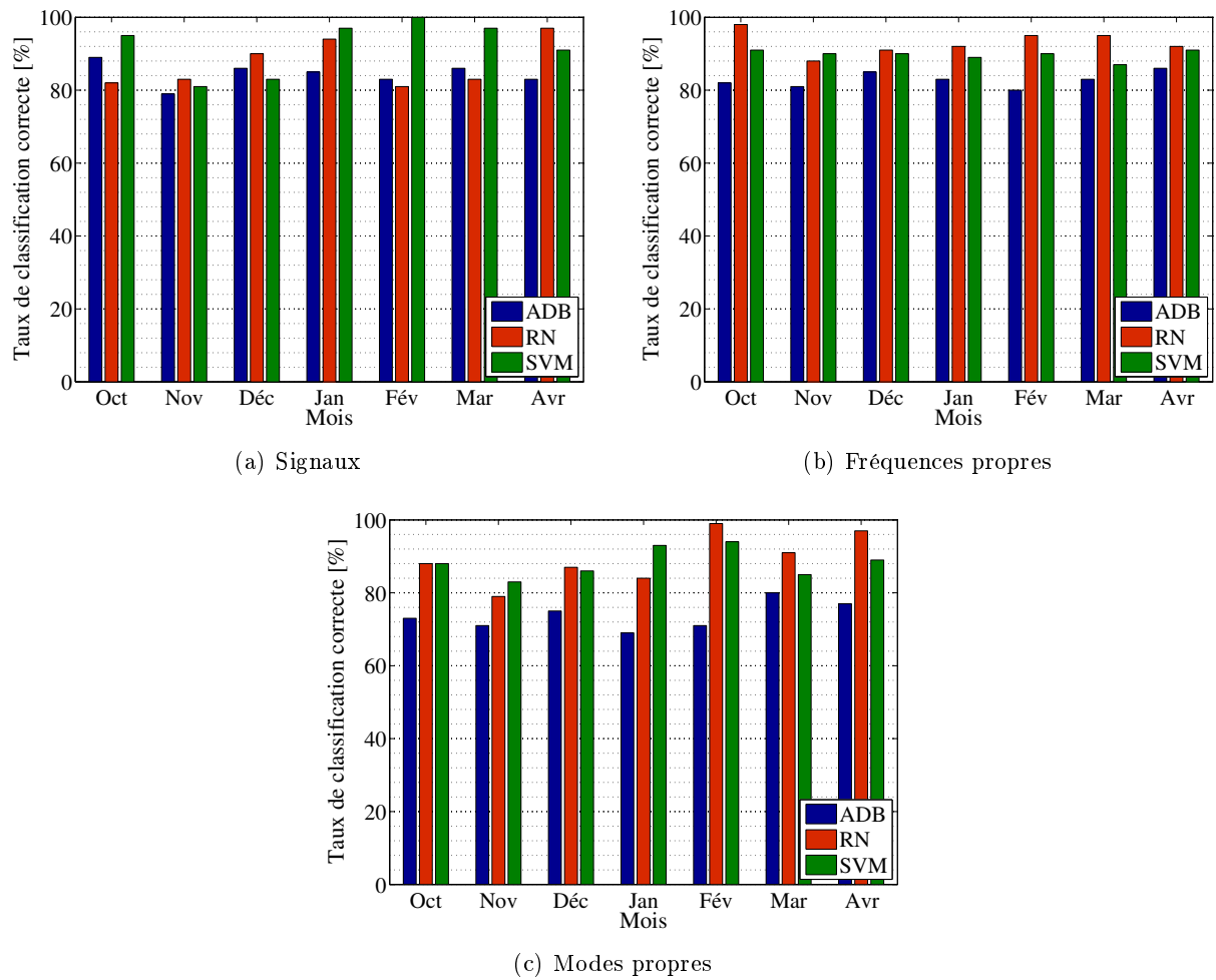
FIGURE C.18 – Méthodes de classification supervisée appliquées aux signaux et paramètres modaux transformés en histogrammes (analyse mois par mois ; 40% entr., 10% val., 50% test ; valeurs en %).
