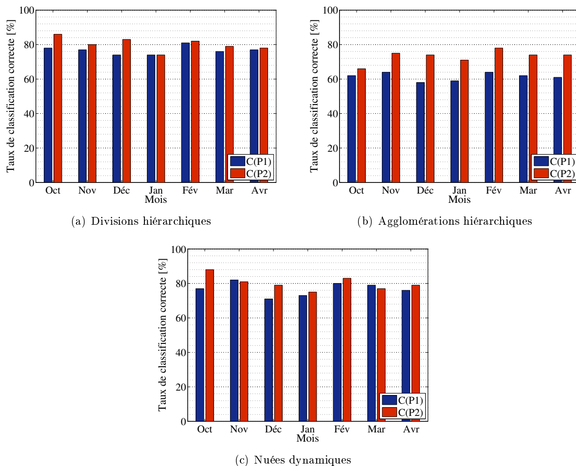
FIGURE 6.37 – Méthodes de partitionnement appliquées aux modes propres transformés en histogrammes.
