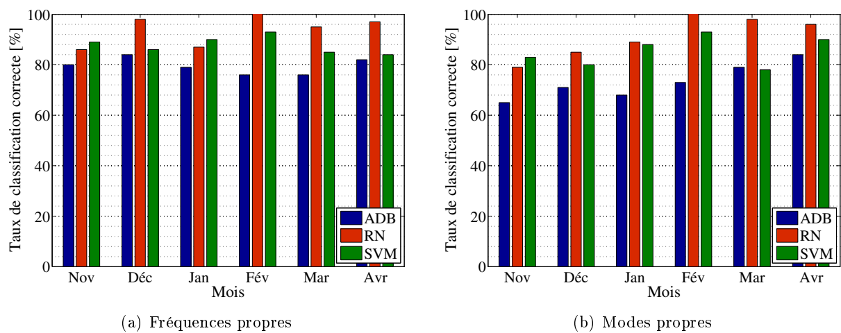
FIGURE C.23 – Méthodes de classification supervisée appliquées aux paramètres modaux transformés en histogrammes (filtre linéaire ; analyse mois par mois ; 40% entr., 10% val., 50% test ; valeurs en %).
