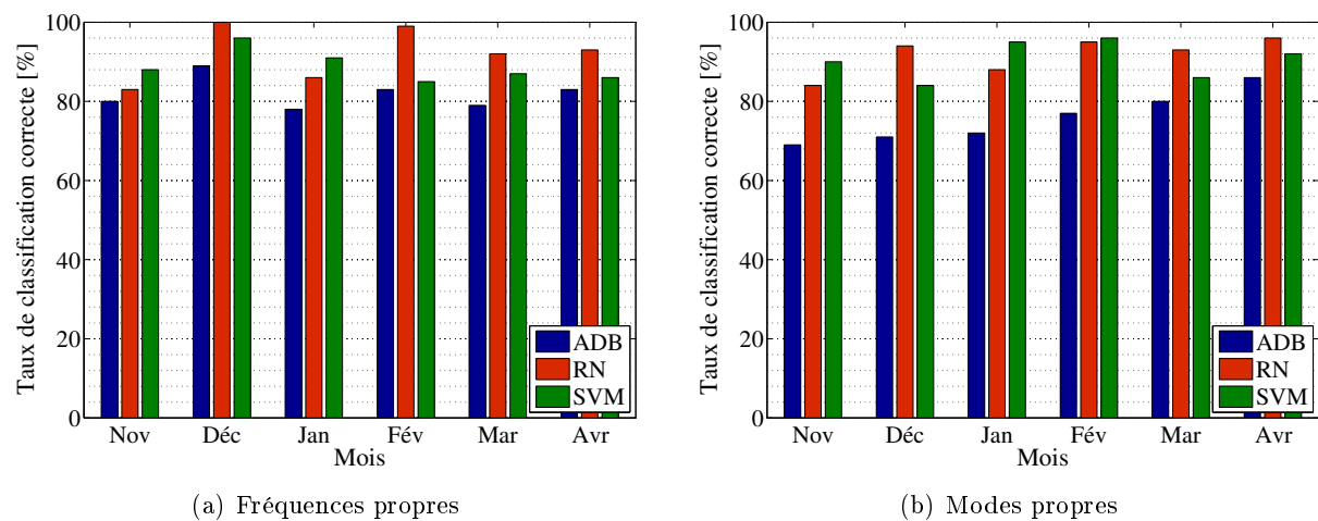
FIGURE C.25 – Méthodes de classification supervisée appliquées aux paramètres modaux transformés en histogrammes (filtre non linéaire ; analyse mois par mois ; 40% entr., 10% val., 50% test ; valeurs en %).
