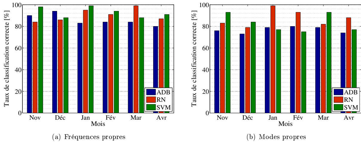
FIGURE C.30 – Méthodes de classification supervisée appliquées aux paramètres modaux transformés en intervalles (filtre non linéaire ; analyse mois par mois ; 30% entr., 10% val., 60% test ; valeurs en %).
