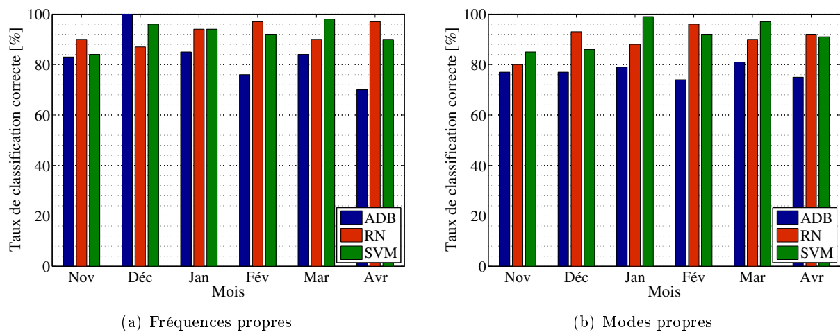
FIGURE C.31 – Méthodes de classification supervisée appliquées aux paramètres modaux transformés en intervalles (filtre non linéaire ; analyse mois par mois ; 40% entr., 10% val., 50% test ; valeurs en %).
