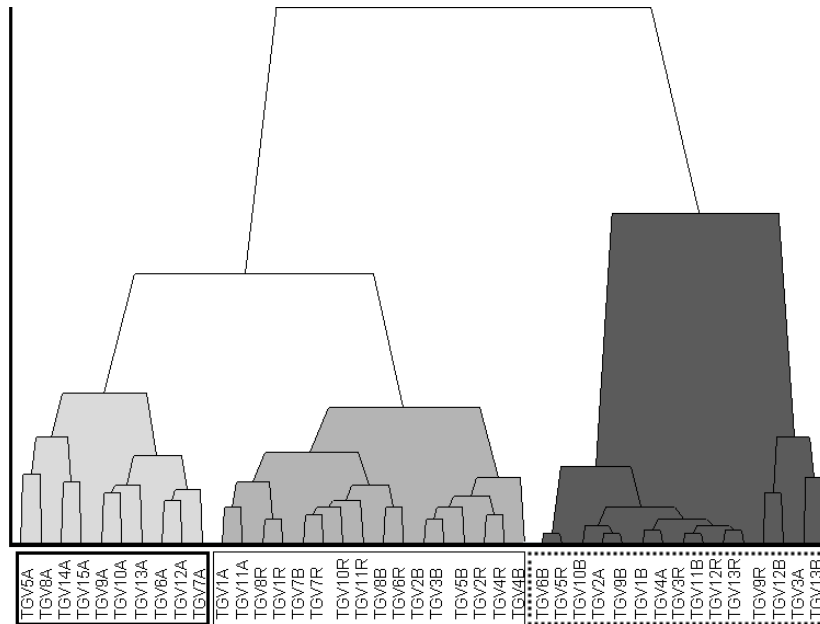
FIGURE 5.15 – Classification des signaux en utilisant les agglomérations hiérarchiques (histogrammes).
