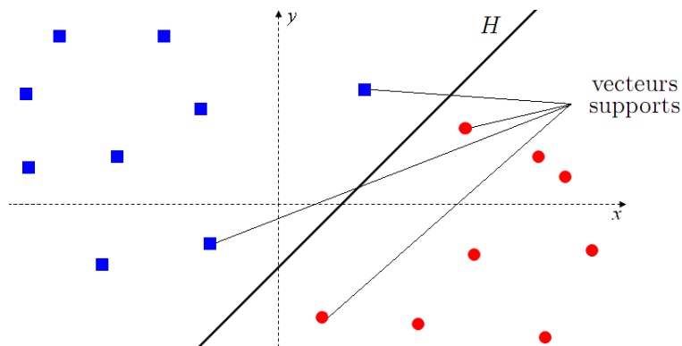
FIGURE 3.10 – Séparation de deux classes de données par un hyperplan H .
