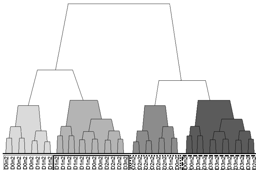
FIGURE A.17 – Classification des modes propres avec bruit (n2) utilisant les agglomérations hiérarchiques (intervalles).
