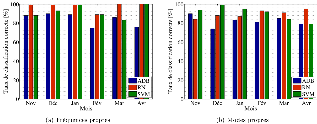
FIGURE C.26 – Méthodes de classification supervisée appliquées aux paramètres modaux transformés en histogrammes (filtre non linéaire ; analyse mois par mois ; 50% entr., 10% val., 40% test ; valeurs en %).
