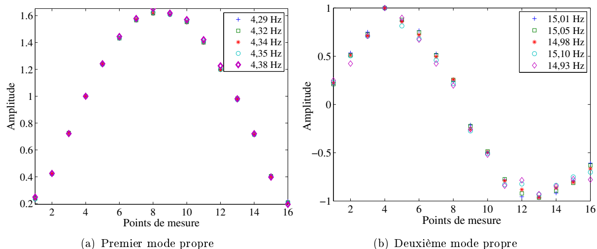
FIGURE 2.3 – Fréquences et modes propres identifiés pour 5 réalisations d'une identification modale.
