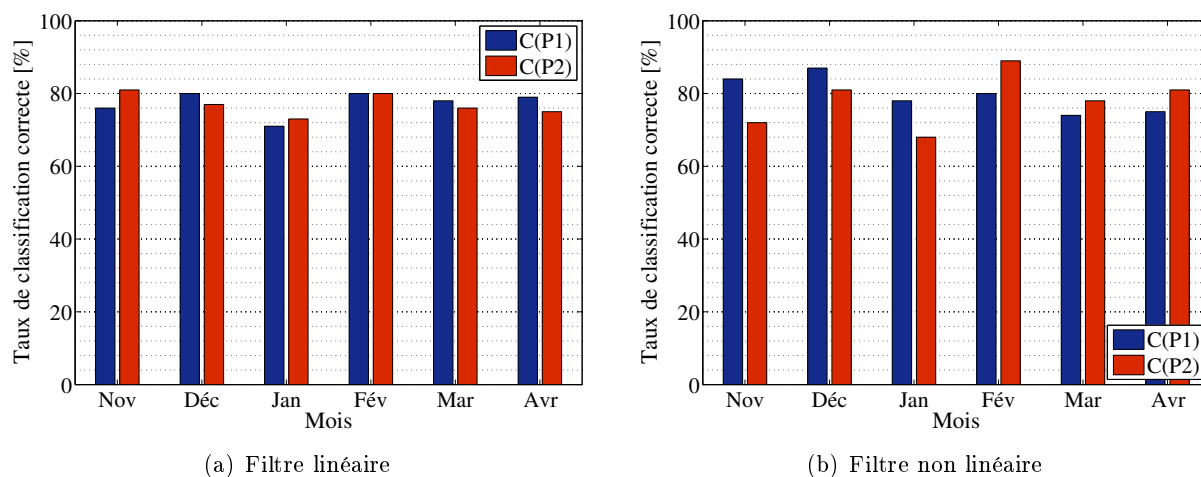
FIGURE 6.38 – Méthode des divisions hiérarchiques appliquées aux modes propres « corrigés » (filtre linéaire et non linéaire)
