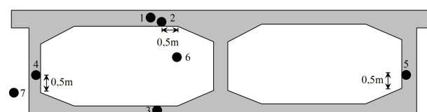
(b) Plan d'instrumentation des sondes de température
