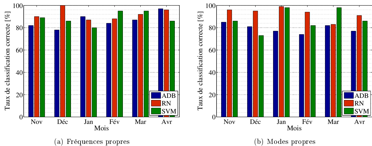
FIGURE C.32 – Méthodes de classification supervisée appliquées aux paramètres modaux transformés en intervalles (filtre non linéaire ; analyse mois par mois ; 50% entr., 10% val., 40% test ; valeurs en %).
