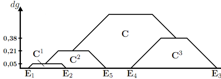
FIGURE 3.2 – Exemple d'une agglomération hiérarchique avec 3 clusters.
