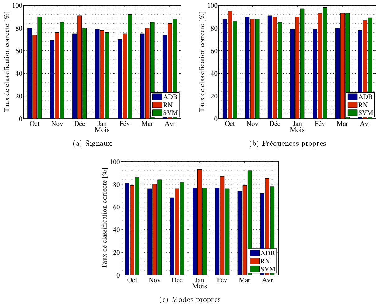
FIGURE C.20 – Méthodes de classification supervisée appliquées aux signaux et paramètres modaux transformés en intervalles (analyse mois par mois ; 30% entr., 10% val., 60% test ; valeurs en %).
