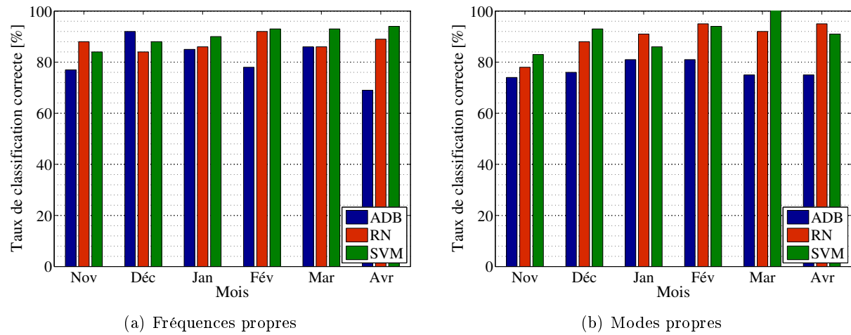
FIGURE C.28 – Méthodes de classification supervisée appliquées aux paramètres modaux transformés en intervalles (filtre linéaire ; analyse mois par mois ; 40% entr., 10% val., 50% test ; valeurs en %).
