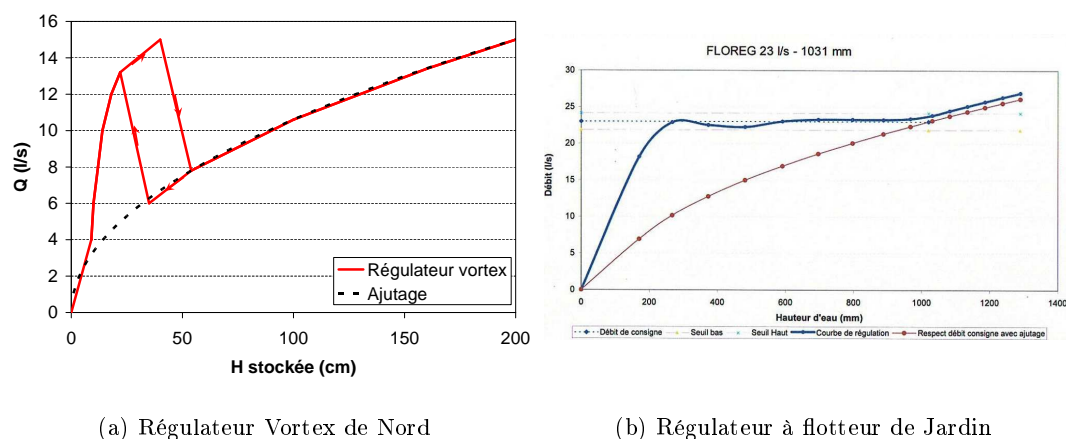
FIG. 19.6: Courbes de régulation des régulateurs commerciaux et comparaison avec un ajustage (dimensionné pour avoir le même Q_{\max} )
