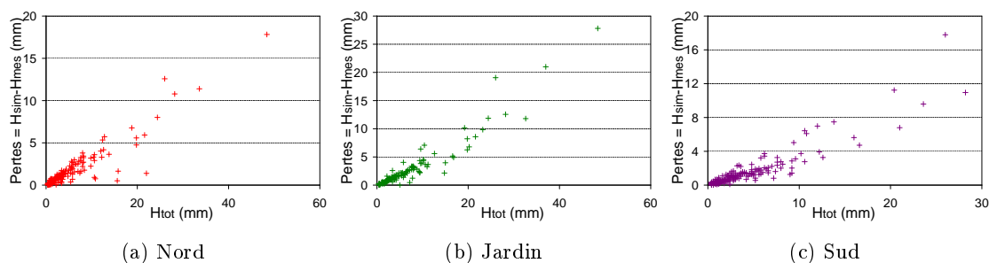
FIG. 19.5: Pertes estimées entre les simulations sans techniques alternatives et les mesures, en fonction de la hauteur d'eau précipitée
