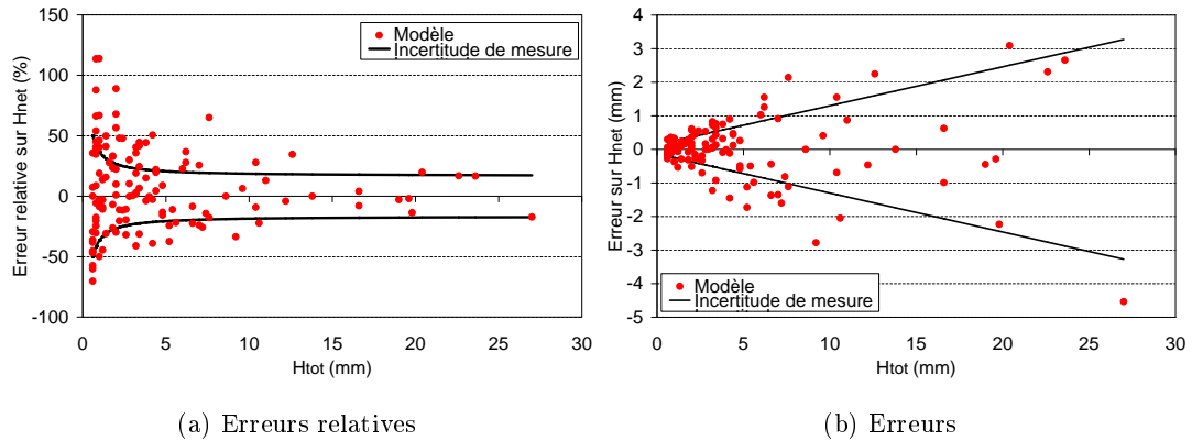
FIG. 17.6: Erreurs et erreurs relatives sur la hauteur ruisselée en fonction de la hauteur précipitée, et intervalle de confiance des erreurs (déduit des incertitudes de mesure)
