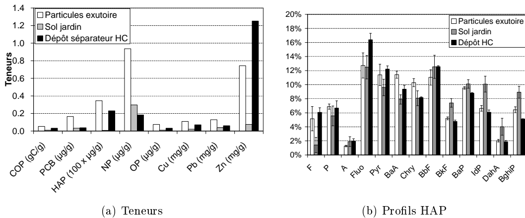
FIG. 21.5: Comparaison des teneurs et des profils HAP dans les différents types de particules sur Jardin
