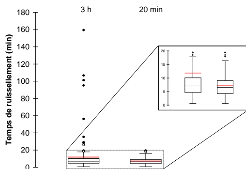
FIG. 10.8: Temps de réaction sur Référence suivant qu'on cherche le début de la pluie 3 h ou 20 min avant le début du débit
