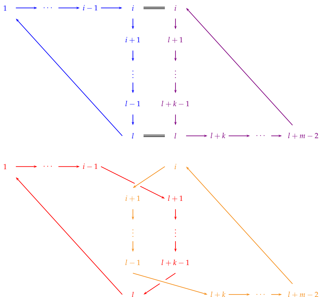
FIGURE 10.5 – Le produit de deux cycles C_l (en bleu) et C_m (en violet) s'intersectant en deux points d'écart (i, l - i) dans C_l et (k, m - k) dans C_m est égal au produit de deux cycles disjoints de longueurs respectives i + k - 1 (en rouge) et (l - i) + (m - k) - 1 (en orange).
