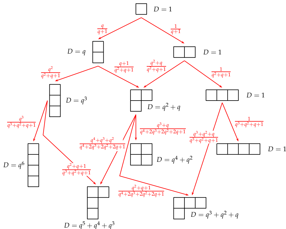
FIGURE 7.1 – Degrés génériques et q -probabilités de transition sur les quatre premiers niveaux du graphe de Young.
