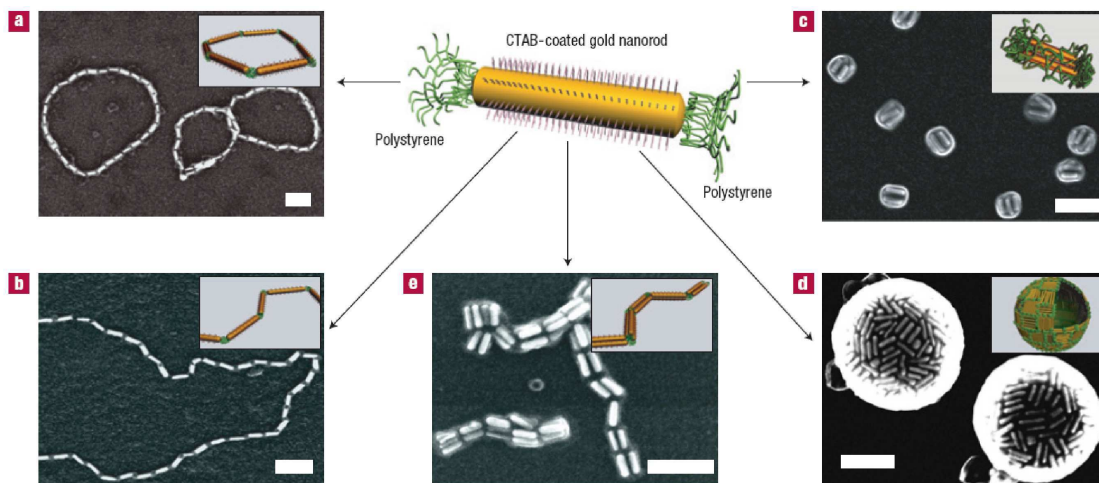
FIGURE 1.4 – Auto-assemblage de nanobâtonnets d'or fonctionnalisées par du polymère en solvant sélectif : (a) anneaux, (b) chaînes (DMF/H 2 O à 6 et 20 % en eau), (c) paquets de bâtonnets, (d) nanosphères (THF/H 2 O à 6 et 20 % en eau), (e) paquets de bâtonnets en chaînes (DMF/THF/H 2 O à 42,5 :42,5 :15) [36].
