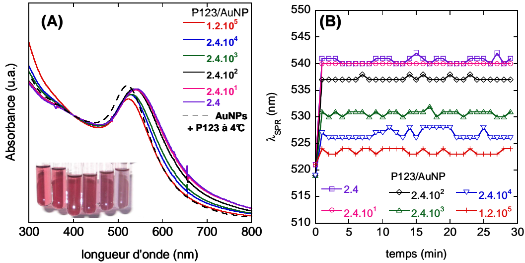
FIGURE 4.10 – (A) Spectres d’absorbance UV-visible (normalisés à 400 nm) des AuNP@100/0 dans une solution de KCl à 10 mM ( T_{agg} = 12\text{ °C} ) avec différentes concentrations en P123 après 30 min à 40 °C. Photo des solutions de AuNP@100/0 correspondantes avec 5, 1, 10^{-1} , 10^{-2} , 10^{-3} , 10^{-4} % en masse de P123 de gauche à droite. (B) Cinétique en UV-visible à 40 °C des mêmes solutions. Les valeurs de \lambda_{SPR} ont été enregistrées toutes les minutes pendant 30 min. À t = 0 , la solution refroidie dans un bain de glace est directement introduite dans une cuve UV thermostatée à 40 °C.
