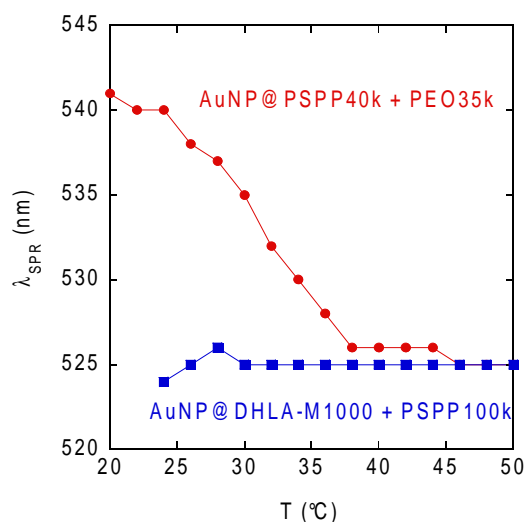
FIGURE 5.22 – Évolution de la longueur d'onde maximale \lambda_{SPR} en fonction de la température des AuNP@PSPP70k dans une solution aqueuse de PEO35k à 1 % en masse et des AuNP17@DHLA-M1000 dans une solution de 1 % en masse de PSPP100k (par pas de 2 °C toutes les 6 min),
