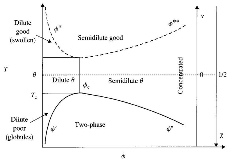
FIGURE 5.25 – Diagramme de phase de solutions de polymère avec une UCST. La séparation de phase a lieu en dessous de la courbe en trait plein. La courbe en pointillé est la frontière en température du régime dilué en bon solvant au régime semi-dilué. D’après Rubinstein et al. [89].
