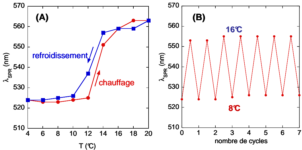
FIGURE 2.13 – (A) Évolution du maximum de la bande de résonance plasmon de surface \lambda_{SPR} en fonction de la température pour les AuNP6@DHLA-M600 dans une solution de KCl à 10 mM pour un cycle complet de chauffage/refroidissement (par pas de 2 °C toutes les 5 min), (B) Variation de \lambda_{SPR} pour plusieurs cycles de chauffage/refroidissement du même échantillon (par pas de 8 °C toutes les 15 min).
