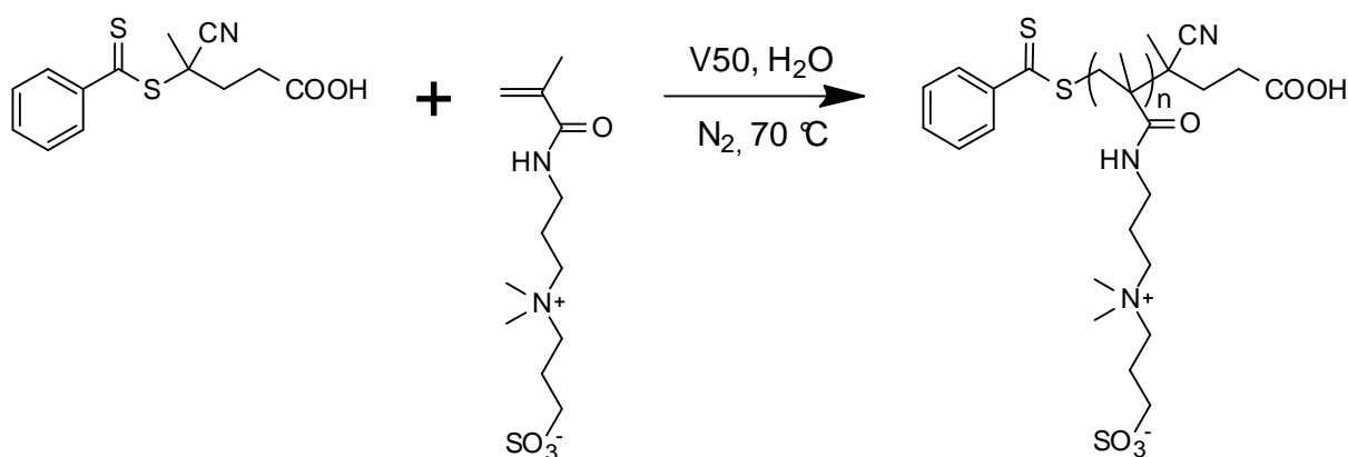
FIGURE 5.4 – Représentation schématique de la stratégie de synthèse des polymères P(SPP).
