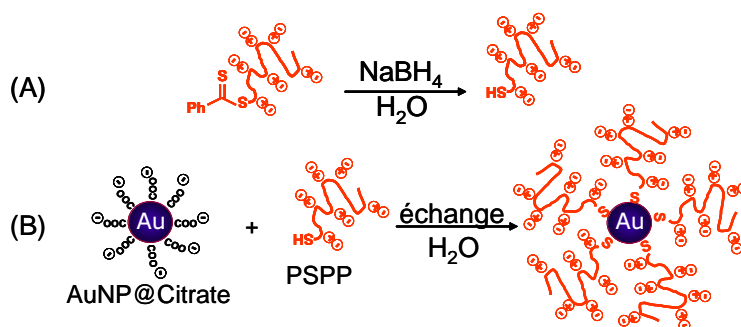
FIGURE 5.8 – Voie de synthèse des AuNPs hybrides.
