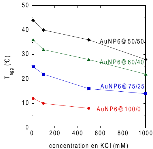
FIGURE 2.23 – Évolution de la température d'agrégation T_{agg} en fonction de la concentration en KCl pour les différentes AuNP6@x/y.
