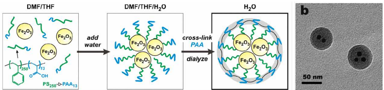
FIGURE 1.3 – Représentation et imagerie MET de l'encapsulation de nanoparticules Fe 2 O 3 dans des micelles de PS-PAA [28].
