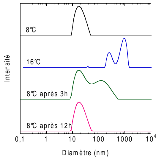
FIGURE 2.14 – Distributions de taille (déterminées en DLS) des AuNP6@DHLA-M600 dans une solution de KCl à 10 mM sur un cycle de chauffage/refroidissement.
