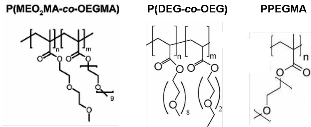
FIGURE 1.13 – Structure chimique des polymères synthétisés par Lutz et al. [69] (2-(2-méthoxyéthoxy)éthyl méthacrylate-oligo(éthylène glycol) méthacrylate), Boyer et al. [70] (di(éthylène glycol) méthyl éther méthacrylate-oligoéthylène glycol méthacrylate) et Gibson et al. [72] (poly(poly(éthylène glycol)mono-méthyléther)méthacrylate)).
