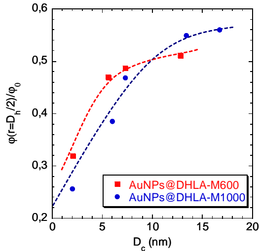
FIGURE 2.21 – Concentration en polymère calculée à la surface externe \varphi(r) ( r = D_h/2 ) rapportée à la concentration en polymère à la surface du coeur \varphi_0 en fonction du diamètre de coeur D_c .
