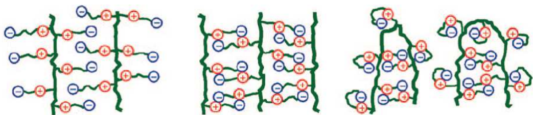
FIGURE 5.1 – Différents états de conformation de polyzwitterions : de chaînes non-associées totalement hydratées (à gauche), à des chaînes effondrées avec associations inter-chaînes (au milieu) et intra-chaînes (à droite). D'après Cheng et al. [73].
