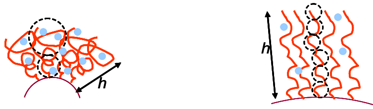
FIGURE 2.19 – Représentation schématique des différentes conformations du polymère à la surface de la particule. Les ronds bleus schématisent les molécules d'eau.
