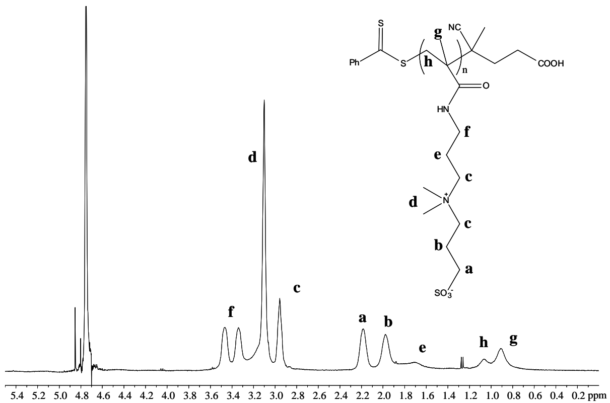
FIGURE C.4 – Spectres RMN ^1\text{H} du PSCP100k dans \text{D}_2\text{O} .
