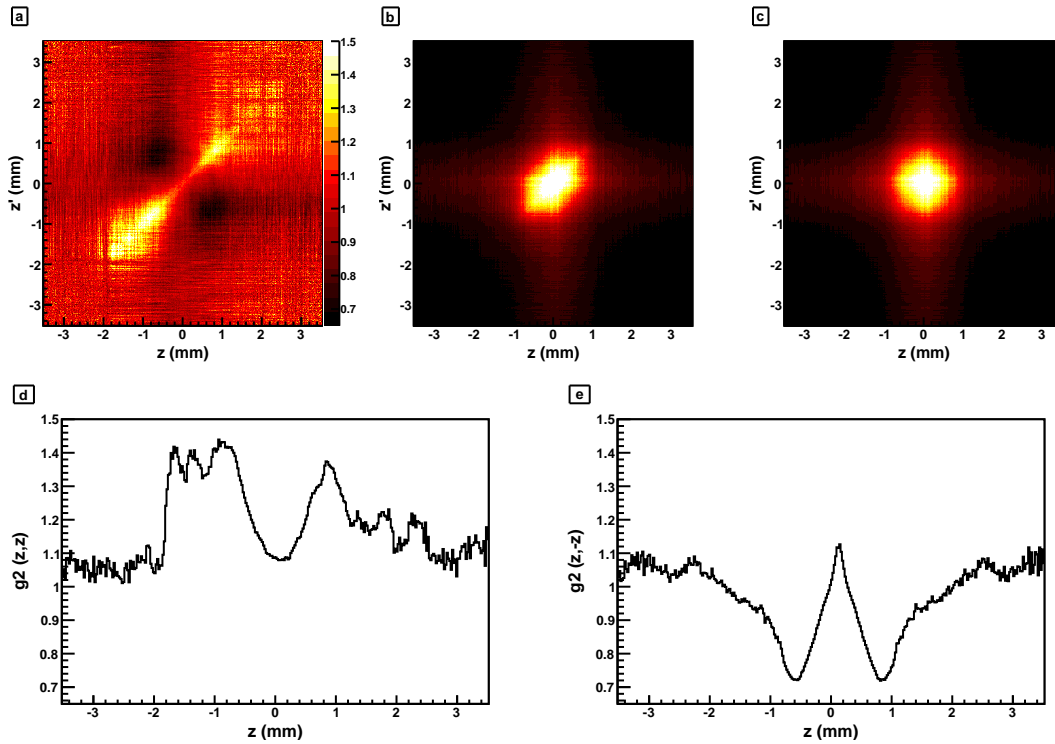
FIGURE 2.14 La fonction de corrélation du second ordre g^{(2)}(z, z') (a) pour un condensat après temps de vol de 307 ms est obtenue en normalisant la fonction de corrélation brute G^{(2)}(z, z') (b) par le produit des densités \langle n(z) \rangle \langle n(z') \rangle (c). Si l'on ne corrige pas les fluctuations du temps d'arrivée, g^{(2)} est maximal sur les flancs du condensat pour z' = z (coupe d), et minimal, sur les flancs également, pour z' = -z (coupe e).
