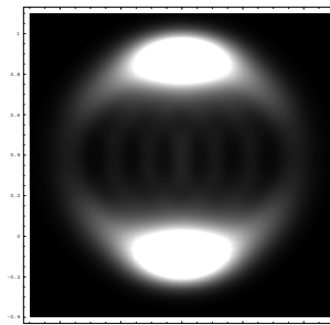
FIGURE 4.17 Coupe 2D de la distribution en impulsion des atomes, en supposant que la population de chaque mode est proportionnelle au carré du recouvrement, pour une profondeur du réseau de 0.9 E_{rec} et k_0 = 0,6k_{rec} . On sous-estime alors la population des pics en k_1 et k_2 , et celles des premiers états excités, proches de ces pics.
