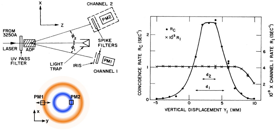
FIGURE 1.6 Mesure des corrélations en vecteur d'onde par Burnham et Weinberg. Le taux de coïncidence R_c entre les photomultiplicateurs PM1 et PM2 - équipés respectivement de filtres fréquentiels centrés en \nu_1 (orange) et \nu_2 (bleu) - est tracé en fonction de la position de PM1 ( PM2 ne bougeant pas). La largeur de la corrélation mesurée vient des résolutions d_1 et d_2 des 2 détecteurs, et est faible devant la largeur de la distribution en intensité (taux de détection R_1 de PM1 , également représenté). Extrait de [Burnham 70].
