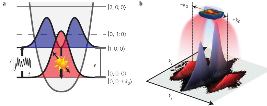
FIGURE 1.17 Les atomes préparés dans le premier état excité transverse (en bleu) ne peuvent se désexciter que par paires, dans les modes longitudinaux (en rouge). Figure extraite de [Bücker 11].
