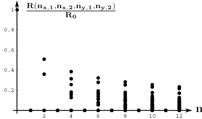
FIGURE 4.16 Recouvrement des fonctions d'ondes transverses R(n_{x,1}, n_{x,2}, n_{y,1}, n_{y,2}) = \int dx \phi_0(x)^2 \phi_{n_{x,1}}(x) \phi_{n_{x,2}}(x) \int dy \phi_0(y)^2 \phi_{n_{y,1}}(y) \phi_{n_{y,2}}(y) pour tous les modes (n_{1x}, n_{1y}, n_{2x}, n_{2y}) , en fonction du nombre total d'excitation n = n_{1x} + n_{1y} + n_{2x} + n_{2y} . Le recouvrement est ici normalisé par R_0 = \int dx \phi_0(x)^4 \int dy \phi_0(y)^4 , qui correspond au cas du mélange à quatre ondes unidimensionnel.
