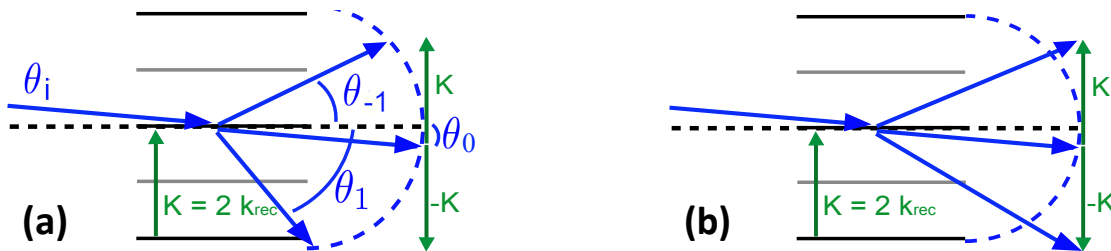
FIGURE 3.6 (a) Dans le régime de Raman-Nath, le vecteur d'onde du réseau est mal défini, en raison de la faible épaisseur du réseau. La diffraction a alors lieu dans plusieurs directions, déterminées par la loi des réseaux 3.21. (b) Dans le régime de Kapitza-Dirac, la diffraction est suffisamment rapide pour que l'énergie ne soit pas strictement conservée. Les atomes d'impulsion initiale \hbar q sont alors diffractés vers les états d'impulsion \hbar(q + mK) , m \in \mathbb{N}
