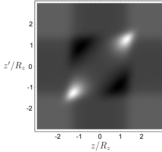
FIGURE 2.15 Fonction de corrélation du 2e ordre obtenue en simulant une distribution de Thomas-Fermi dont le centre fluctue de 0,1R_z , sans introduire de corrélation quantique.
