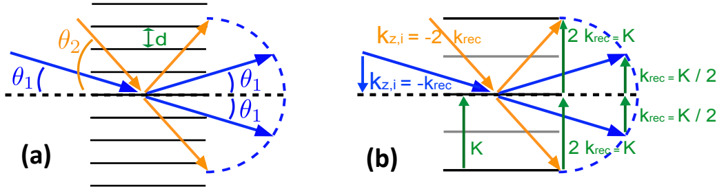
FIGURE 3.4 (a) La diffraction de Bragg d'un faisceau de vecteur d'onde k_{z,i} par un réseau de pas d et de vecteur réciproque K = 2\pi/d n'a lieu que pour des angles incidents \theta_n qui vérifient la loi de Bragg, qui peut se traduire par la conservation de l'impulsion (transfert de K ) et de l'énergie (conservation de la norme). (b) Pour un faisceau d'atomes, ce processus correspond à l'absorption puis à la réémission de n photons, soit un transfert d'impulsion \hbar k_{rec} pour chaque photon absorbé ou réémis.
