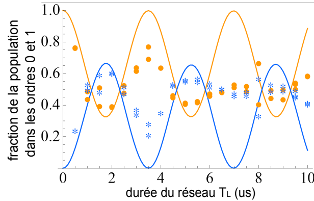
FIGURE 3.11 Fraction des atomes détectés à 0v_{rec} (ronds oranges) et \pm 2v_{rec} (* bleus) après application du réseau pendant une durée T_L à une puissance de 240mW, sur un quasi-condensat initialement au repos, et comparaison avec les fractions calculées dans le régime de Kapitza-Dirac (courbe orange pour 0v_{rec} et bleue pour \pm 2v_{rec} ) pour une profondeur du réseau de 7,7E_{rec} . La saturation du nombre d'atomes détectés pour les pics très peuplés tend à réduire l'amplitude de ces oscillations. Par ailleurs, celles-ci sont amorties dès la deuxième période. La précision de l'estimation de V_0 par cette méthode est de \pm 0,5E_{rec} .
