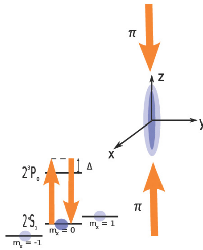
FIGURE 1.11 Déclenchement de la collision - On a préalablement appliqué un pulse radio-fréquence pour transférer la moitié des atomes de m = 1 vers m = 0 . Le reste des atomes est en m = \pm 1 (en bleu ciel), formant des condensats superposés spatialement à celui en m = 0 (en bleu foncé). Ce dernier est ensuite séparé en 3 : avec 2 faisceaux contrapropageants désaccordés de \Delta = 600\text{MHz} sur le bleu de la transition 2^3s_1 - 2^3p , on réalise un quart d'oscillation de Rabi de la classe d'impulsion nulle vers celles d'impulsion \pm 2\hbar k_{rec} (absorption d'un photon d'un des faisceaux et réémission selon l'autre faisceau). Les faisceaux sont polarisés \pi et n'adressent donc que les atomes en m = 0 . Les collisions interatomiques ont lieu au moment de la séparation des 3 condensats d'impulsions 0 et \pm 2\hbar k_{rec} .
