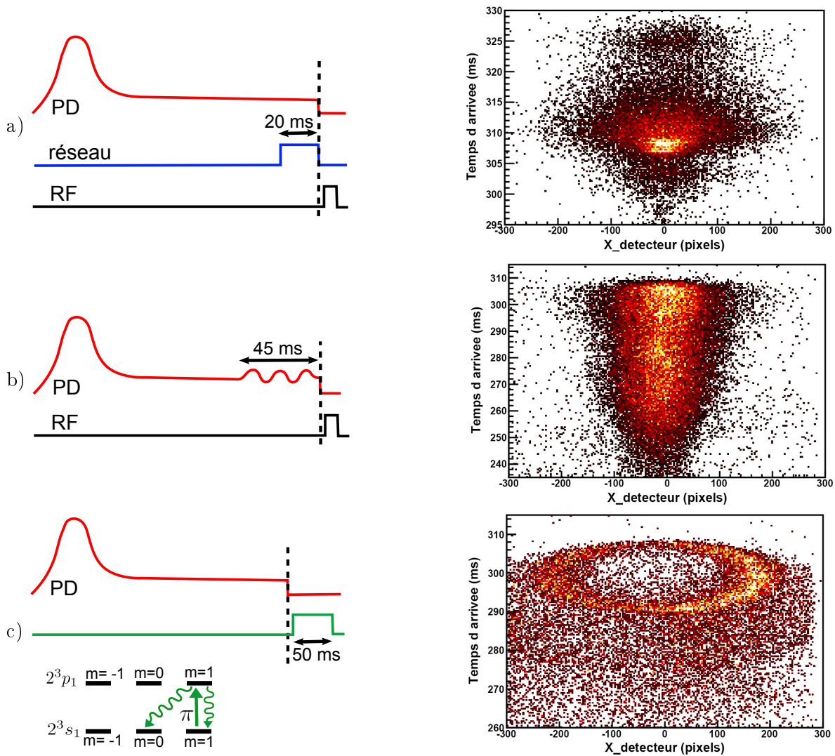
FIGURE 2.8 Pour mesurer le nombre d'atomes du condensat, nous éclatons celui-ci pour diminuer la densité atomique, de sorte qu'il n'y ait pas de saturation du signal détecté. Nous avons testé 3 méthodes différentes, pour lesquelles je représente la séquence temporelle (à gauche), et une coupe dans le plan (x,z) du signal détecté après temps de vol (à droite), intégrée sur 200 pixels (environ 3cm) selon y (Les axes sont pris dans le référentiel du détecteur). a) Le réseau optique est allumé à la fin du piège dipolaire (PD) pour chauffer les atomes. À la coupure du PD, une rampe radio-fréquence (RF) transfère une partie des atomes de m = 1 vers m = 0 , et l'on applique un fort gradient magnétique pour éjecter les atomes en m = \pm 1 et ne détecter que les m = 0 . On observe une distribution thermique autour du temps d'arrivée normal du BEC (307ms), et autour du pic de diffraction à 326ms, favorisé par la vitesse du réseau dans le référentiel du laboratoire (§3.3). b) Le piège dipolaire est modulé après la fin de l'évaporation, avec une amplitude suffisante pour faire continuellement tomber du piège une partie des atomes. Comme en (a), on ne détecte que les atomes transférés en m = 0 par RF. c) Les atomes sont excités par un faisceau polarisé \pi proche de résonance, allumé après la coupure du PD. On détecte la sphère d'émission spontanée vers m=0 (en haut de l'image), et les atomes qui sont transférés en m=0 après plusieurs cycles d'absorption-émission spontanée (atomes sous la sphère). Comme la transition 2^3s_1, m=0 - 2^3p_1, m'=0 est interdite, les atomes ne subissent plus de transfert d'impulsion un fois dans m=0 .
