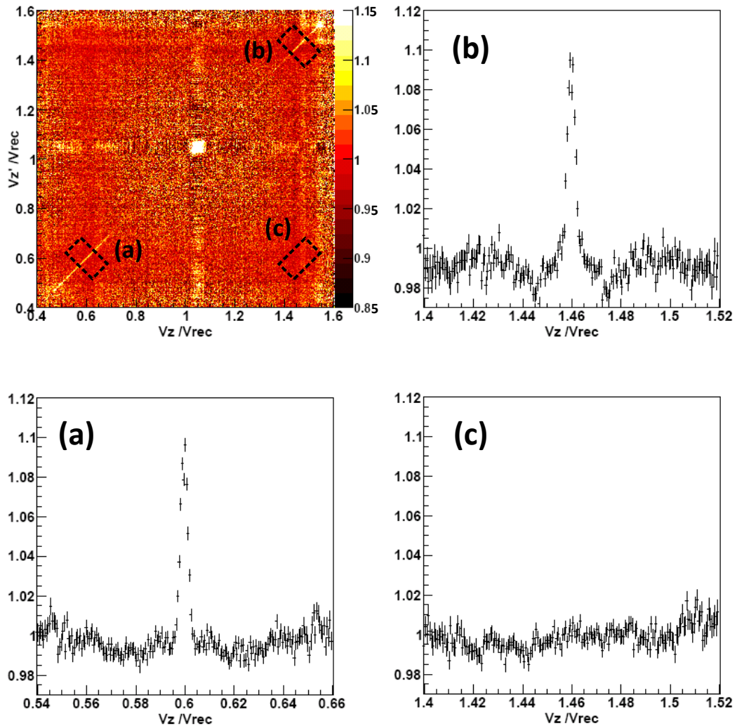
FIGURE 4.22 Carte de g^{(2)}(v_z, v'_z) après recentrage et sélection des données, restreinte aux deux pics formés par les paires en v_1 \sim 0,6v_{rec} et v_2 \sim 1,45v_{rec} . Les motifs présents sur la carte sans recentrage de la figure 4.18 ont presque totalement disparu. On distingue sur la diagonale un maximum de g^{(2)} au niveau de chacun des deux pics, mais aucune corrélation croisée entre ces pics ne sort du bruit sur la carte. La singularité à mi-distance des pics (à 1,05v_{rec} ) est due à notre procédure de recentrage séparé des atomes autour des deux pics. Les rectangles en pointillés sur la carte indiquent les limites des zones d'intégrations des coupes (a), (b) et (c) (la coupe est toujours intégrée selon le petit côté du rectangle). (a) Coupe de la corrélation locale en v_1 , en fonction de l'axe horizontal v_z . Autour du pic principal - ride sur la diagonale déjà visible sur la carte -, on distingue des pics latéraux. (b) Coupe de la corrélation locale en v_2 , en fonction de l'axe horizontal v_z . (c) Coupe selon la direction ( v'_z = v_z + \text{constante} ), on ne distingue pas le signal de corrélation croisé attendu au centre de la fenêtre.
