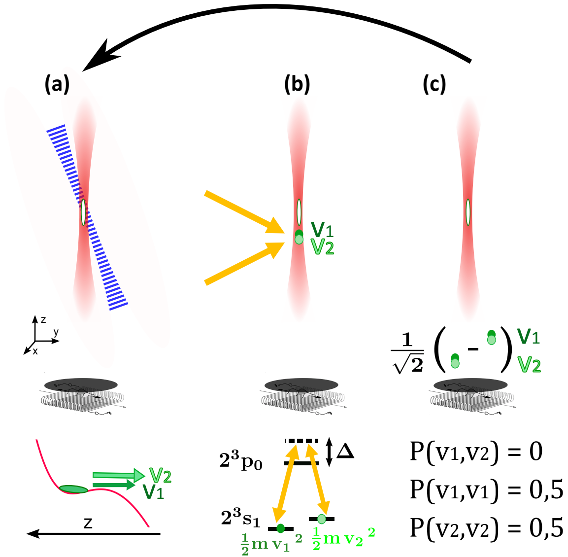
FIGURE 4.24 Schéma proposé pour mesurer l'effet Hong-Ou-Mandel atomique sur notre montage expérimental en un temps raisonnable. (a) Application du réseau optique pendant un temps très court, pour ne créer en moyenne que moins d'une paire d'atomes de vitesses v_1 et v_2 . (b) Pulse \pi/2 entre les vitesses v_1 et v_2 , équivalent d'une lame séparatrice 50/50. (c) Détection des atomes. Cette séquence peut être reproduite plusieurs fois au cours d'un cycle expérimental.
