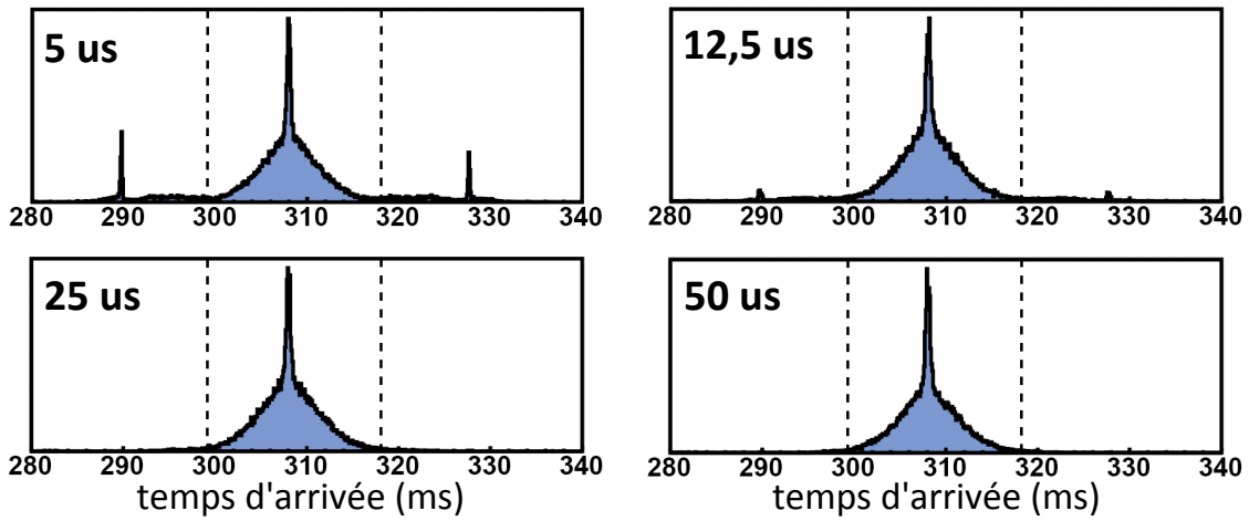
FIGURE 3.14 Pour déterminer quelle doit être la durée minimale d'une rampe du réseau pour que l'évolution du potentiel vue par les atomes soit adiabatique, nous avons appliqué aux atomes des rampes en forme de triangle dont nous faisons varier le temps de montée \tau (égal à celui de descente) de 5 à 50\mu\text{s} . Si la rampe est adiabatique, le signal détecté après temps de vol ne devrait pas présenter de pic de diffraction. Les lignes verticales pointillées indiquent la limite de la première zone de Brillouin.
