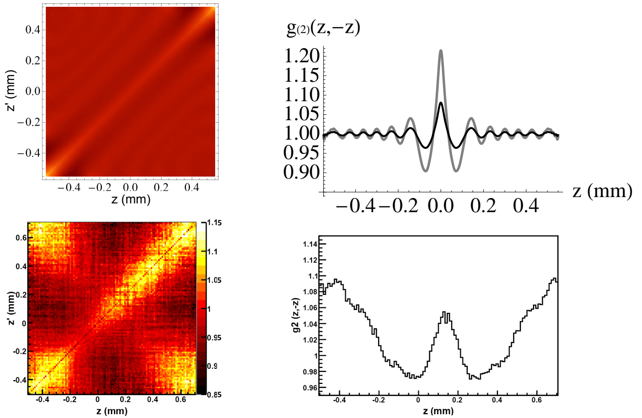
FIGURE 2.17 En haut : fonction de corrélation g^{(2)}(z, z') calculée à partir de l'expression (2.26) pour des températures de 200nK (image 2D et courbe grise sur la coupe z' = -z ) et de 75nK (courbe noire sur la coupe). En bas : fonction de corrélation et coupe z' = -z à partir des données expérimentales.
