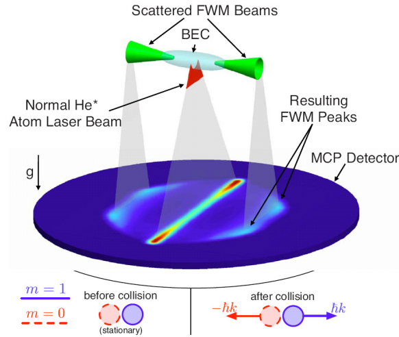
FIGURE 1.19 Paires de faisceaux jumeaux générés par mélange à quatre ondes spontané à Canberra. Figure extraite de [Dall 09].
