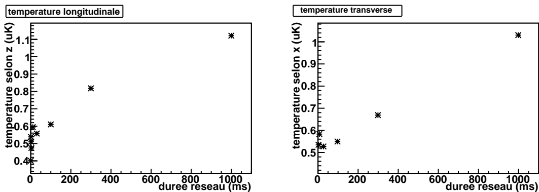
FIGURE 3.16 Pour différentes durée du réseau, monté et descendu en 500 \mu s , on mesure sur le temps de vol la largeur en vitesse sur chaque axe, dont on déduit la température.
