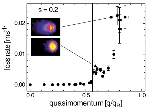
FIGURE 4.1 Taux de pertes d'un condensat dans un réseau optique en fonction de sa quasi-impulsion q . L'augmentation des pertes coïncide avec le seuil attendu de l'instabilité dynamique (ligne verticale). Quand celle-ci est très importante, la distribution de densité présente des structures complexes, traduisant la perte de cohérence. Figure extraite de [Fallani 04].
