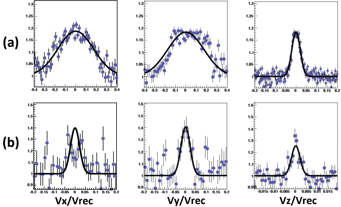
FIGURE 1.13 Coupes des fonctions de corrélation opposée g_{opp}^{(2)}(\vec{r}) (a) et locale g_{loc}^{(2)}(\vec{r}) (b) selon les 3 axes de l'expérience.
