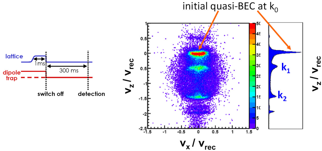
FIGURE 4.8 Séquence expérimentale pour la création de paires, et signal détecté après le temps de vol : coupe selon v_x et v_z , et selon v_z . Le pic le plus intense correspond au condensat initial, et 2 autres pics émergent. Ceux-ci sont relativement fins, mais on détecte des atomes entre eux, repartis sur un halo sphérique. Le petit pic à -2v_{rec} est dû à la diffraction.
