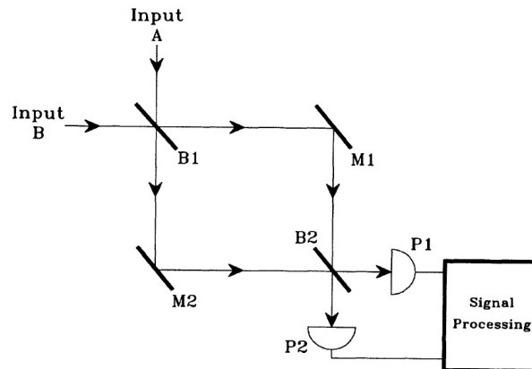
FIGURE 1.10 Dans le schéma proposé par M.Holland et K.Burnett, 2 faisceaux jumeaux générés par conversion paramétrique sont injectés dans les 2 ports d'entrée A et B d'un interféromètre de Mach-Zehnder, et la mesure de la différence des photocourants des détecteurs P1 et P2 permet de déterminer le déphasage entre les 2 voies avec une sensibilité inférieure à la limite quantique standard. Figure extraite de [Holland 93].
