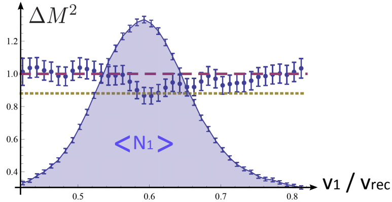
FIGURE 4.23 Variance du nombre d'atomes relatif (ronds bleus) en fonction de la position du centre de la première zone, la seconde étant fixe. Cette variance est inférieure à 1 au centre du nuage 1, dont la distribution de densité est représenté par la surface coloriée. La ligne en pointillés indique la variance minimale attendue ( \sigma_0^2 ), compte tenu de notre efficacité de détection.
