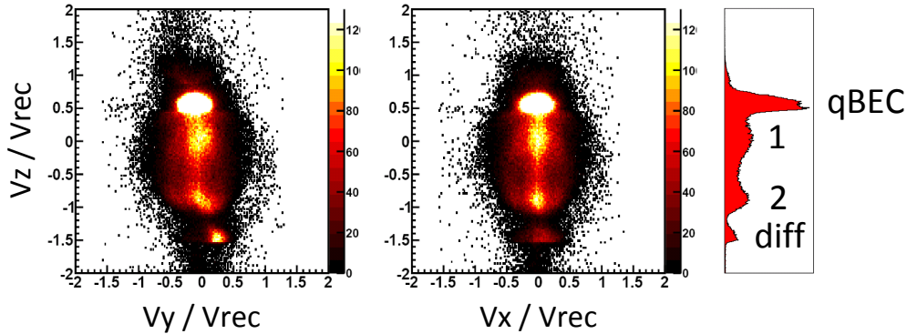
FIGURE 4.5 Coupes 2D et 1D des nuages détectés après temps de vol, les positions au niveau du détecteurs sont ici converties en vitesses. L'axe des vitesses verticales étant orienté vers le haut, les atomes ayant les plus grandes vitesses sont ceux qui arrivent en dernier sur le détecteur. L'origine de cet axe correspond à un condensat initialement au repos (dont le temps d'arrivée est de 307ms). Le pic principal correspond au quasi-condensat initial ("qBEC"), les deux pics suivants (1 et 2) sont formés par les paires, et le dernier ("diff") est un pic de diffraction du quasi-condensat.
