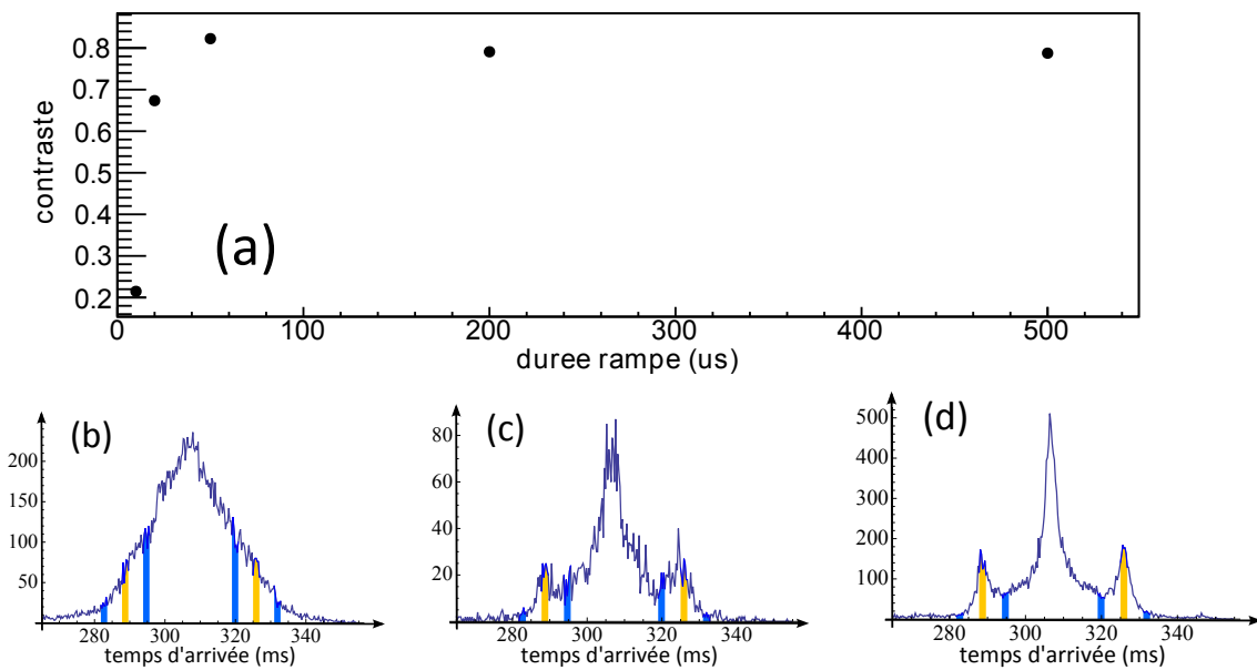
FIGURE 3.15 (a) Le contraste des pics de diffraction en fonction de la durée de la rampe de montée du réseau chute pour \tau < 50\mu\text{s} . Le contraste est défini comme C = (N_{pic} - N_{ref}) / (N_{pic} + N_{ref}) , où N_{pic} est le nombre d'atomes dans les 2 pics latéraux (zone orange sur les temps de vol) et N_{ref} est la moyenne de la population des zones de part et d'autres de ces pics (en bleu) : N_{ref} correspond au fond thermique à la position des pics. Les exemples de profils de temps de vol ont été obtenus pour des rampes de durée \tau = 10\mu\text{s} (b), \tau = 20\mu\text{s} (c) et \tau = 50\mu\text{s} (d).
