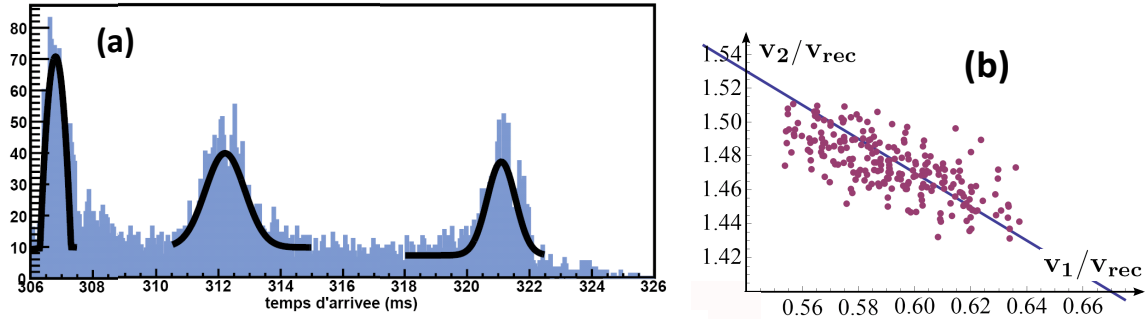
FIGURE 4.20 (a) Profil de temps de vol pour une réalisation expérimentale. L'ajustement du quasi-condensat par un profil parabolique marche mal, car la saturation lors de la détection rend le quasi-condensat asymétrique (cf §A.3). Les 2 autres pics sont ajustés par des gaussiennes. (b) On déduit de ces ajustements les vitesses centrales des 2 pics dans le référentiel du laboratoire, dont on voit ici qu'elles sont corrélées (points rouges), et superposées à la courbe d'accord de phase (en bleu). Les déplacements de v_1 et v_2 le long de cette courbe résultent des fluctuations de la vitesse initiale v_0 du quasi-condensat, alors que la dispersion autour de cette courbe provient des fluctuations de sa position initiale z_0 .
