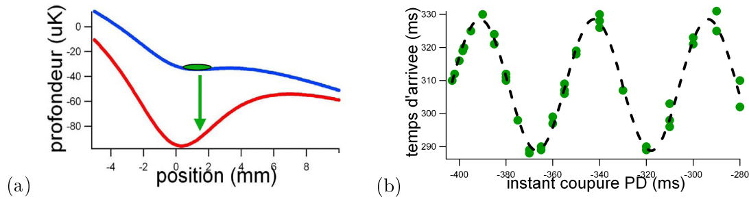
FIGURE 2.6 Lorsque la profondeur du piège optique est augmentée brusquement, le condensat est décalé par rapport au minimum du potentiel (a), ce qui excite une oscillation dipolaire (b).
