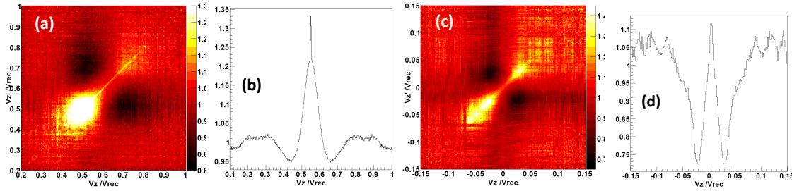
FIGURE 4.19 Agrandissement (a) et coupe selon l'antidiagonale (b) de la fonction de corrélation locale g^{(2)}(v_z, v'_z) du nuage en v_1 . La forme est similaire à celle que l'on obtenait pour un quasi-condensat sans réseau (c) et (d), bien que les largeurs ne soient pas du tout les mêmes. En effet, cette structure caractéristique apparaît sur les flancs de la distribution de densité, qui est beaucoup plus large pour le pic en v_1 que pour un quasi-condensat.
