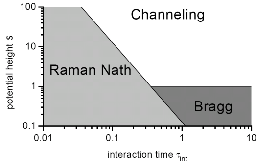
FIGURE 3.5 Régimes de diffraction en fonction de la durée \tau_{int} = T_L E_{rec}/\hbar et de la profondeur s = V_0/4E_{rec} du réseau, d'après [Keller 99]
