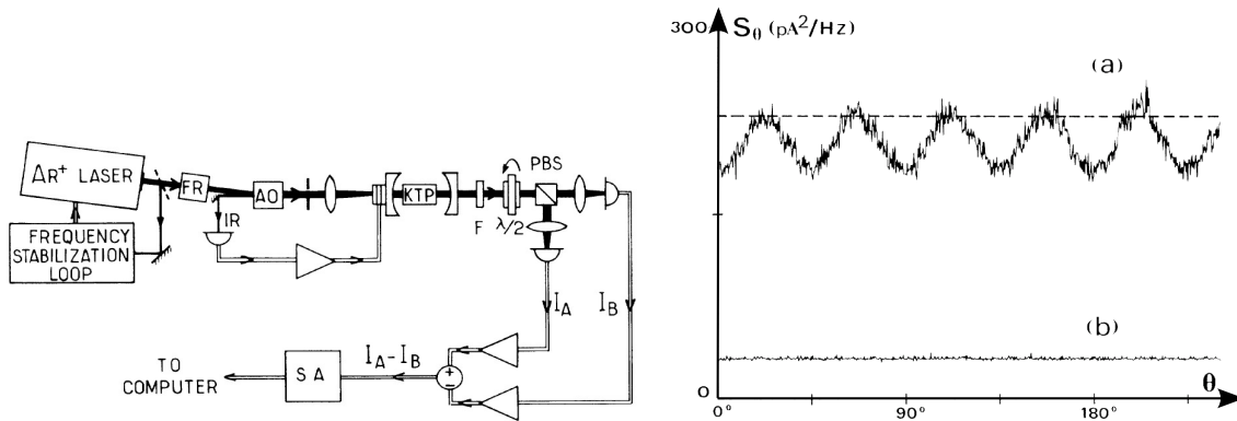
FIGURE 1.9 Dispositif expérimental et mesure des fluctuations d'intensité relative entre deux faisceaux jumeaux générés par conversion paramétrique de type II, en fonction de l'angle \theta de la lame d'onde ( \lambda/2 ). Cette fluctuation (a) est toujours inférieure au bruit de grenaille (indiqué en pointillés), sauf quand les faisceaux signal et complémentaire sont parfaitement mélangés dans les 2 voies de détections. Le bruit électronique est également représenté (b). Figures extraites de [Heidmann 87].
