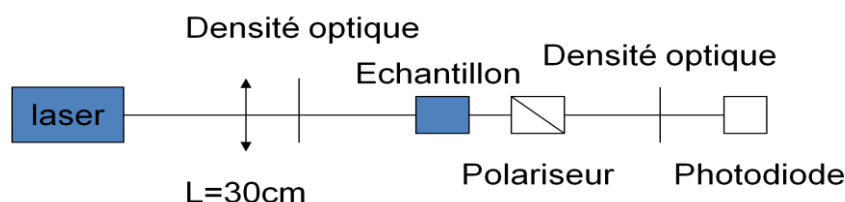
Figure 59 : Schéma expérimental pour l'étude de la polarisation de l'émission conique et du continuum de lumière blanche
