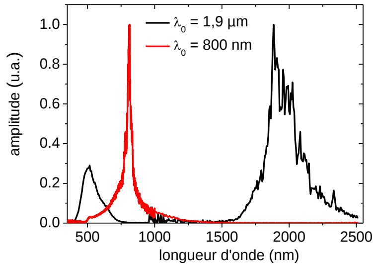
Figure 76 : Intégrale du spectre du continuum généré par filamentation dans la silice dans le cas d'un régime de dispersion normale (800 nm) et anormale (1,9 \mu\text{m} ).
