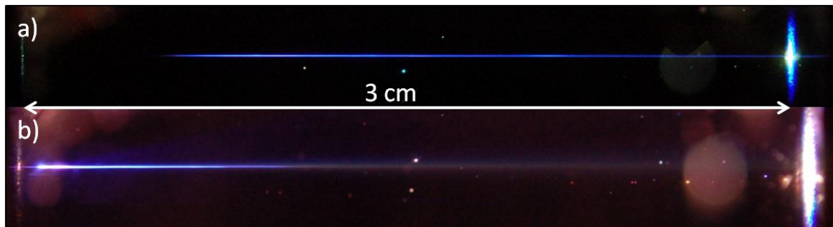
Figure 77 : Photographie d'un filament dans un cube de silice fondue de 3 cm d'épaisseur pour une impulsion de 15 \mu\text{J} , 50 fs a) pour \lambda_0 = 1,9 \mu\text{m} , b) pour \lambda_0 = 0,8 \mu\text{m} .
