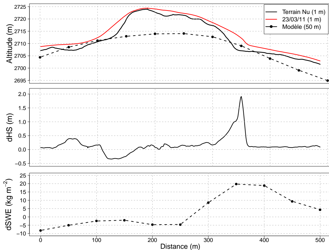
FIGURE 8.12 – Transect dans le sens Nord/Sud au Col du Lac Blanc. Haut : topographie du modèle (résolution horizontale de 50 m) et topographie observée avec et sans neige (résolution horizontale de 1 m). Milieu : différence de hauteur de neige mesurée entre le 28/02/11 et le 17/02/11. Bas : différence d'équivalent en eau simulée pour l'épisode du 18/03/11. La localisation du transect est indiquée sur la figure 8.11 (b). Les données observées ont été moyennées sur une bande large de 50 m représentant la taille d'un point de grille du modèle.
