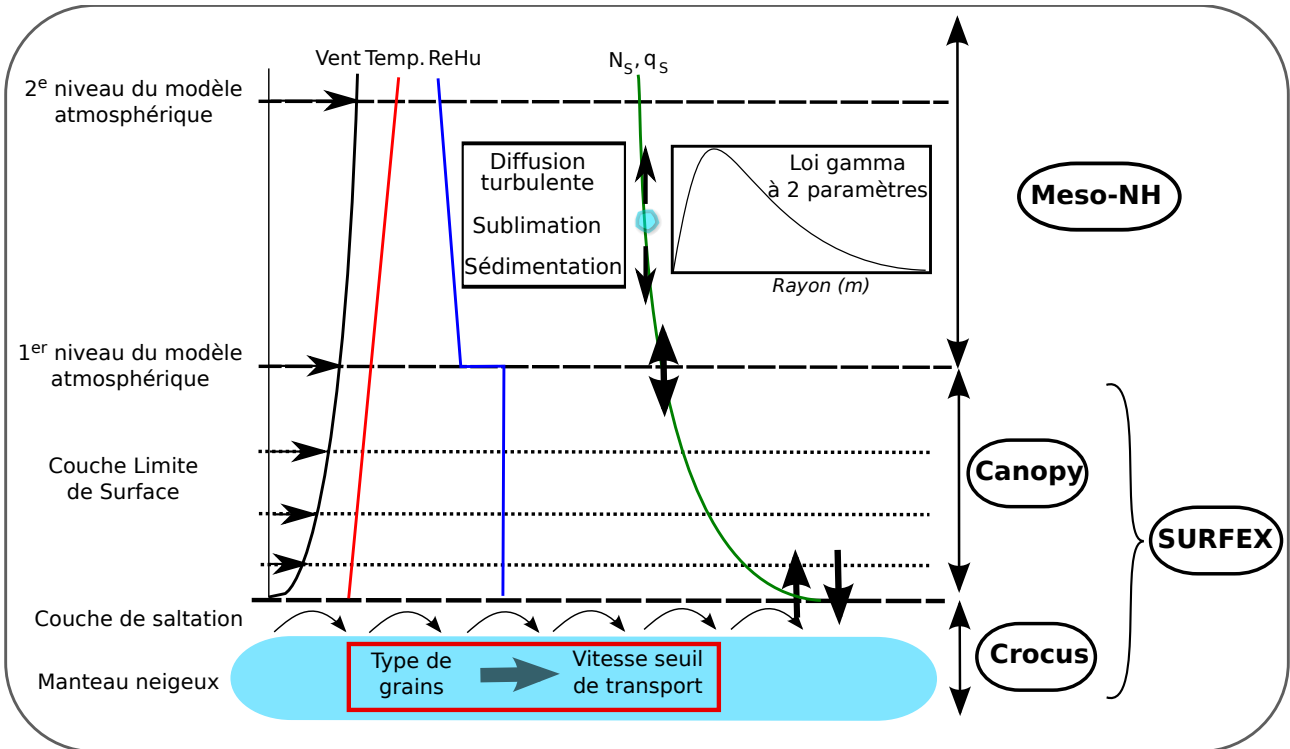
FIGURE 5.1 – Schéma de fonctionnement du module de transport de neige par le vent dans Meso-NH/Crocus. N_s ( \text{kg}^{-1} ) désigne le nombre de particules de neige en suspension par unité de masse de fluide et q_s ( \text{kg kg}^{-1} ), le rapport de mélange en particules de neige en suspension.
