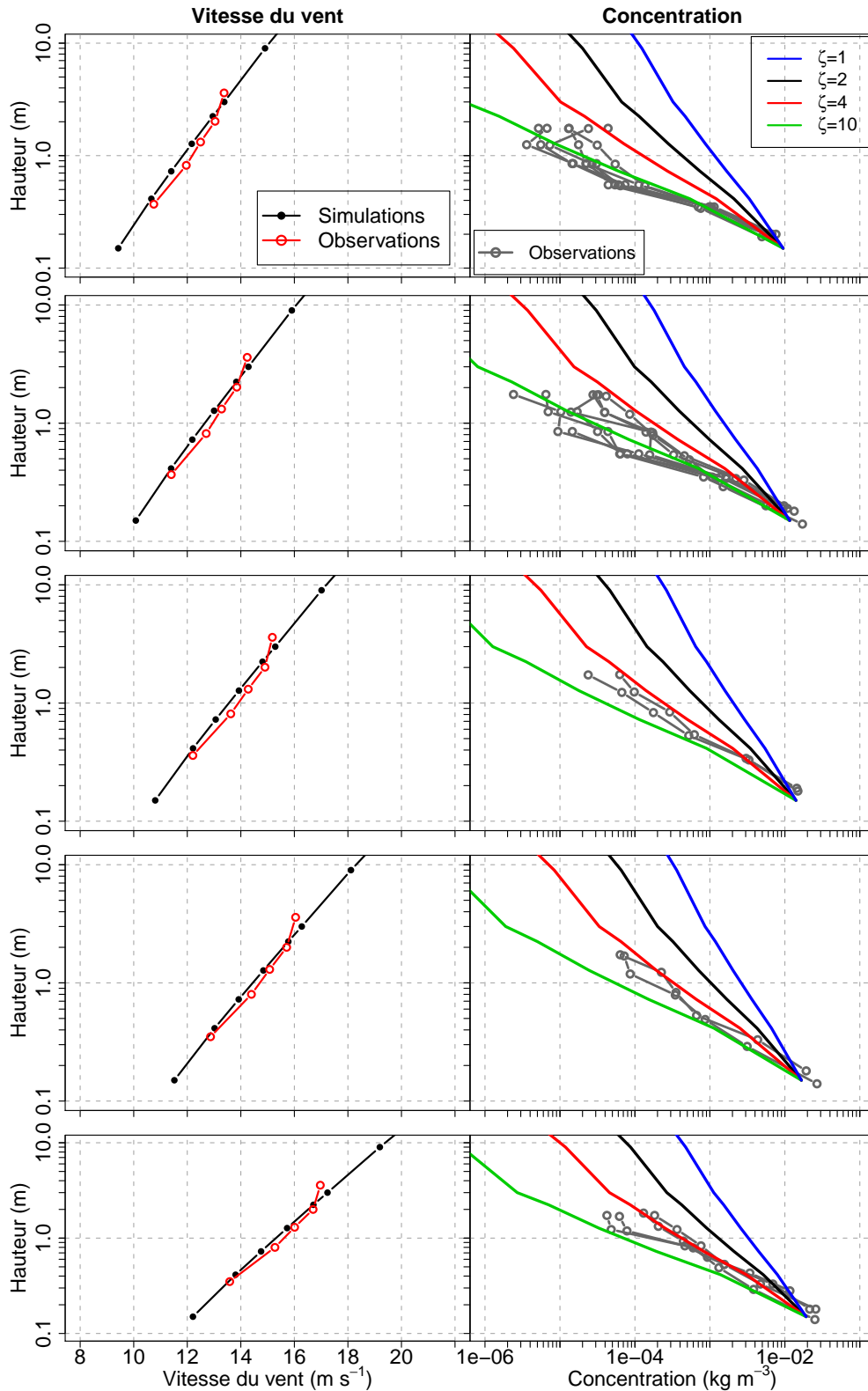
FIGURE 6.4 – Profils verticaux de vitesse de vent (gauche) et de concentration (droite) mesurés et simulés par Meso-NH/Crocus pour 5 catégories de vitesse de vent à 2.5 m le 18/03/11. Quatre valeurs du paramètre \zeta sont testées.
