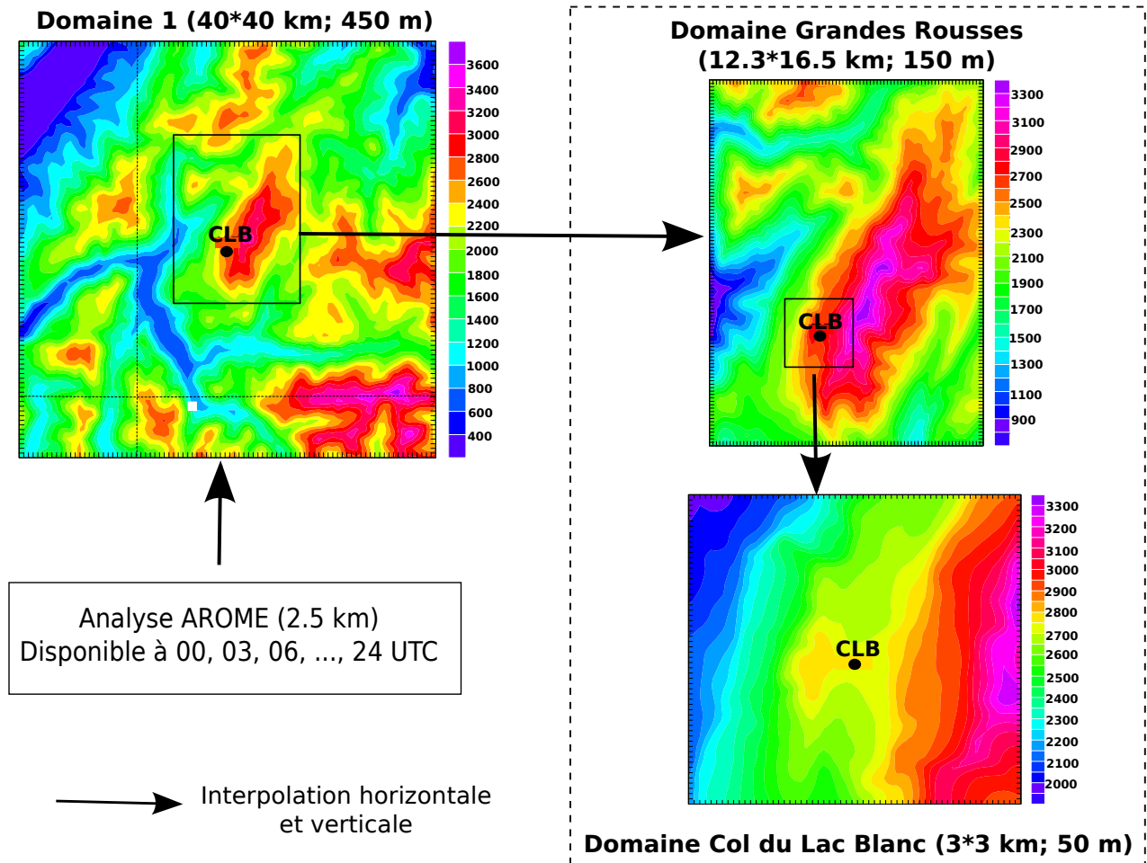
FIGURE 7.1 – Principe de fonctionnement de la descente d'échelle sur le site expérimental du Col du Lac Blanc. Le cadre en pointillé désigne les domaines sur lesquels les simulations de transport de neige par le vent seront effectuées.
