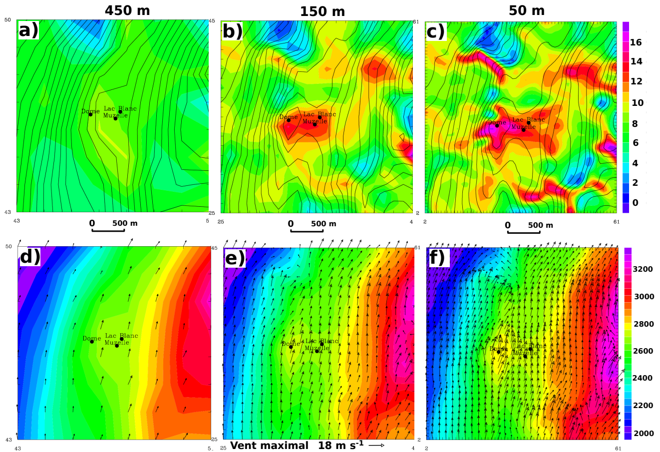
FIGURE 9.5 – Module ( a, b et c , en \text{m s}^{-1} ) et direction du vent ( d , e et f ) simulés autour du Col du Lac Blanc pour 3 résolutions horizontales différentes le 15/02/11 à 09h00. Pour des raisons de clarté, la figure f omet un vecteur vent sur deux. Les positions des 3 stations météo. automatiques sont indiquées sur chaque carte. L'orographie est représentée sous forme d'isolignes en trait continu sur a, b et c , et en couleur sur d , e et f .
