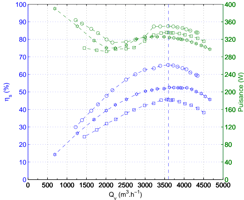
FIGURE 4.2 – Courbes de rendement statique (bleue) et de puissance absorbée par R1 (vert). ( \square ) pour R1, ( \diamond ) pour RS et ( \circ ) pour RR.
