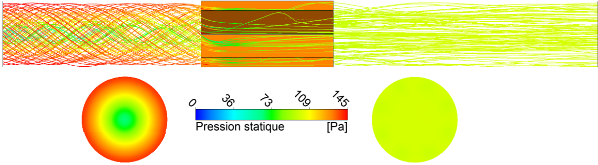
FIGURE 3.3 – Simulation numérique du redresseur positionné 3D en aval de l'entrée. La vitesse axiale imposée en entrée correspond au débit Q_v=1 \text{ m}^3 \cdot \text{s}^{-1} , soit une vitesse axiale de V_a=8.8 \text{ m} \cdot \text{s}^{-1} . Une composante tangentielle homogène de valeur V_\theta=7 \text{ m} \cdot \text{s}^{-1} est imposée. Cet ordre de grandeur est proche de celle sortant du rotor amont du système contrarotatif. En haut, sont tracées les lignes de courant depuis l'entrée du conduit jusqu'à la sortie. En bas, sont tracés les profils de pression statique à 0.5D en amont et en aval du redresseur.
