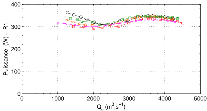
FIGURE 5.11 – Courbes de puissance pour R1 pour différentes distances axiales. La vitesse du rotor R1 est N_{R1}=2000 rpm et \theta=0.9 . (□) : R1 seul, (o) : A=0.17 , (☆) : A=0.86 , (□) : A=2.58 , (×) : A=3.1 .
