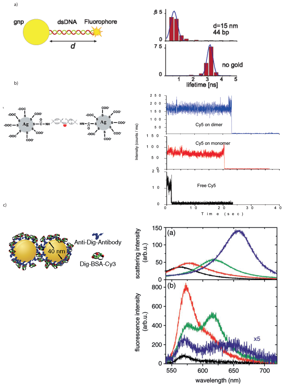
Figure 1.12 – Couplage par voie chimique : a) Molécule unique liée par un double brin d'ADN à une NP Au de 15 nm de diamètre, [20], b) mesures du signal de fluorescence de molécule dans des dimers d'argent de NPs de 20 nm de diamètre [21], c) mesures de la réponse spectrale de molécules à proximité de dimères de NPs Au de 40 nm de diamètre [23].
