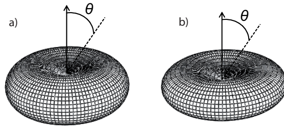
Figure 2.21 – Représentation tridimensionnelle des deux premiers termes de la série de la fonction de distribution D_\theta(\theta) , (a) D_\theta(\theta) = (2/\pi) \sin^2(\theta) , (b) D_\theta(\theta) = (8/3\pi) \sin^4(\theta)
