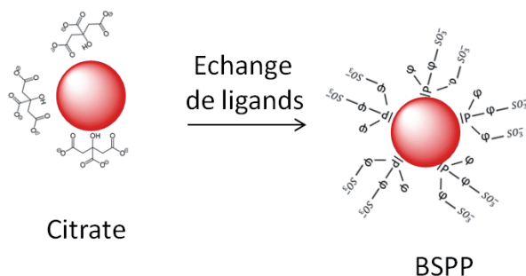
Figure 2.1 – Représentation schématique du premier échange de ligands. Les particules stabilisées avec du citrate sont passivées de bis(p-sulfonatophényl) phenylphosphine (BSPP) chargé négativement.
