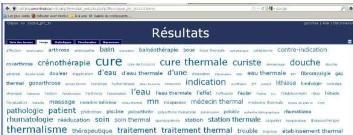
Figure 3 : fenêtre Nuage.
