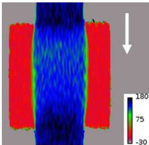
Figure 4.1 – Carte de vitesse dans une section longitudinale d'un pore de 7 \text{ cm} (diamètre et longueur de la boîte) pour V = 0,16 \text{ mm/s} . La vitesse (en microns par seconde) dans chaque voxel est représentée par une couleur selon l'échelle en bas à droite. La flèche indique le sens de l'écoulement, i.e. de haut en bas.
