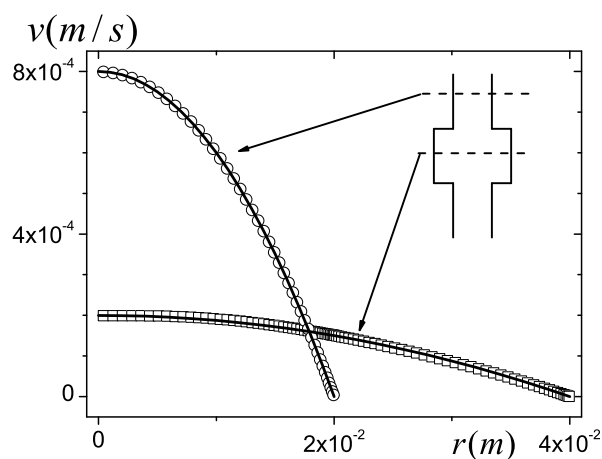
Figure 4.20 – Profils de vitesse longitudinale dans la petite conduite (ronds), à z = -0.08m , et au centre du pore (carrés), à z = 0.04m , pour le même écoulement que celui de la figure 4.19 dans un pore avec LR = 1 , CR = 2 , Bi = 10^{-3} et le maillage M4 . Les lignes continues représentent le profil théorique d'écoulement dans une conduite simple.
