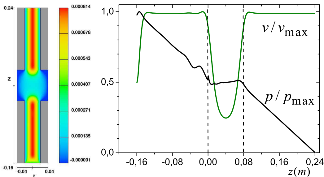
Figure 4.19 – Pore avec LR = 1 , CR = 2 , Bi = 10^{-3} et le maillage M4 . A gauche, le champ de vitesse longitudinale. La hauteur z et la largeur r sont exprimées en m . La vitesse dans chaque voxel (en m/s ) est représentée par une couleur selon l'échelle à droite de l'image. A droite, la vitesse longitudinale (en vert) et la pression (en noir) sur l'axe de révolution en fonction de la hauteur, ces deux grandeurs sont adimensionnées par leur valeur maximale. L'écoulement a lieu de bas en haut.
