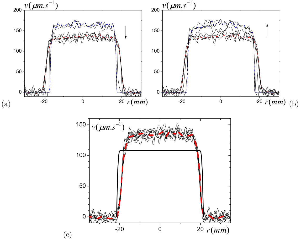
Figure 4.3 – Ecoulement d'un fluide à seuil à travers une boîte cylindrique (à V = 0,16\text{mm/s} ) : profils de vitesse longitudinale obtenus à partir des images en fonction de la distance à l'axe de symétrie à différentes position z séparées par des intervalles de 0,5\text{cm} : (a) de 0,5 à 4,5\text{cm} (entrée), (b) de -4,5 à 0,5\text{cm} (sortie), (c) de -1,5 à 1,5\text{cm} (centre). La ligne pointillée bleue est la vitesse moyennée entre 3,5 et 4,5\text{cm} dans (a) et entre -4,5 et -3,5\text{cm} dans (b). La ligne pointillée rouge est la vitesse moyennée entre -1,5 et 1,5\text{cm} . La ligne noire continue (en trait épais) correspond à la théorie d'un écoulement uniforme dans une conduite d'un rayon de 21,5\text{mm} . La flèche indique le sens de l'écoulement.
