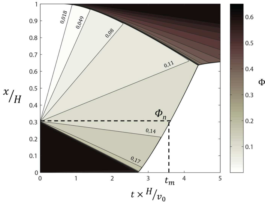
Figure 9.18 – Diagramme spatio-temporel théorique de la fraction volumique \Phi de microcapsules qui crèment dans une colonne d'eau. Paramètre de la loi de Richardson-Zaki : n = 6,5 .
