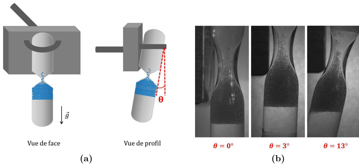
Figure 9.10 – (a) Schéma de fixation du sablier sur son support. Vue de face, le sablier est maintenu vertical. L'effet de la position du sablier sur la vitesse d'écoulement a été étudiée en variant l'angle \theta . (b) Photos du Sablier C pour les trois angles \theta étudiés dans l'expérience.
