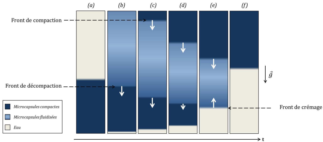
Figure 9.22 – Représentation schématique du crépage de microcapsules d'huile dans une colonne d'eau. Les flèches blanches traduisent le mouvement de la position des différents fronts.
