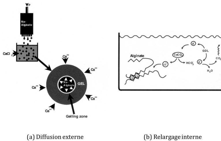
Figure 3.3 – Les deux principales techniques de gélification de l'alginate : (a) par diffusion externe, illustrée par la technique d'immobilisation dans une bille de gel et (b) par relargage interne, illustrée par la libération de \text{Ca}^{2+} à partir de \text{CaCO}_3 et Delta-gluconolactone (GDL). Adapté de [Draget et al., 2005].
