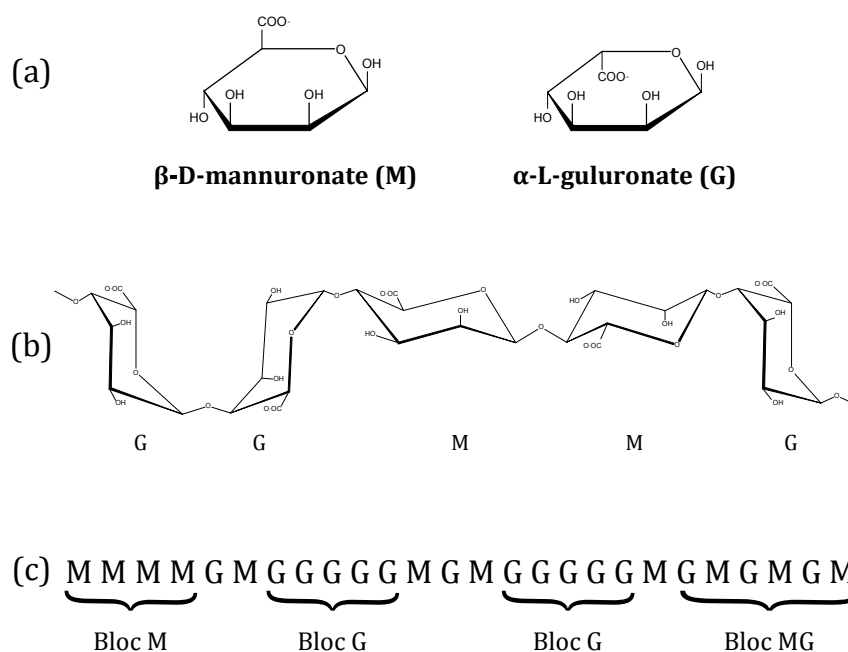
Figure 3.1 – Structure et composition de l'alginate : (a) monomères d'acides uroniques, (b) conformation des chaînes et (c) distribution des blocs.
