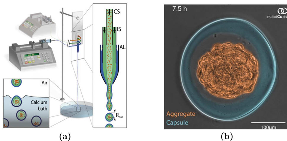
Figure 2.15 – (a) Schéma du procédé microfluidique de fabrication des microcapsules à membrane d'alginate. La phase interne contient une suspension de cellules tumorales. La phase intermédiaire est une solution aqueuse sans calcium et sert de barrière à la diffusion des ions calcium contenus dans le milieu cellulaire et qui pourraient gélifier l'alginate et boucher le capillaire. (b) Image de la croissance d'un agrégat de capsules dans une capsule prise 7,5 heures après le formation de la capsule. Adapté de [Alessandri et al., 2013]
