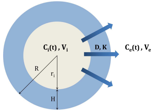
Figure 5.3 – Schéma d'une capsule millimétrique à cœur aqueux contenant un soluté à la concentration C_i et une membrane huileuse d'épaisseur H .
