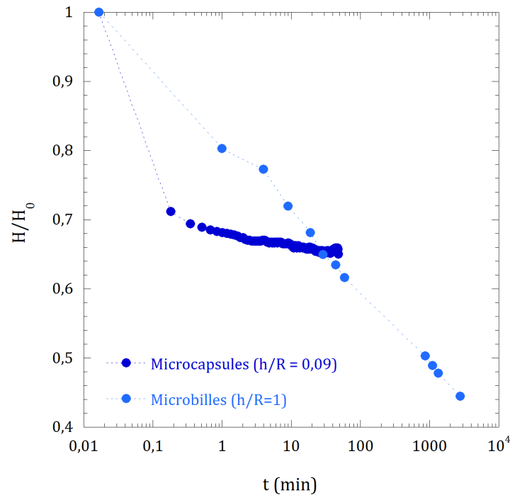
Figure 8.2 – Variation de la hauteur H de microcapsules et de microbilles normalisée par la hauteur initiale H_0 en fonction du temps après l'application d'un piston de masse égale 630 g (respectivement 304 g).
