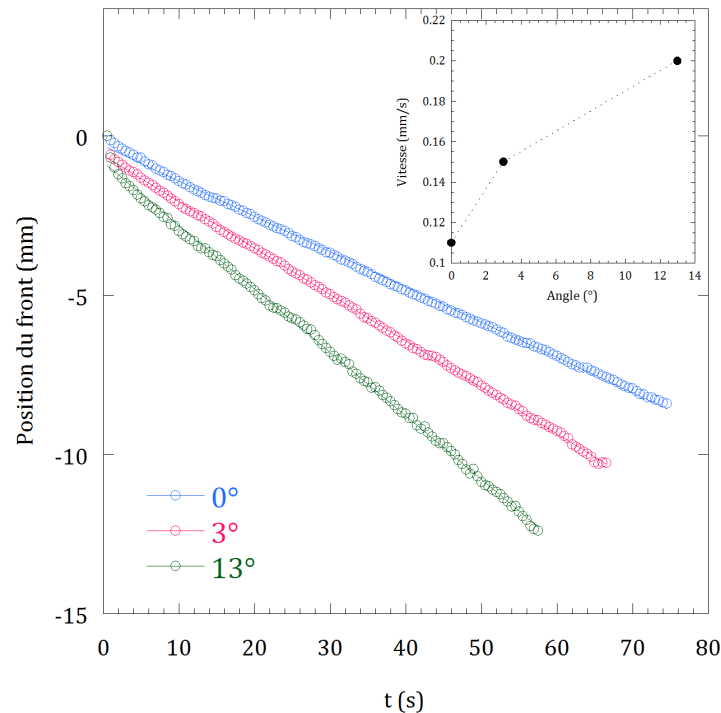
Figure 9.11 – Position du front arrière en fonction du temps pour trois différents angles \theta . Inséré : Vitesse du front en fonction de l'angle du sablier. Expérience réalisée avec le Sablier C et les billes de 550 \mu\text{m} de diamètre.
