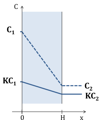
Figure 5.2 – Schéma du profil de la concentration en soluté dans la membrane modifié par le coefficient de partage K .
