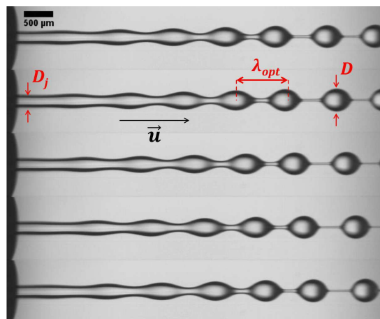
Figure 2.12 – Fragmentation d'un jet composé d'alginate et d'une solution de Dextran. Fréquence d'excitation = 1500 Hz, \Delta t=0,1ms . Pour des raisons de commodités, les clichés sont présentés horizontalement, mais il faut bien imaginer un jet vertical dans l'expérience. (Crédits Hugo Doméjean).
