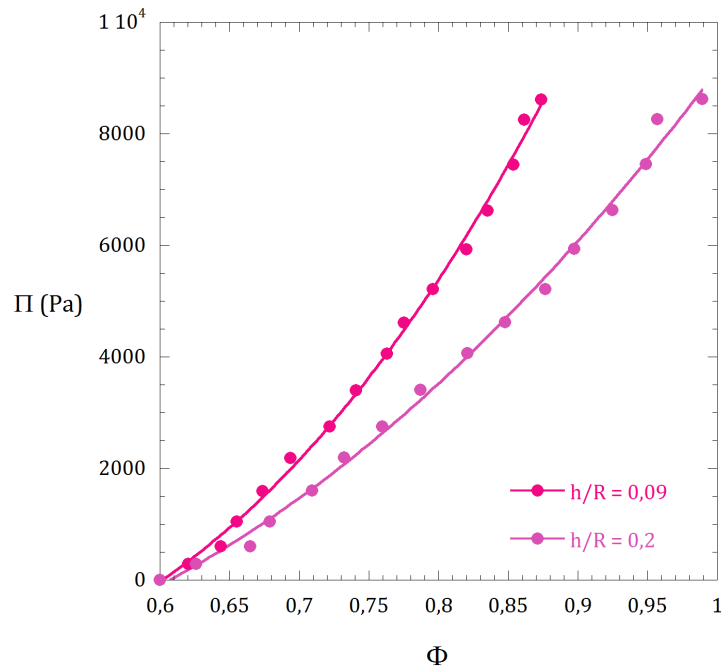
Figure 8.4 – Équation d'état d'une dispersion de capsules d'alginate pour deux ratios h/R . Les points expérimentaux ont été ajustés par l'équation \alpha\Phi^\beta(\Phi - \Phi^*) .
