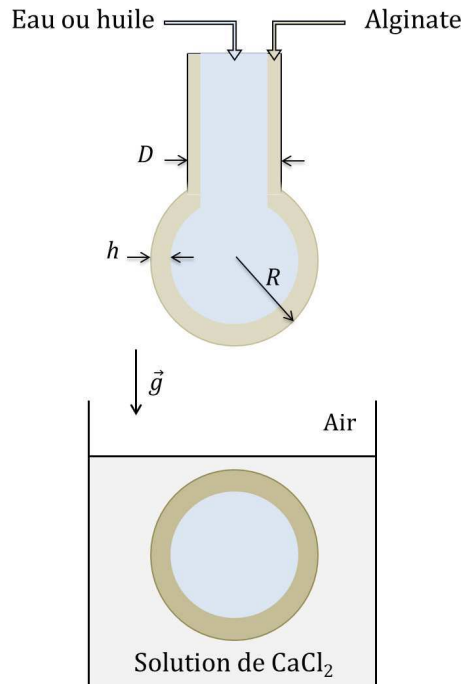
Figure 2.5 – Schéma du procédé de fabrication des capsules. Une bi-goutte est formée par co-extrusion de la solution de cœur (eau ou huile) et la solution d'alginate. En tombant dans une bain de calcium, l'alginate gélifie instantanément pour former une capsule à cœur liquide et membrane fine d'hydrogel.
