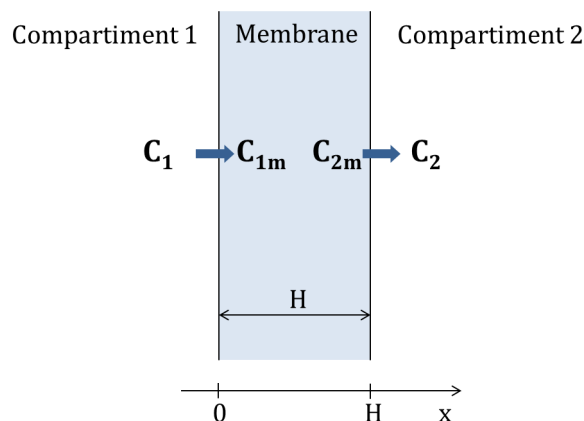
Figure 5.1 – Représentation de la diffusion d'un soluté d'un compartiment 1 à la concentration homogène C_1 vers un compartiment 2 à la concentration homogène C_2 à travers une membrane.
