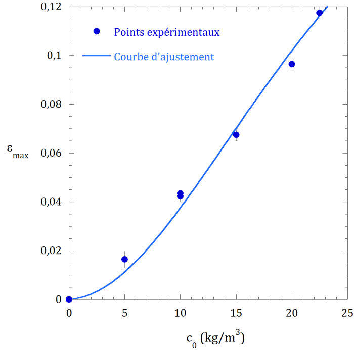
Figure 7.7 – Déformation maximale de la capsule \epsilon_{max} = \Delta R/R_0 obtenue à l'équilibre de gonflement en fonction de la concentration initiale dans le cœur c_0 . Les points expérimentaux ont été ajustés par l'équation (7.9), permettant d'obtenir un module moyen E égal à 70 kPa.
