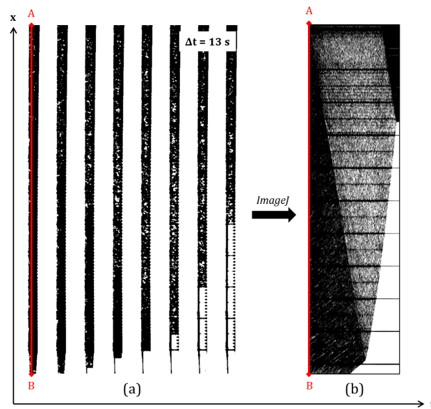
Figure 9.20 – Analyse de l'expérience de crémage des microcapsules : (a) Échantillon d'images ( \Delta t = 13s ) enregistrées avec la caméra Pixelink. Le segment AB est une ligne de 1 pixel d'épaisseur correspondant au milieu de la colonne. (b) Diagramme spatio-temporel obtenu par juxtaposition des coupes AB sur chaque image, réalisé avec le logiciel ImageJ. L'expérience a été réalisée avec des capsules de diamètre 412 \mu\text{m} et un diamètre de tube D égal à 3 mm.
