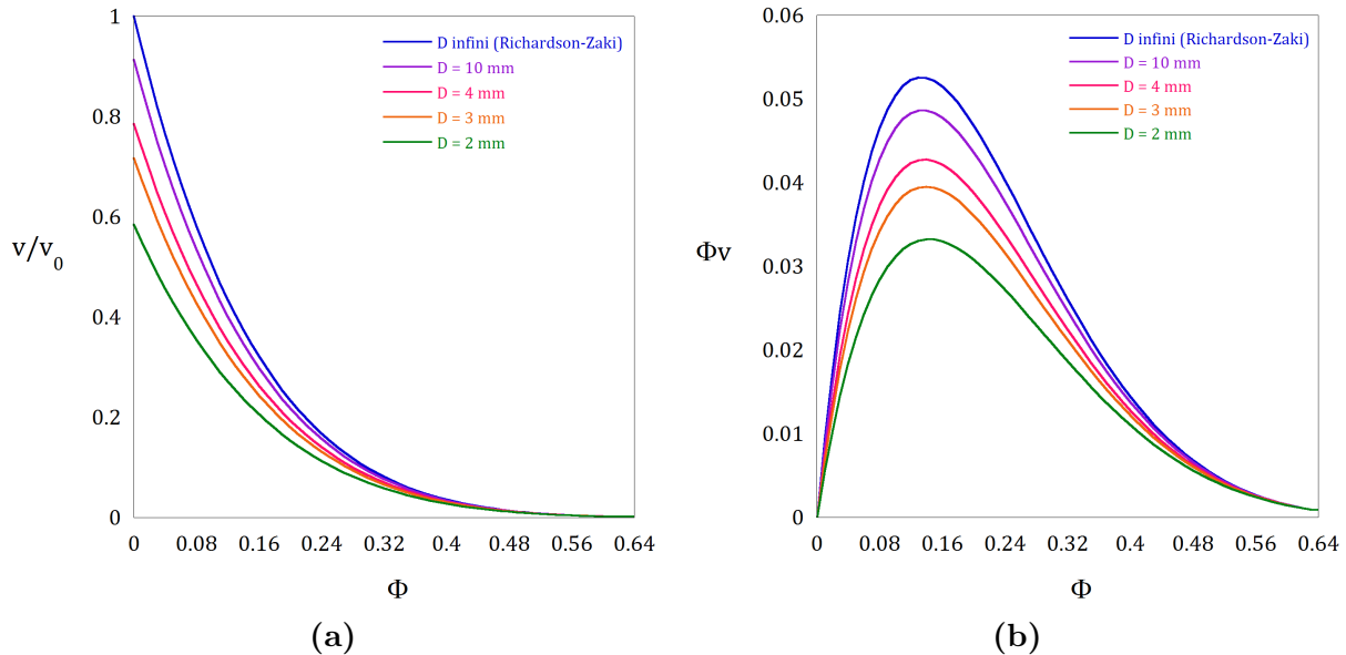
Figure 9.19 – (a) Lois de vitesse des particules en fonction de \Phi pour différents diamètres. (b) Flux de particules \Phi v en fonction de la fraction volumique \Phi pour différents diamètres.
