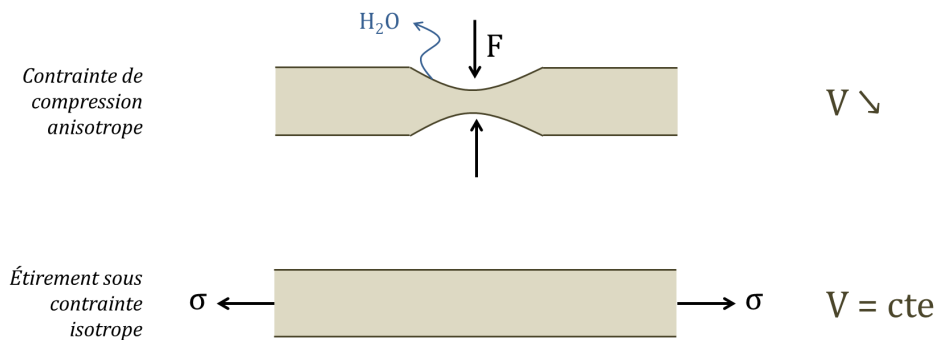
Figure 8.7 – Lorsque le gel est soumis à une compression anisotrope, l'eau est expulsée du gel et son volume diminue. Soumis à un allongement isotrope, le gel est étiré mais son volume reste constant. La plasticité est plus grande dans le premier cas.
