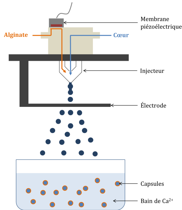
Figure 2.11 – Schéma du dispositif de fabrication des micro-capsules par fragmentation d'un jet composé inspiré d'un appareil commercial ( Encapsulator STARTUP ) et optimisé par H. Doméjean.
