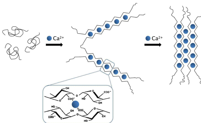
Figure 3.2 – Gélification de l'alginate par des ions calcium, selon de modèle "boite d'oeufs". Les blocs G de deux chaînes sont d'abord dimérisés par une liaison électrostatique avec un cation \text{Ca}^{2+} , puis ensuite polymérisés afin de former un gel dur.
