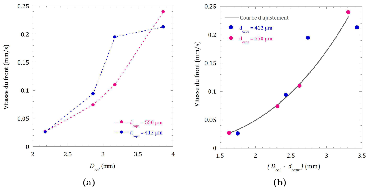
Figure 9.13 – (a) Vitesse de montée du front de capsules en fonction du diamètre du col pour deux tailles de capsules. (b) Vitesse de montée du front de capsules en fonction de la différence entre le diamètre du col et de diamètre des capsules ( D_{col} - d_{capsules} ) pour deux tailles de capsules.
