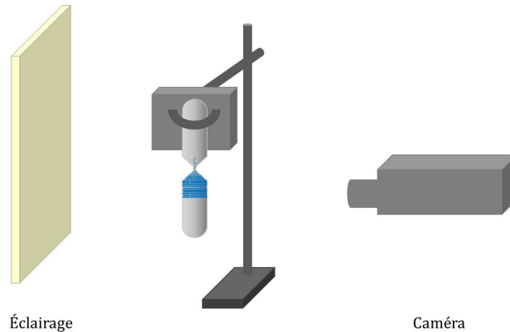
Figure 9.7 – Schéma de l'expérience d'enregistrement de l'écoulement des microcapsules dans un sablier.
