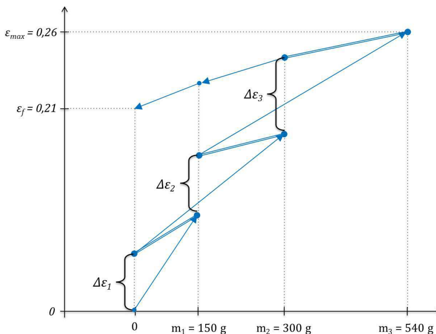
Figure 8.6 – Schéma de la courbe d'hystérèse du système. Inséré : Courbe expérimentale correspondante.
