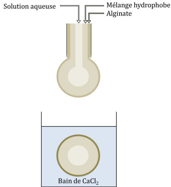
Figure 2.9 – Principe de fabrication d'une DuoPearl Inverse TM par un procédé millifluidique de coextrusion à trois voies.
