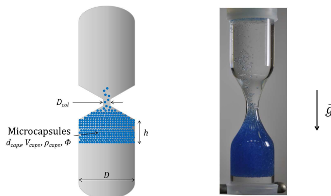
Figure 9.6 – Schéma et photo d'un sablier "liquide" rempli d'eau et d'un volume V_{caps} de microcapsules d'huile. Le diamètre intérieur du col du sablier est appelé D_{col} . Les microcapsules ont un diamètre d_{caps} , une masse volumique \rho_{caps} et leur fraction volumique est \Phi .
