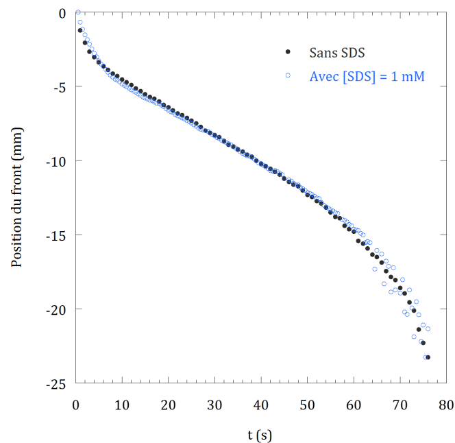
Figure 9.14 – Position du front de capsules en fonction du temps dans le Sablier C avec et sans SDS.
