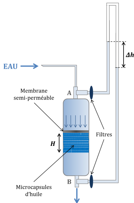
Figure C.1 – Schéma de l'expérience de lit fluidisé avec les microcapsules de diamètre 412 \mu\text{m} . Les deux filtres situés aux points A et B servent de résistance (perte de charge) et évitent que l'écoulement de l'eau ne soit dévié de la colonne.
