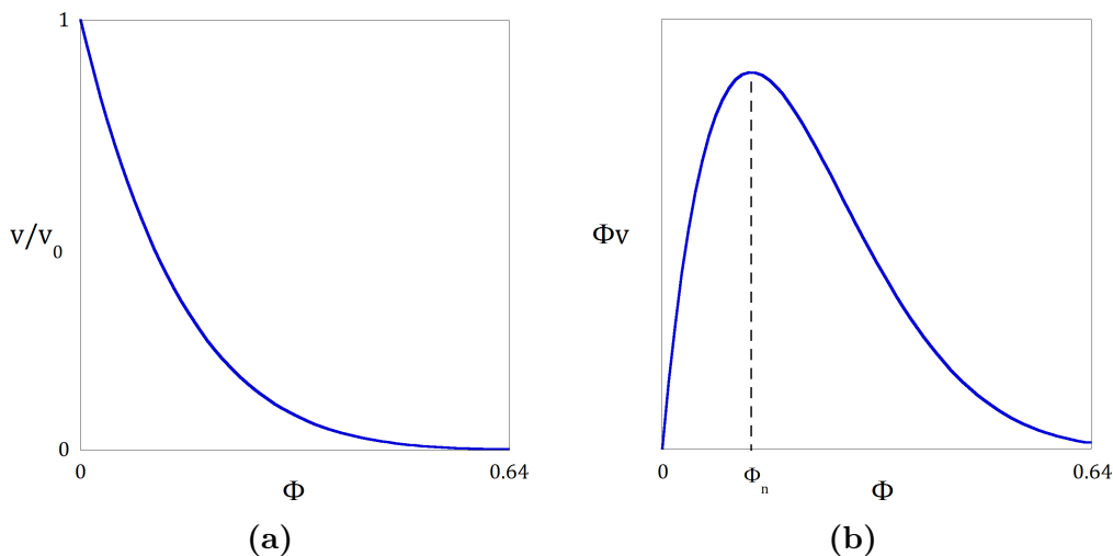
Figure 9.16 – (a) Allure de la loi de Richardson-Zaki (équation (9.10)). (b) Flux de particules \Phi v en fonction de la fraction volumique \Phi .
