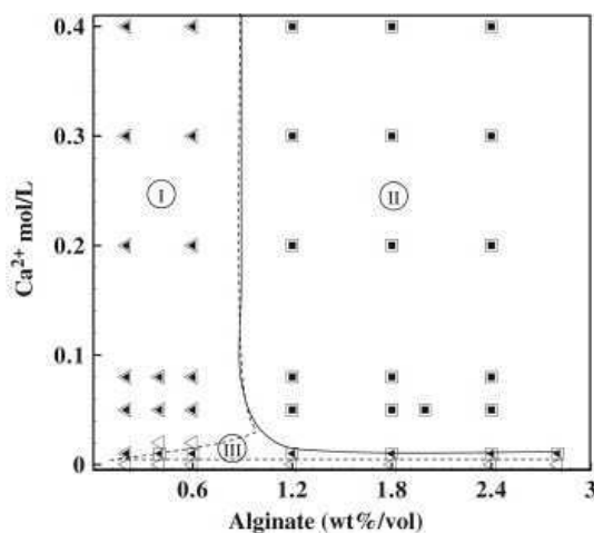
Figure 3.6 – Diagramme de la transition sol-gel de l'alginate de calcium réalisé dans les travaux de Zhao et al. [2011]. La région I correspond à l'état sol et la région II correspond à l'état gel .
