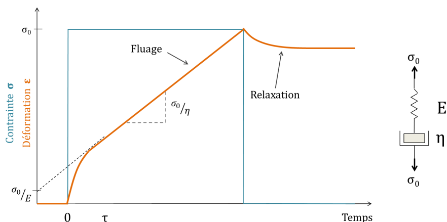
Figure 6.2 – Comportement d'un liquide viscoélastique soumis à l'action soudaine d'une contrainte et schéma du modèle de Maxwell.
