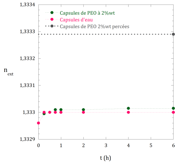
Figure 7.4 – Mesure de la fuite du PEG par réfractométrie. Quatre capsules sont immergées dans 500 \mu\text{L} d'eau ultra pure et l'indice de la solution extérieure n est mesuré en fonction du temps. L'expérience est réalisée avec des capsules contenant du PEG à 2% (points verts). À la fin de l'expérience, les capsules sont percées volontairement pour déterminer l'indice maximal de saturation (point gris). L'expérience de référence est réalisée avec des capsules contenant uniquement de l'eau pure (points roses).
