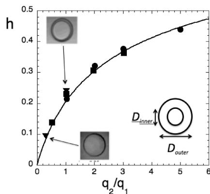
Figure 2.4 – Épaisseur relative h = (D_{outer} - D_{inner})/D_{outer} de la membrane de microcapsules de PNIPAM fabriquées par microfluidique, en fonction du ratio des débits entre les fluides interne et intermédiaire. Adapté de [Hennequin et al., 2009].
