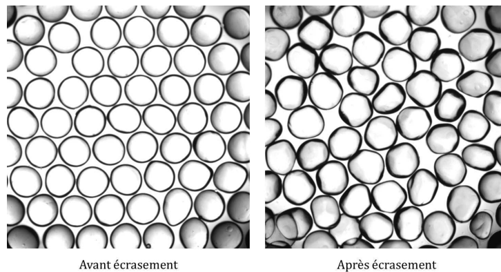
Figure 8.8 – Photo des microcapsules avant et après l'expérience de compression. Le diamètre initial des capsules est de 550 \mu\text{m} .
