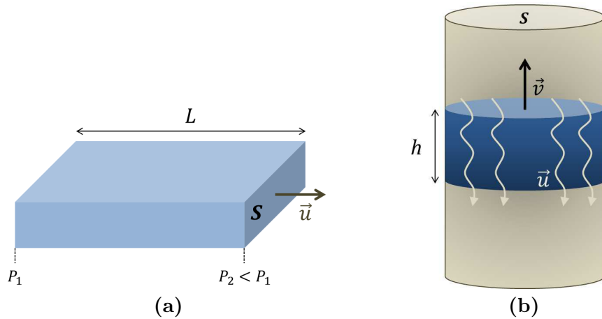
Figure 9.15 – (a) Schéma montrant les paramètres intervenant dans l'écoulement d'un fluide à travers un milieu poreux. (b) Schéma du modèle de crémage d'un lit de capsules d'huile dans l'eau, dans un cylindre à section constante.
