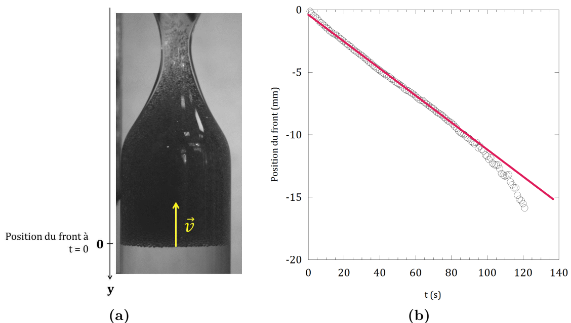
Figure 9.9 – (a) Image du front de capsules dans un sablier à t = 0 . (b) Courbe typique obtenue pour la position du front en fonction du temps. Expérience réalisée avec le Sablier C et des capsules de 550 \mu\text{m} de diamètre.
