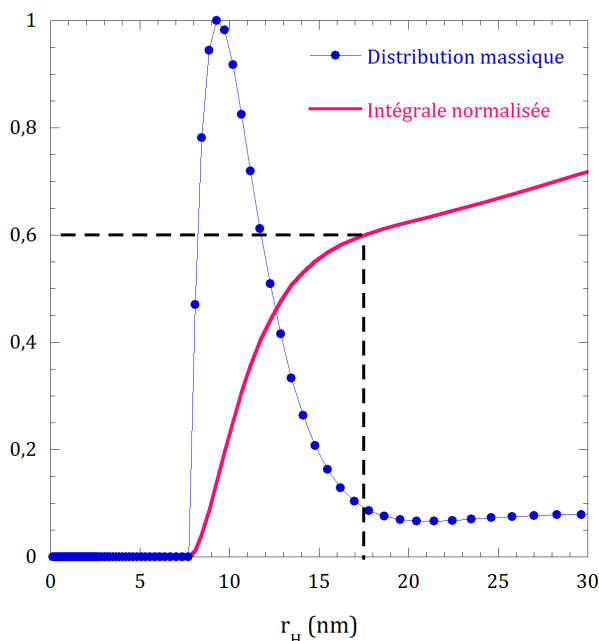
Figure 4.6 – Courbe de distribution en volume du Dextran 2000 mesurée par DLS et intégrale normalisée en fonction du rayon hydrodynamique r_H .
