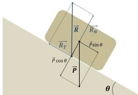
Figure 9.1 – Schéma d'un solide en équilibre sur une surface inclinée.
