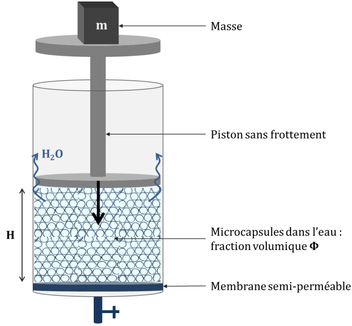
Figure 8.1 – Schéma de l'expérience de compression d'une pile de microcapsules d'huile dispersées dans l'eau par ajout d'une masse sur un piston sans frottement.
