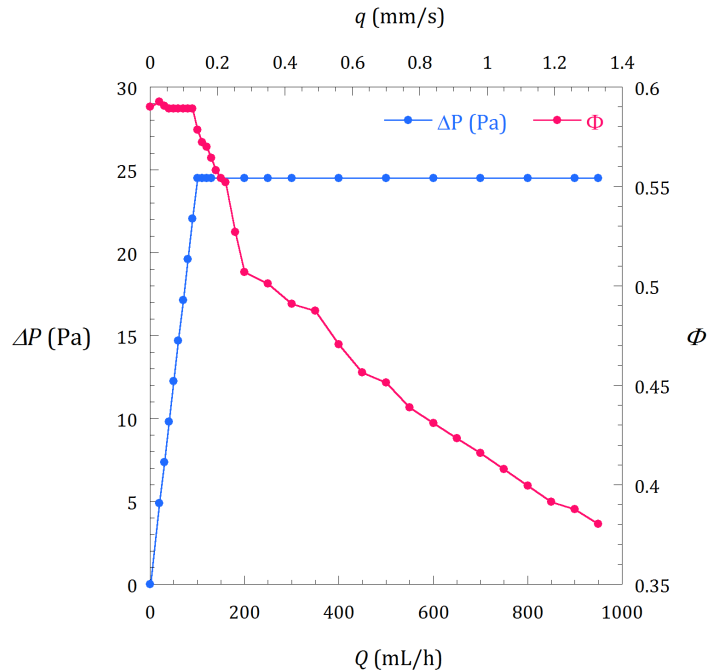
Figure C.2 – Variation de la différence de pression \Delta P entre les extrémités de la colonne et de la fraction volumique du lit de capsules \Phi en fonction du débit d'écoulement de l'eau Q (ou de sa vitesse q = Q/S ). L'expérience a été réalisée avec des capsules de diamètre égal à 412 \mu\text{m} .
