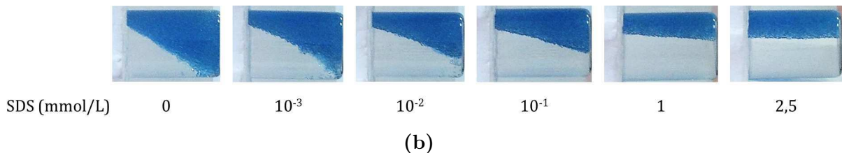
Figure 9.4 – (a) Schéma de l’expérience définissant l’angle de friction et le calcul du coefficient de friction. (b) Photo de l’expérience de variation de l’angle de friction en fonction de la concentration en SDS dans la phase continue.
