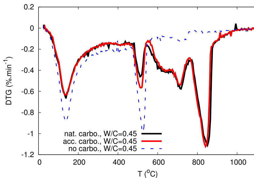
Fig. 3.22 – DTG sur pâtes de ciment (pâte CN) carbonatées en conditions de carbonatation naturelle et accélérée (10 % de \text{CO}_2 ) comparé au cas NC. Les trois modes de décomposition de \text{C}\bar{\text{C}} sont présents, même pour les conditions naturelles de carbonatation.
