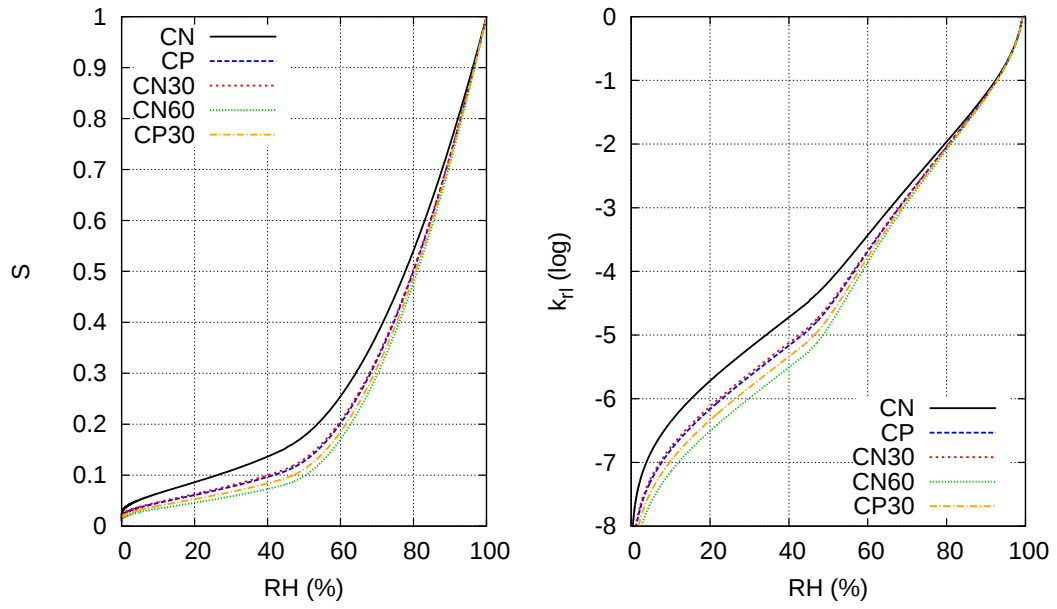
Fig. B.4 – Taux de saturation en fonction de HR (Eq.B.14) et k_{rl} , perméabilité relative à l'eau liquide, déduite par intégration numérique de la courbe p_c = f(S) [189].
