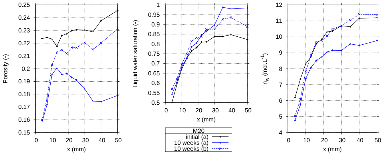
Fig. 4.10 – Mortier M20 : profils de porosité \phi_\gamma (cf. Eq. 2.5), de saturation en eau liquide S_w (cf. Eq. 2.6) et de teneur en eau n_w (mol.L ^{-1} ) (cf. Eq. 2.7), à l'état initial et après 10 semaines de carbonatation accélérée. On observe des résultats différents entre les éprouvettes labellisées (a) et (b) (cf. § 2.4.2) dus à un phénomène de ségrégation lors de la fabrication.
