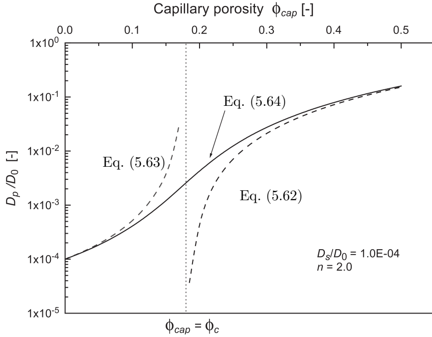
Fig. 5.17 – Lois d'évolution du coefficient de diffusion au sein du milieu poreux en fonction de l'évolution de la porosité, d'après [194, 199]
