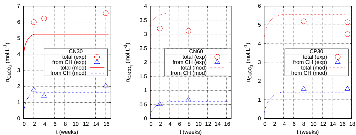
Fig. 6.7 – Teneur en \text{CC} après calibration de la cinétique de dissolution de CH pour les pâtes de ciment CN30, CN60 et CP30.
