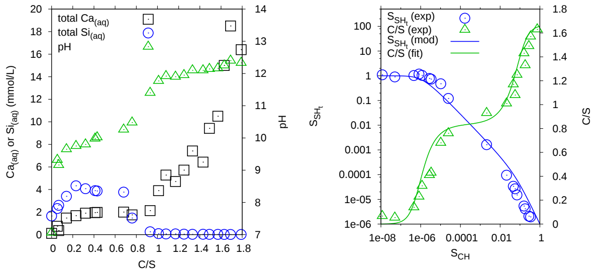
Fig. 5.3 – Comparaison entre le modèle thermodynamique proposé Eq. (5.21) (en traits pleins) et les données expérimentales de Greenberg et Chang [172] (points).
