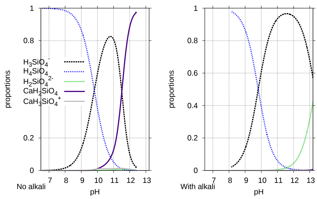
Fig. 5.7 – Spéciation du silicium. L’ajout des alcalins (à droite) a une forte influence sur la distribution des espèces en solution.
