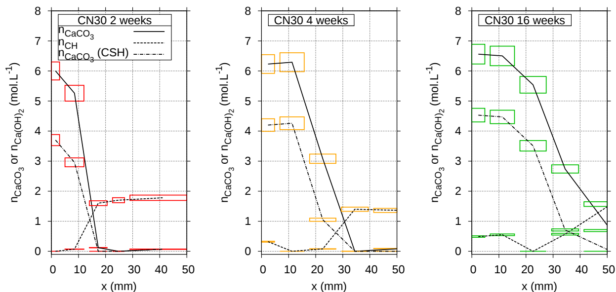
Fig. 4.18 – Profils de teneur en \overline{\text{C}}\overline{\text{C}} totaux, CH et \overline{\text{C}}\overline{\text{C}} issus de la carbonatation des C-S-H pour CN30 après 2, 4 et 16 semaines de carbonatation accélérée.
