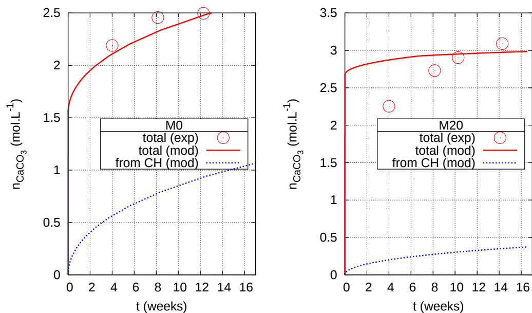
Fig. 6.8 – Teneur en \text{CC} après calibration de la cinétique de dissolution de CH pour les mortiers M0 et M20.
