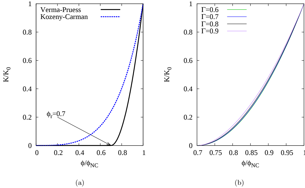
Fig. 5.14 – Courbe (a) : comparaison entre les modèles d'évolution de la perméabilité selon [182] ou [183] et influence du paramètre \Gamma sur le modèle de Verma et Pruess, courbe (b) ; pour une valeur de \phi_r = 0,7 .
