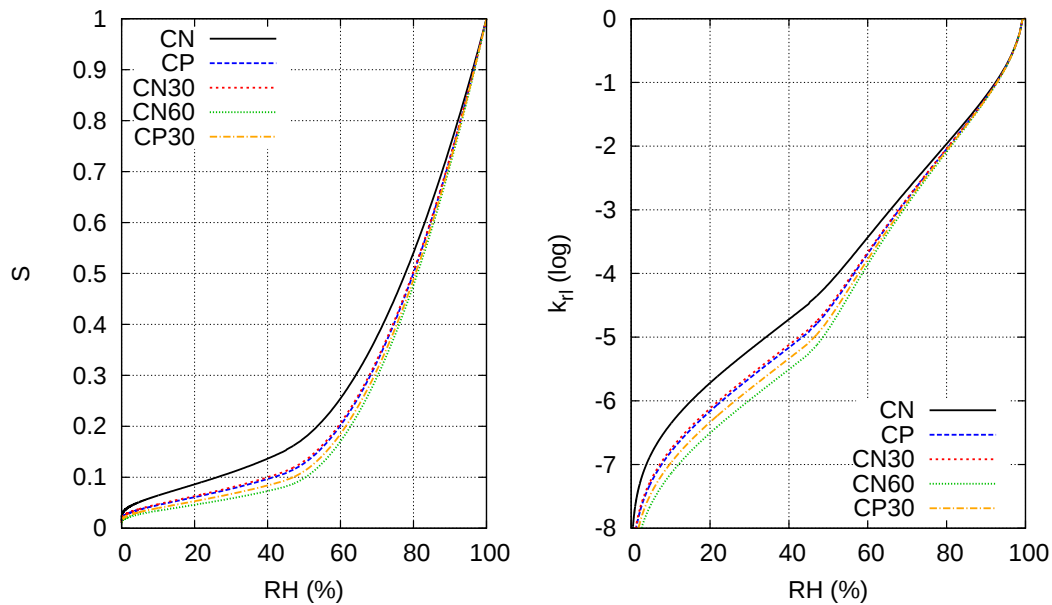
Fig. 5.15 – Taux de saturation en fonction de HR (Eq. B.14) (modélisation) et k_{rl} , perméabilité relative à l'eau liquide, déduite par intégration numérique de la courbe p_c = f(S) [189] pour les pâtes de ciment étudiées. Courbes de désorption.
