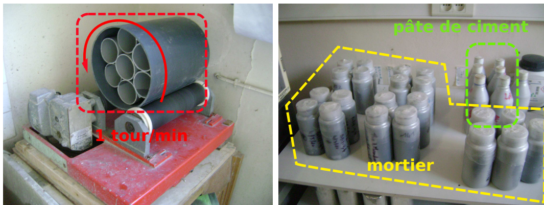
Fig. 2.1 – Dispositif anti-ségrégation utilisé et bouteilles non sciées en phase de conservation.
