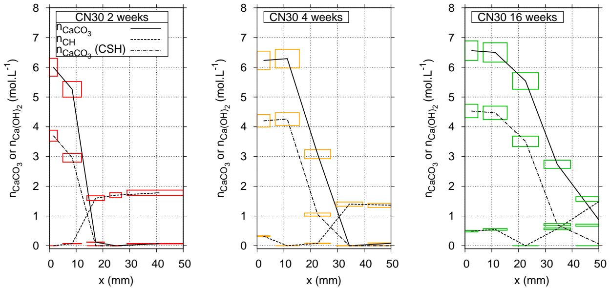
Fig. 4.18 – Profils de teneur en \overline{C\overline{C}} totaux, CH et \overline{C\overline{C}} issus de la carbonatation des C-S-H pour CN30 après 2, 4 et 16 semaines de carbonatation accélérée.
