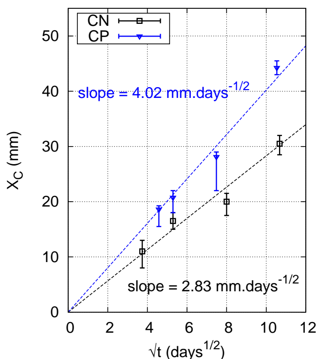
Fig. 3.9 – Évolution de la profondeur de carbonatation mesurée par projection de phénolphtaléine pour les deux formulations CN et CP. Les barres d'erreur présentent le minimum et le maximum des résultats obtenus sur les 12 valeurs mesurées.
