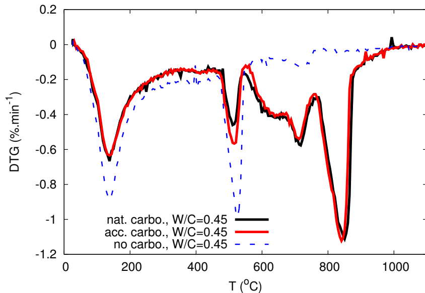
Fig. 3.22 – DTG sur pâtes de ciment (pâte CN) carbonatées en conditions de carbonatation naturelle et accélérée (10 % de CO 2 ) comparé au cas NC. Les trois modes de décomposition de C-C sont présents, même pour les conditions naturelles de carbonatation.
