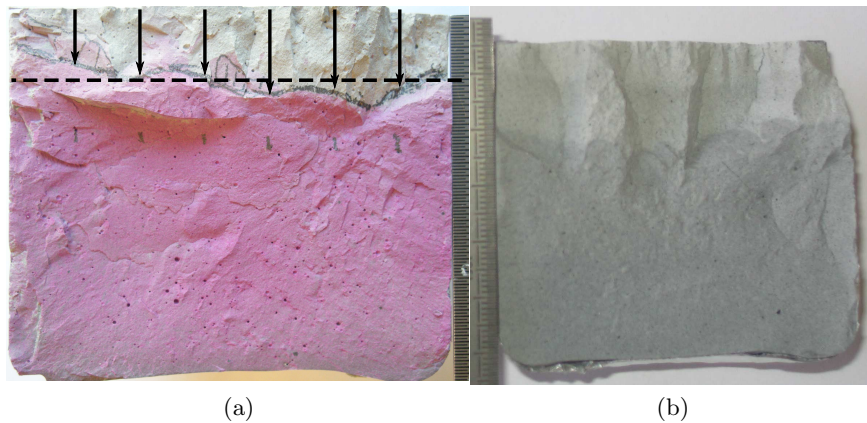
Fig. 2.4 – Exemple de projection de phénolphthaléine à 14 jours de carbonatation accélérée pour un rapport E/C de 0,45. La profondeur de carbonatation est de 1,1 cm (a). Sur la formulation CP60 (b), on distingue nettement le front de carbonatation sans projection de phénolphthaléine à 7 jours à 1,8 cm coïncidant avec le front détecté par projection de phénolphthaléine.
