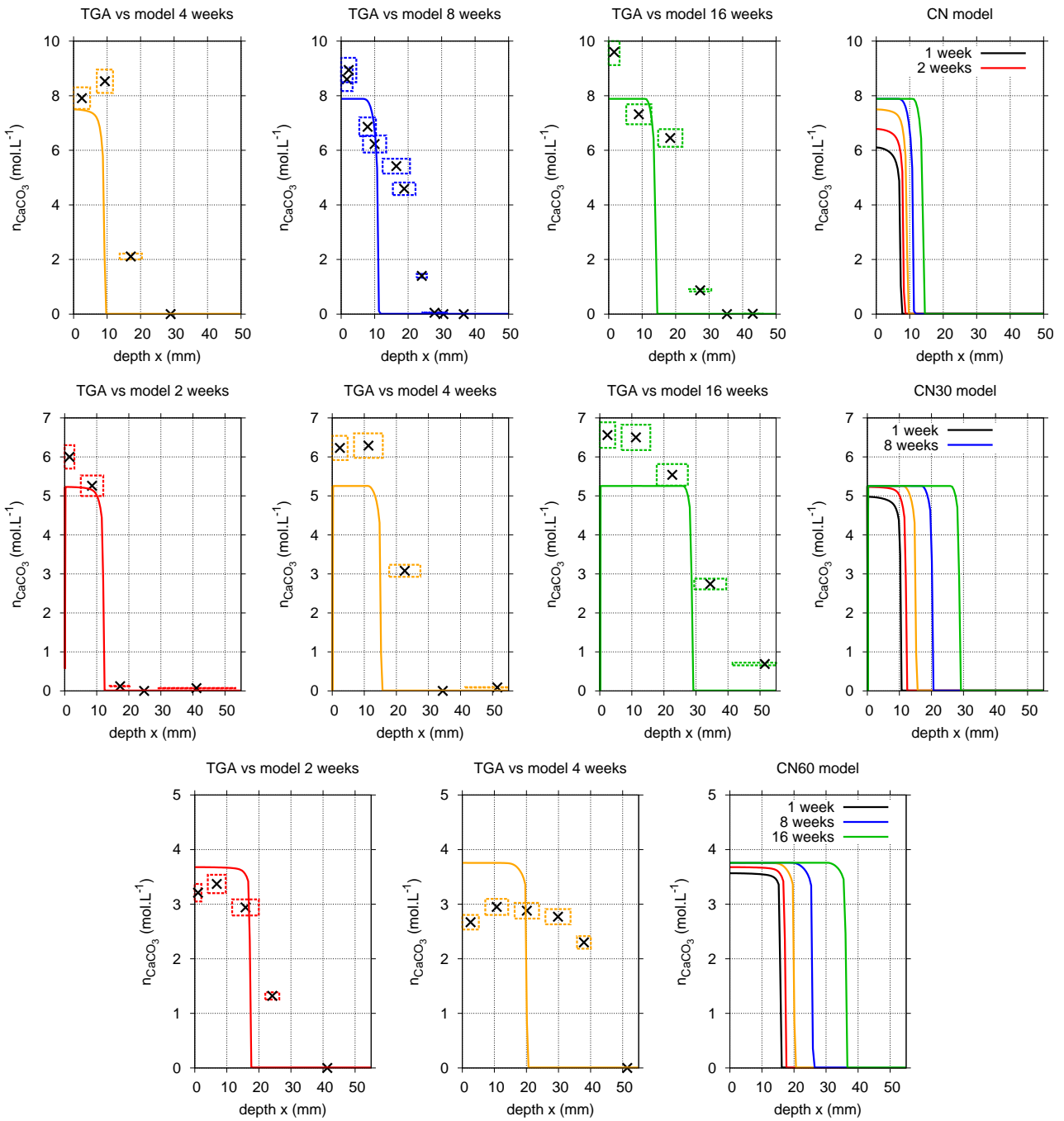
Fig. 6.14 – Profils de teneur en \overline{C\overline{C}} , comparaison des résultats ATG et de modélisation pour CN, CN30 et CN60.
