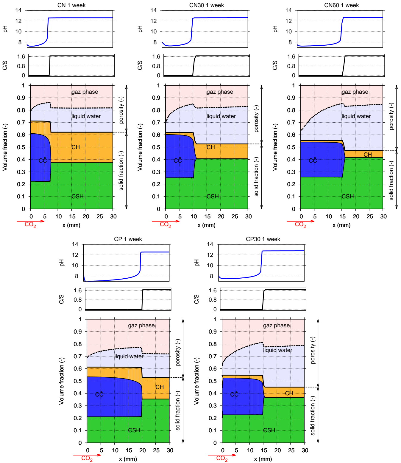
Fig. 6.11 – Aperçu global des résultats de simulation numérique de carbonatation accélérée après 1 semaine. On trace, pour chaque formulation, le profil de pH, le profil de \frac{C}{S} des C-S-H carbonatables, et la distribution volumique adimensionnée des différentes phases (solide, liquide et gaz).
