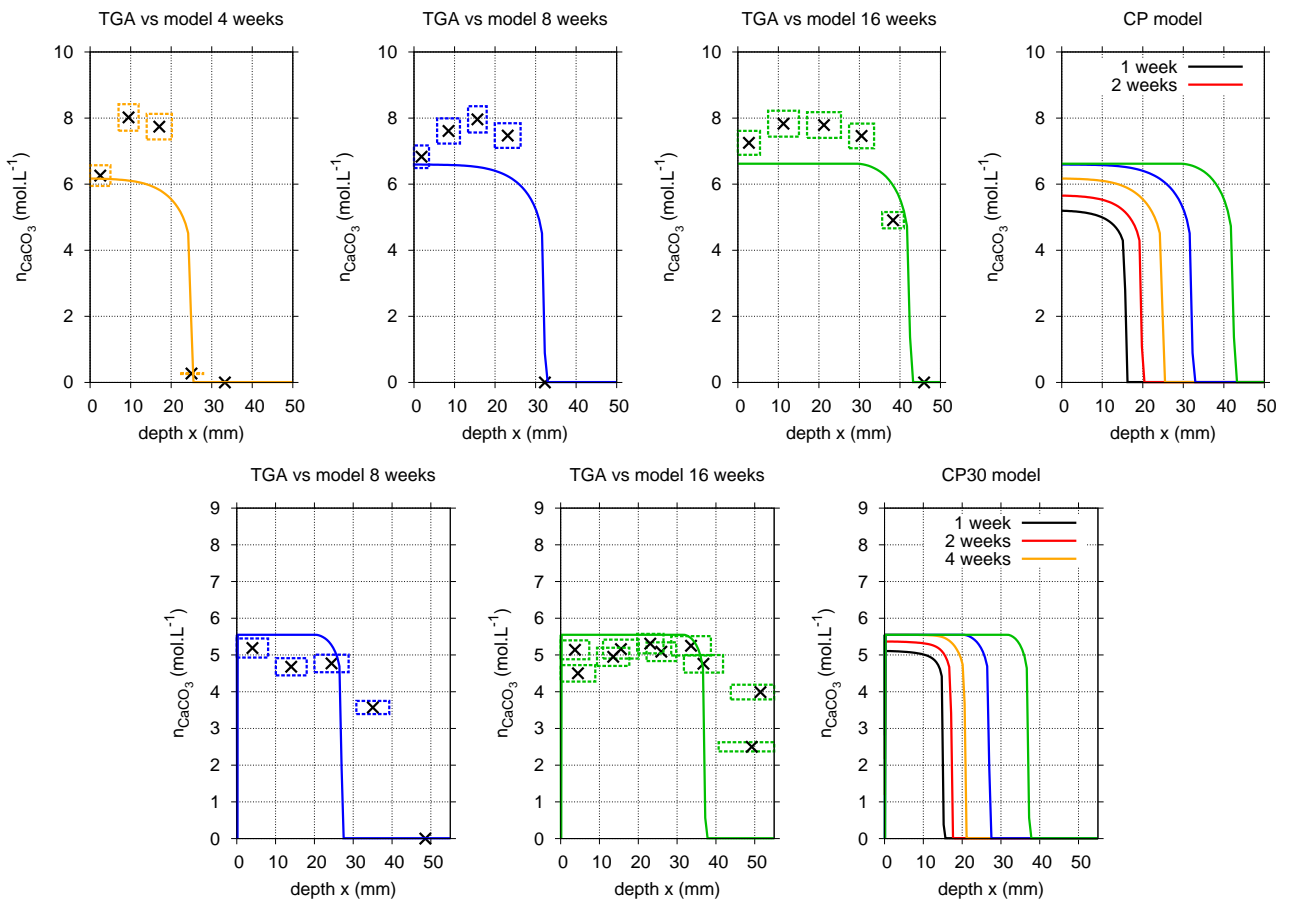
Fig. 6.15 – Profils de teneur en \overline{CC} , comparaison des résultats ATG et de modélisation pour CP et CP30 .
