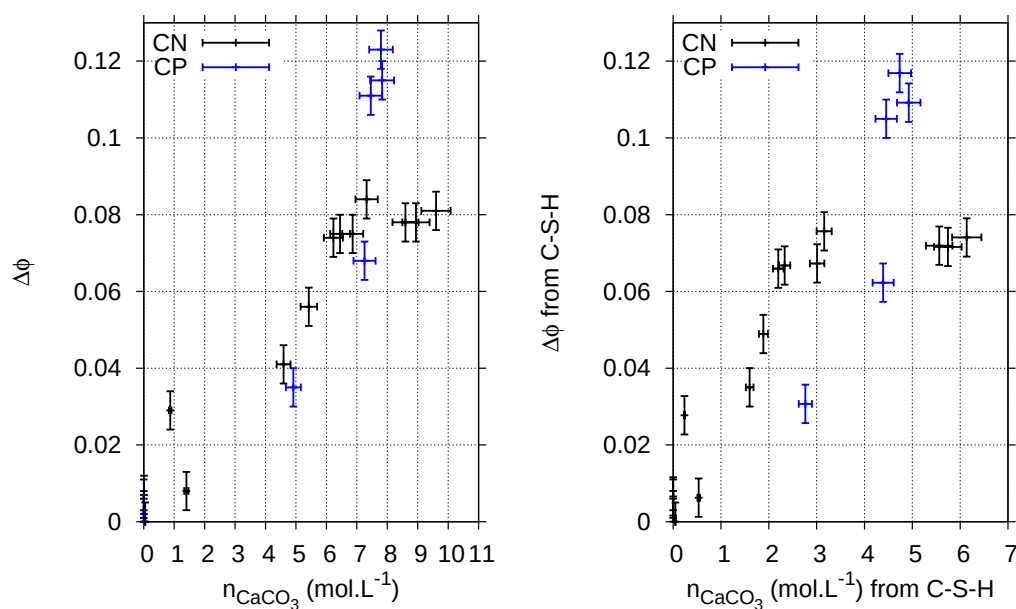
Fig. 3.31 – À gauche, variation de porosité totale en fonction de la quantité totale de \text{C}\bar{\text{C}} . À droite, on a considéré seulement la contribution des C-S-H, que ce soit à la variation de porosité où à la formation de \text{C}\bar{\text{C}} .
