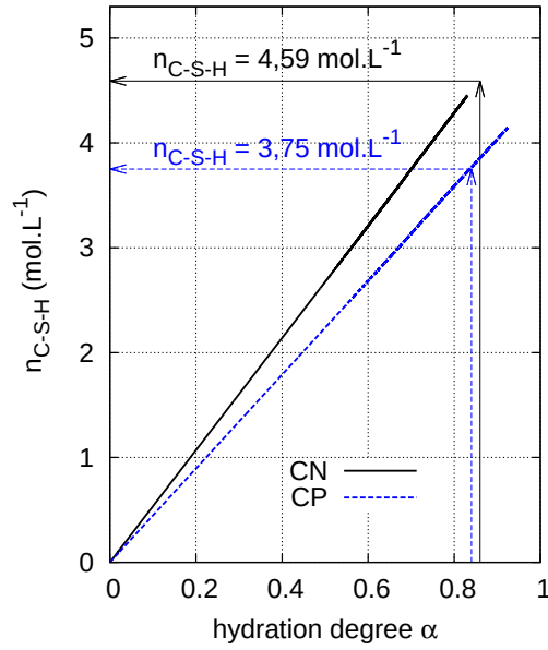
Fig. 3.29 – Évaluation de la quantité initiale de C-S-H calculée à partir du degré d'hydratation, la stœchiométrie choisie pour les C-S-H est C_{1,7}S_1H_{1,5} .
