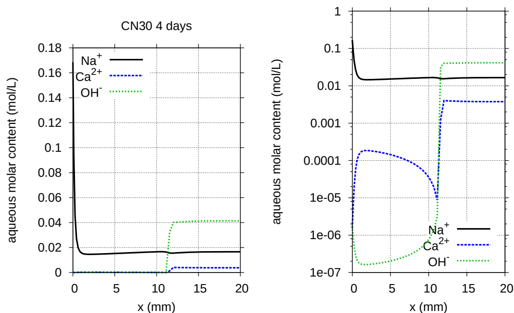
Fig. 6.28 – Profils de concentration en Na^+ , Ca^{2+} et OH^- pour la pâte CN30 à 4 jours. Le profil de K^+ est similaire à celui de Na^+ et n'a pas été représenté pour alléger la figure.
