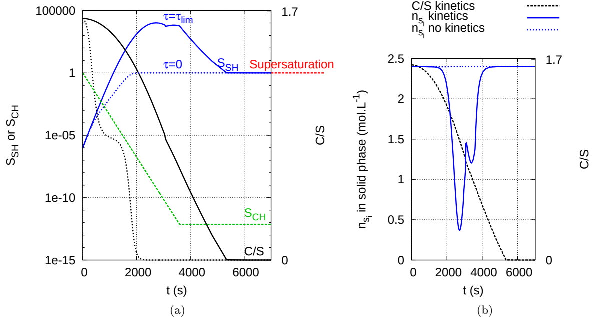
Fig. 6.10 – Comparaison de deux simulations numériques, avec et sans cinétiques sur les C-S-H. On trace S_{\text{CH}} , S_{\text{SH}} et \frac{\text{C}}{\text{S}} en fonction du temps (a). Pour mettre en évidence la dissolution des C-S-H sans précipitation de gel de silice lorsqu'on utilise une cinétique, on trace la quantité de silicium en phase solide (b)
