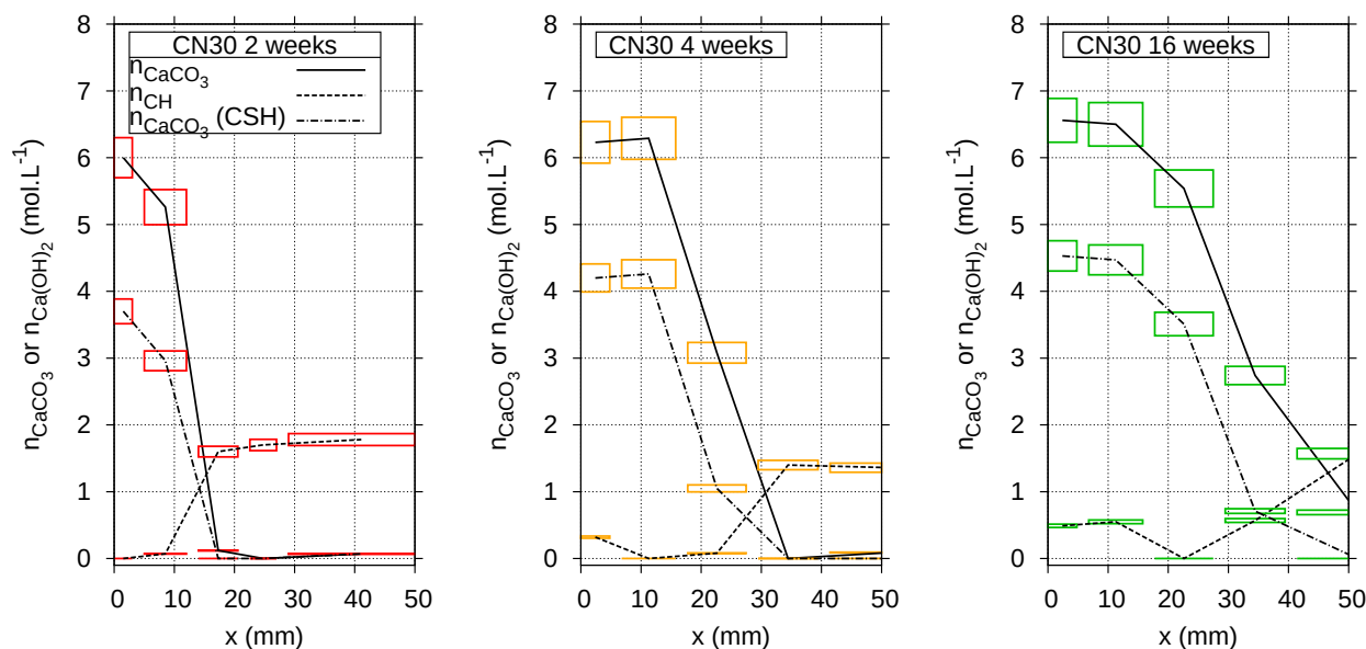
Fig. 4.18 – Profils de teneur en \overline{\text{C}}\overline{\text{C}} totaux, \text{CH} et \overline{\text{C}}\overline{\text{C}} issus de la carbonatation des \text{C-S-H} pour CN30 après 2, 4 et 16 semaines de carbonatation accélérée.
