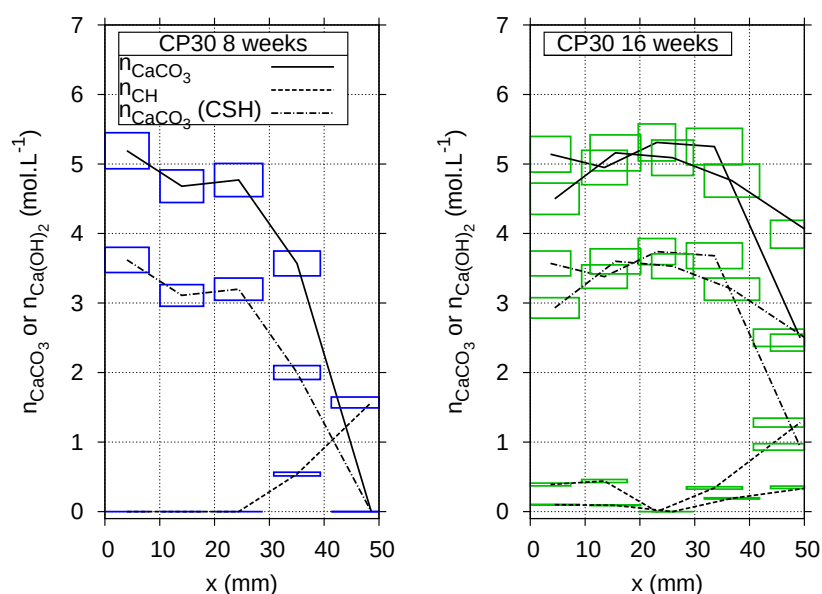
Fig. 4.20 – Profils de teneur en \bar{C}\bar{C} totaux, CH et \bar{C}\bar{C} issus de la carbonatation des C-S-H pour CP30 après 8 et 16 semaines de carbonatation accélérée.
