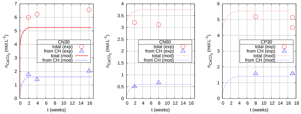
Fig. 6.7 – Teneur en \text{CaCO}_3 après calibration de la cinétique de dissolution de CH pour les pâtes de ciment CN30, CN60 et CP30.
