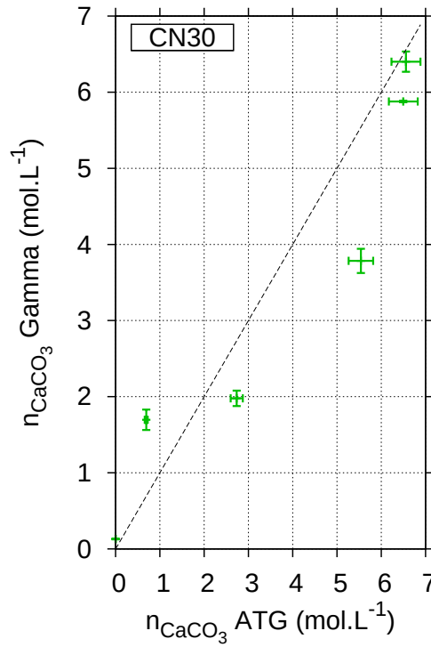
Fig. 4.31 – Comparaison entre les valeurs de n_{\text{C}\overline{\text{C}}} obtenues par la gammadensimétrie et par l'ATG pour CN30 à 16 semaines.
