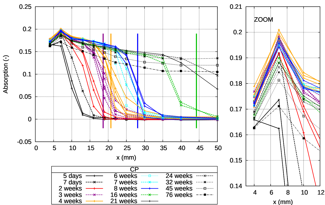
Fig. 3.11 – Profils d'absorption (cf. Eq. 2.4) à différentes échéances de carbonatation accélérée. Compilation de tous les résultats obtenus pour CP. Les profondeurs de carbonatation sont également indiquées par des lignes colorées verticales.
