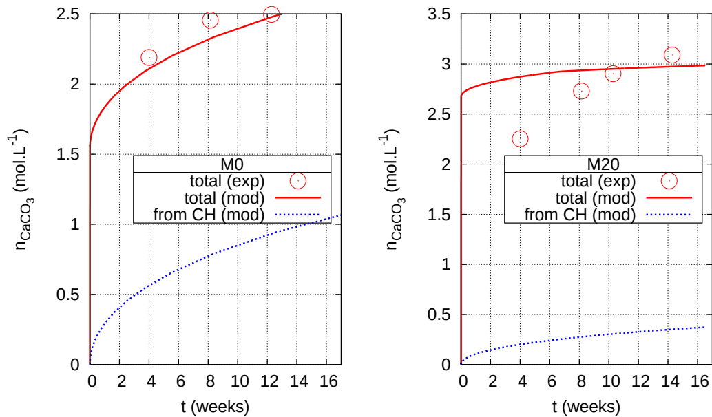
Fig. 6.8 – Teneur en \text{CaCO}_3 après calibration de la cinétique de dissolution de CH pour les mortiers M0 et M20.
