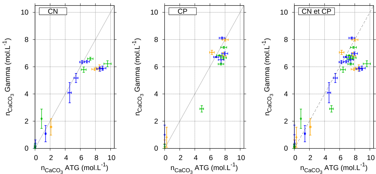
Fig. 3.27 – Comparaison entre les valeurs de n_{\text{CC}} obtenues par gammadensimétrie et par ATG pour CN et CP (méthode décrite Fig. 3.26). On remarque que l'ATG a tendance à conduire à une surestimation.
