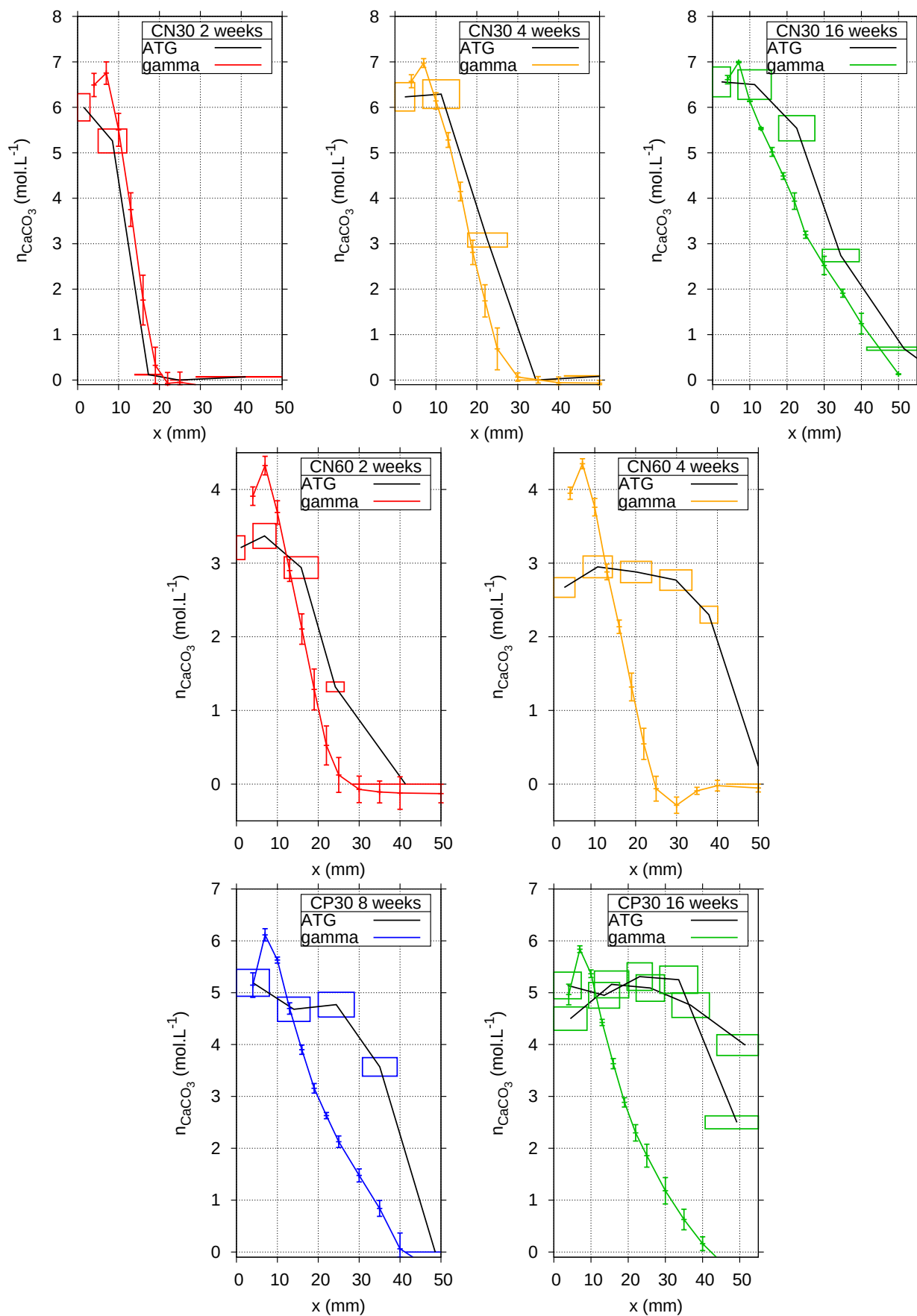
Fig. 4.30 – Comparaison entre les profils de n_{\text{CaCO}_3} obtenus par la gammadensimétrie et par l'ATG pour les pâtes CN30, CN60 et CP30.
