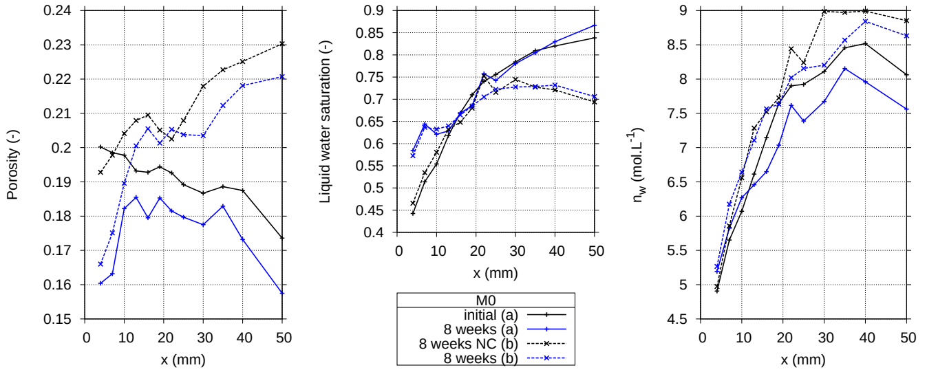
Fig. 3.7 – Mortier M0 : Profils de porosité \phi_\gamma (cf. Eq. 2.5), de saturation en eau liquide S_w (cf. Eq. 2.6) et de teneur en eau n_w (mol.L -1 ) (cf. Eq. 2.7) à l'état initial et après 8 semaines de carbonatation accélérée, ainsi qu'après 8 semaines de séchage dans les mêmes conditions de température et d'humidité que celle de la carbonatation accélérée, mais sans dioxyde de carbone. On observe des résultats différents entre les éprouvettes labellisées (a) et (b) (cf. § 2.4.2)
