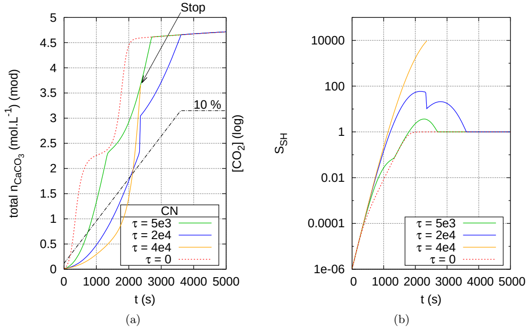
Fig. 6.9 – Calibration de la valeur de \tau Eq. (6.9). On augmente progressivement \tau jusqu'à ce que le modèle numérique s'arrête (a). On illustre en (b) la saturation en gel de silice S_{\text{SH}} au cours des mêmes simulations numériques.
