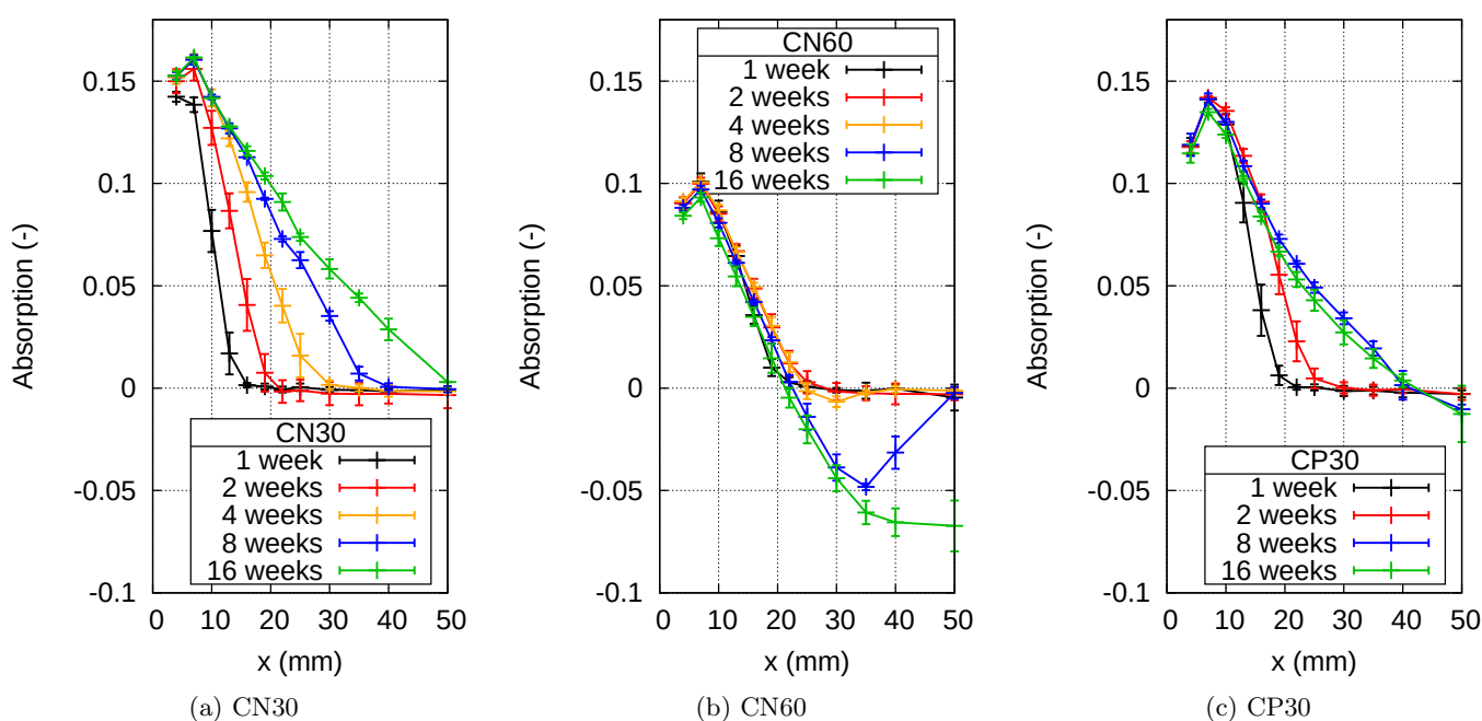
Fig. 4.14 – Profils d'absorption (cf. Eq. 2.4) pour différentes échéances de carbonatation accélérée, moyenne sur plusieurs éprouvettes.
