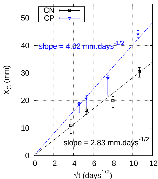
Fig. 3.9 – Évolution de la profondeur de carbonatation mesurée par projection de phénolphthaléine pour les deux formulations CN et CP. Les barres d'erreur présentent le minimum et le maximum des résultats obtenus sur les 12 valeurs mesurées.
