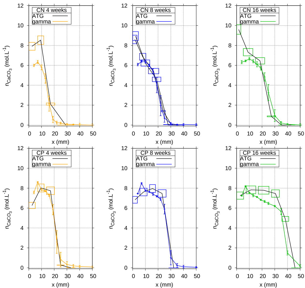
Fig. 3.25 – Comparaison entre les profils de n_{\text{CaCO}_3} obtenus par la gammadensimétrie et par ATG pour les pâtes CN et CP.
