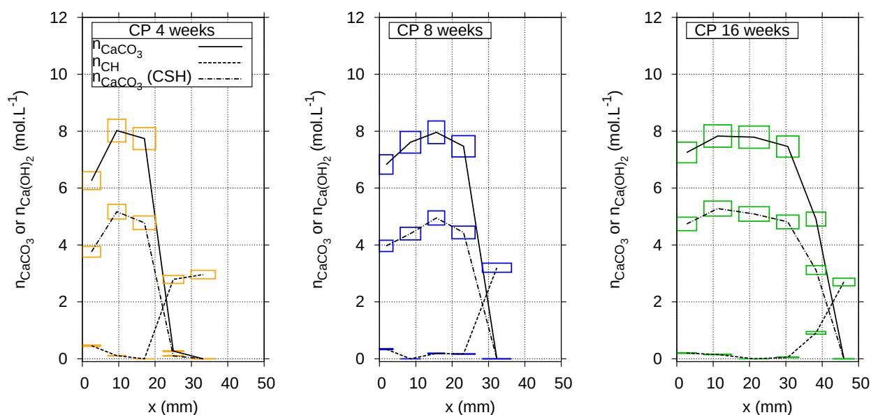
Fig. 3.24 – Profils de teneur en \text{CC} , CH et \text{CC} issus de la carbonatation des C-S-H pour CP après 4, 8 et 16 semaines de carbonatation accélérée.
