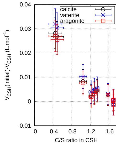
Fig. 3.33 – Influence du volume molaire choisi V_{\text{CC}}^{\text{CSH}} dans l'Eq. (3.12) suivant le choix de la forme de \text{CC} (calcite, aragonite ou vaterite) dans le cas de la pâte CN après 8 semaines. L'influence est négligeable comparée aux incertitudes pour ce calcul.
