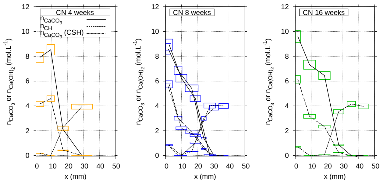
Fig. 3.23 – Profils de teneur en \text{CC} , CH et \text{CC} issus de la carbonatation des C-S-H pour CN après 4, 8 et 16 semaines de carbonatation accélérée.
