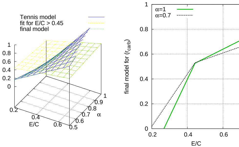
Fig. 6.3 – Tracé de r_{\text{carb}} = n_{\text{CSH}}^{\text{carbonatable}} / n_{\text{CSH}}^{\text{classiques}} en fonction du E/C et du degré d'hydratation.
