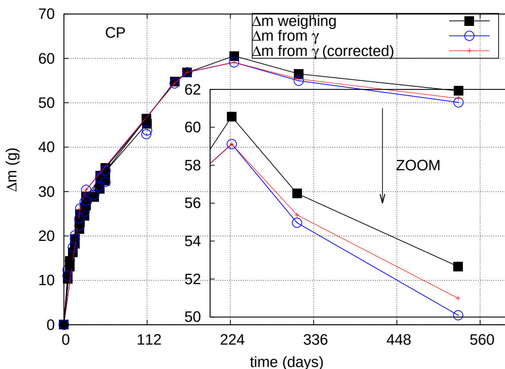
Fig. 3.17 – Gain de masse en fonction du temps pour CP. Le séchage est bien mis en évidence par la perte de masse qui se traduit après la carbonatation complète de l'éprouvette qui a lieu vers 200 jours. On peut effectuer une correction lors de l'intégration des profils de masse volumique en prenant en compte ce séchage de façon plus précise à partir de 224 jours (cf. Eq. 3.4) ce qui permet de mieux se rapprocher de la variation réelle de masse mesurée par pesée.
