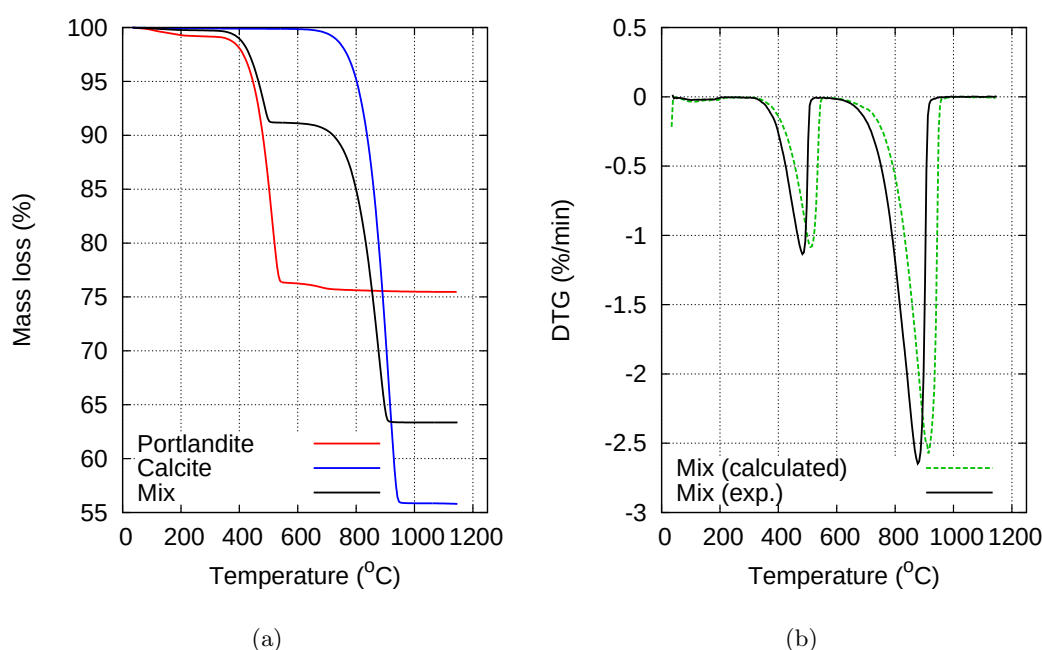
Fig. 2.9 – ATG sur portlandite, calcite et un mélange des deux (a). DTG sur un mélange de calcite et portlandite, résultat expérimental et résultat calculé à partir d'une combinaison linéaire des résultats sur corps purs (b).
