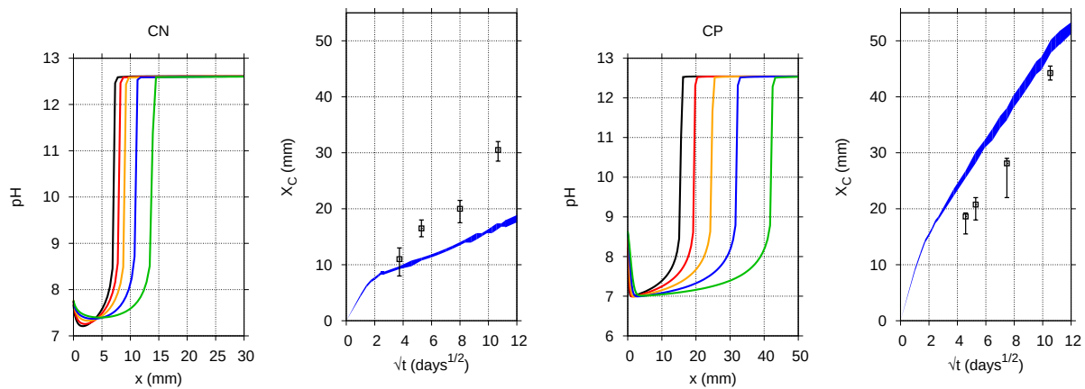
Fig. 6.23 – Pâtes CN et CP, profils de pH et profondeur de carbonatation associée ( X_c en fonction de \sqrt{t} ).
