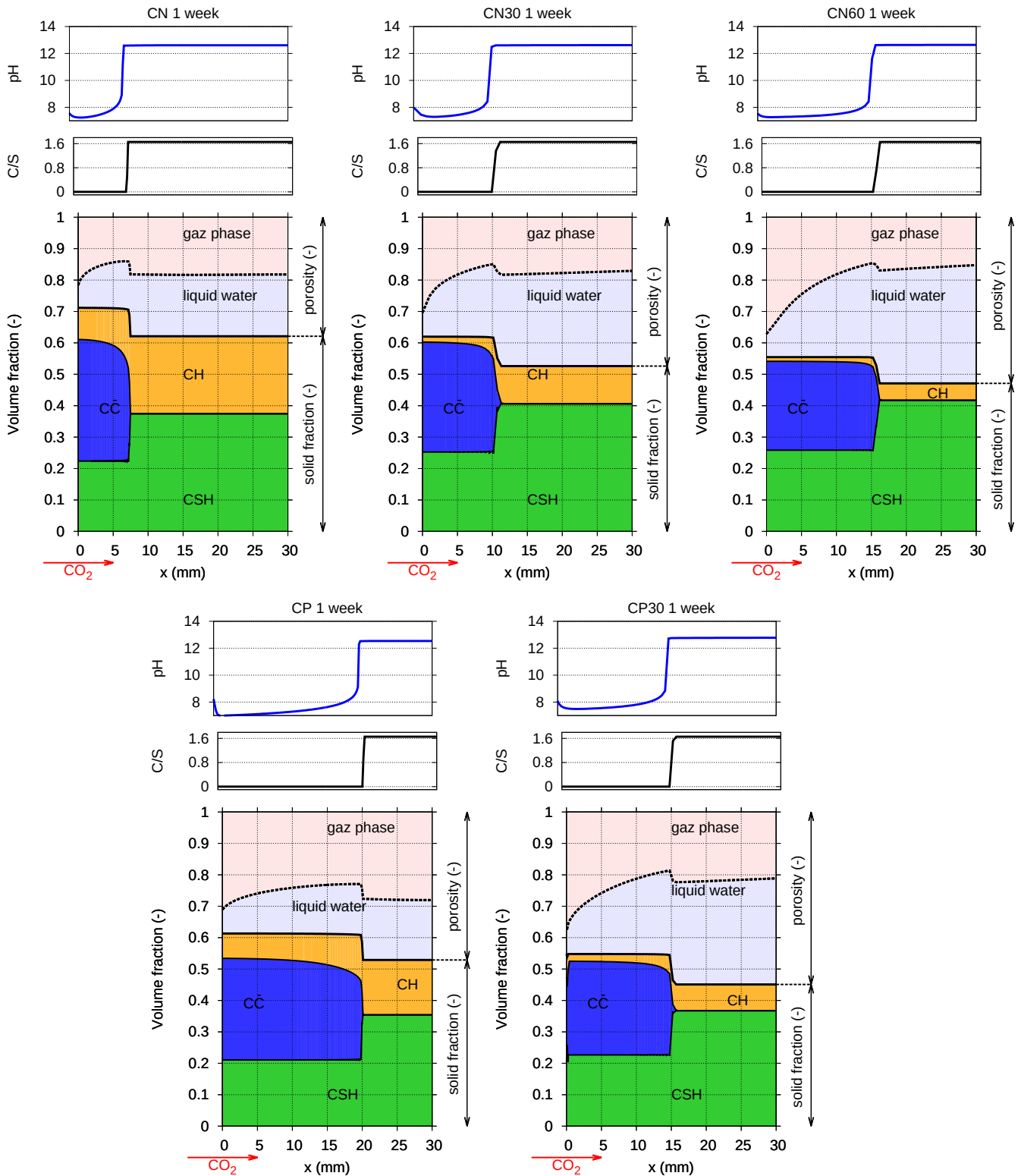
Fig. 6.11 – Aperçu global des résultats de simulation numérique de carbonatation accélérée après 1 semaine. On trace, pour chaque formulation, le profil de \text{pH} , le profil de \frac{\text{C}}{\text{S}} des C-S-H carbonatables, et la distribution volumique adimensionnée des différentes phases (solide, liquide et gaz).
