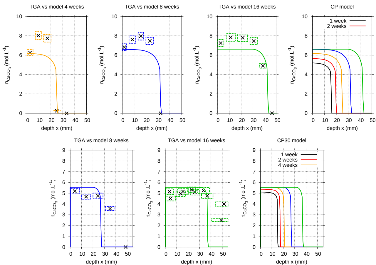
Fig. 6.15 – Profils de teneur en \text{CaCO}_3 , comparaison des résultats ATG et de modélisation pour CP et CP30.
