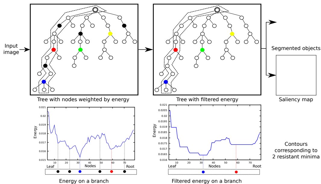
Figure 5: Un exemple de détection d’objets. Dans les arbres, les cercles pleins représentent les minima locaux, et les cercles pleins colorisés, les minima locaux restant après filtrage. En bas, les courbes montrent l’évolution de l’attribut, avant et après filtrage, le long de la branche entourée dans l’arbre. En haut à droite : les objets significatifs détectés (contours colorisés) et une hiérarchie de détection d’objets représentée sous la forme d’une carte de saillance.
