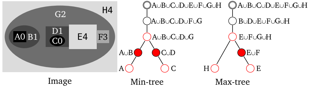
Figure 3: Une image synthétique, son Min-tree (au milieu) et son Max-tree (à droite). Les régions critiques sont représentées par des cercles rouges : ce sont des nœuds ayant plus d'un enfant et les feuilles. Les TBMRs sont les régions correspondants aux nœuds remplis en rouge.
