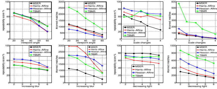
Figure 4: Le score de répétabilité (à gauche) et le nombre de correspondances (à droite) pour les séquences Wall , Bark , Trees , Leuven (de haut en bas, et de gauche à droite).
