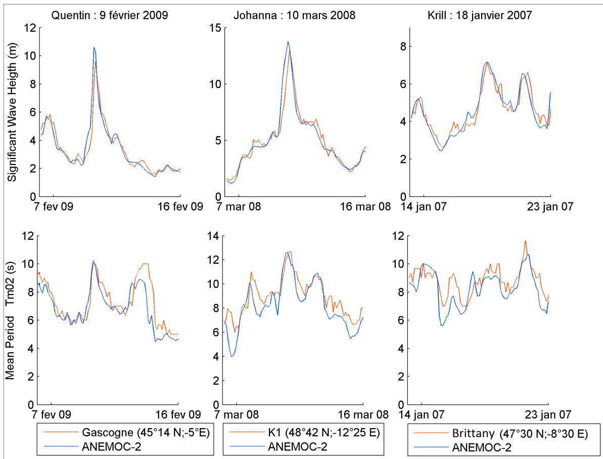
Figure 3.26: Comparaison des observations houlographiques avec les résultats d'ANEMOC-2 pour 3 tempêtes : Quentin, Johanna et Krill.
