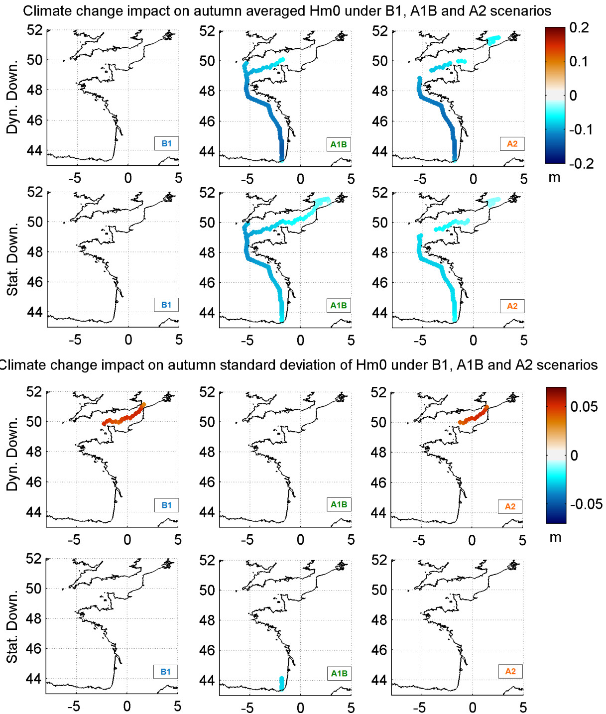
Figure 8.17: Comparaison de l'impact du changement climatique statistiquement significatif au sens du test de Welsh ou Fisher sur la moyenne et la variabilité de H_{m0} en automne suite à l'application des descentes d'échelle dynamique et statistique des scénarios B1, A1B et A2 d'ARPEGE-CLIMAT.
