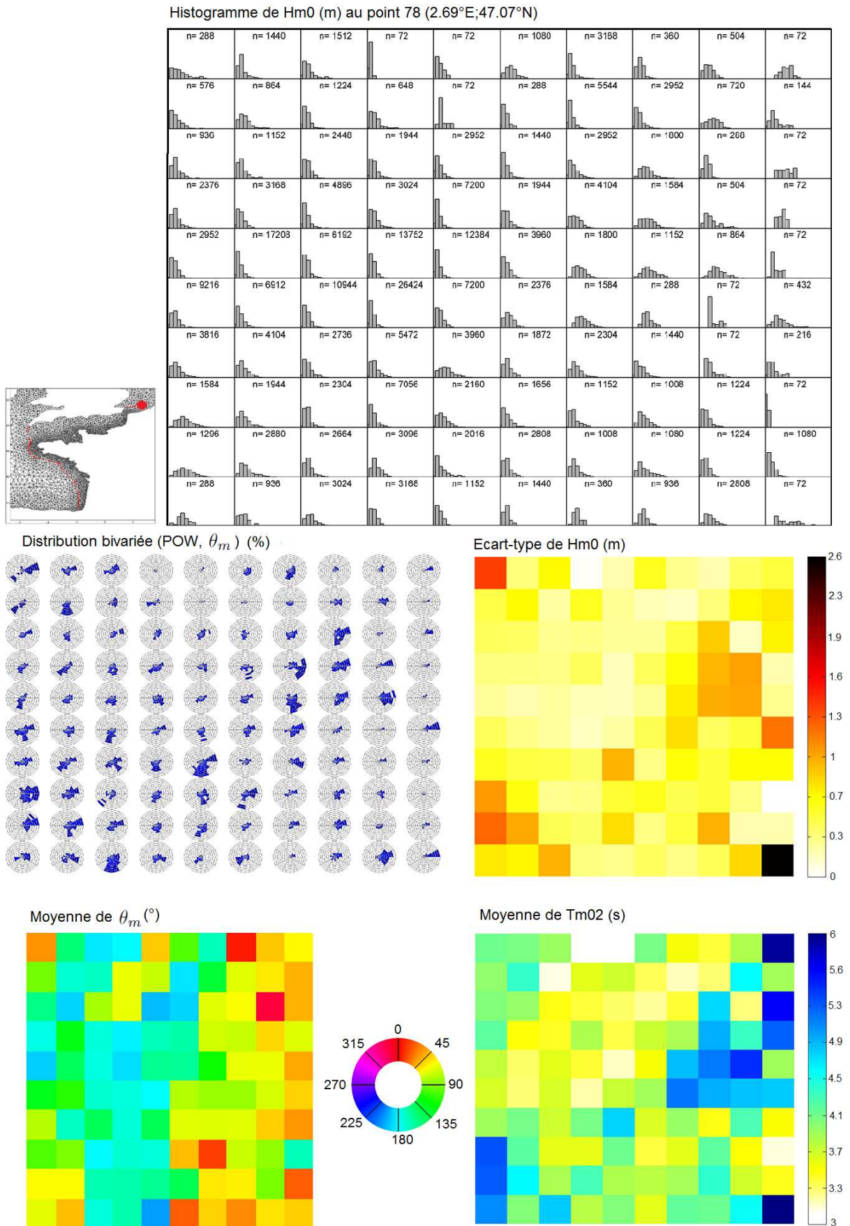
Figure 4.11: Classification des variables predictands : histogramme et écart-type de H_{m0} , distributions bivarée ( POW, \theta_m ) et moyennes de \theta_m et de T_{m02} au nœud 78 à l'approche de la Mer du Nord (2.69°E; 47.07°N).
