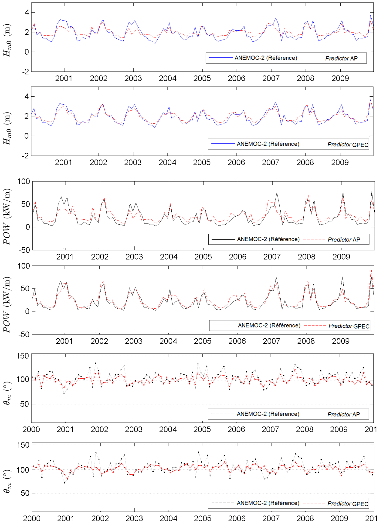
Figure 4.14: Projections des moyennes mensuelles des hauteurs significatives H_{m0} , du flux d'énergie moyen POW et de la direction moyennes \theta_m des vagues au point de validation n°2 ( 45.54^{\circ}N ; 2.05^{\circ}W ) pour les predictors AP et GPEC sur la période 2000-2009, et comparaison avec les résultats d'ANEMOC-2 au vu de la validation du modèle de régression statistique.
