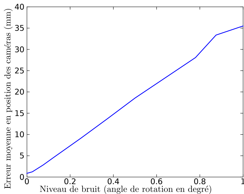
FIGURE 6.17 – Évaluation de la précision d'estimation moyenne de la pose des caméras, en mm, calculée en fonction du bruit introduit sur les rotations globales.
