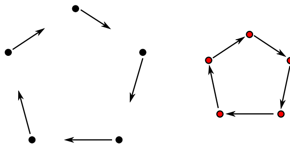
FIGURE 6.15 – A gauche les vecteurs translations \mathbf{t}_{ij} normé initiaux et les translations globales T_i . A droite le résultat identifié par notre méthode. Ce cas parfait de 5 caméras le long d'un cercle à distance régulière identifie une solution avec des vecteurs \lambda_{ij} de valeur 1. Une solution valide au problème a été identifiée à une échelle près de la vérité terrain.
