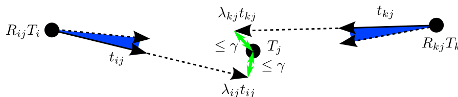
FIGURE 6.14 – Notre approche minimise des distances euclidiennes (distance verte) tandis que SIM et HARTLEY (2006) minimisent les erreurs angulaires indiquées en bleu.
