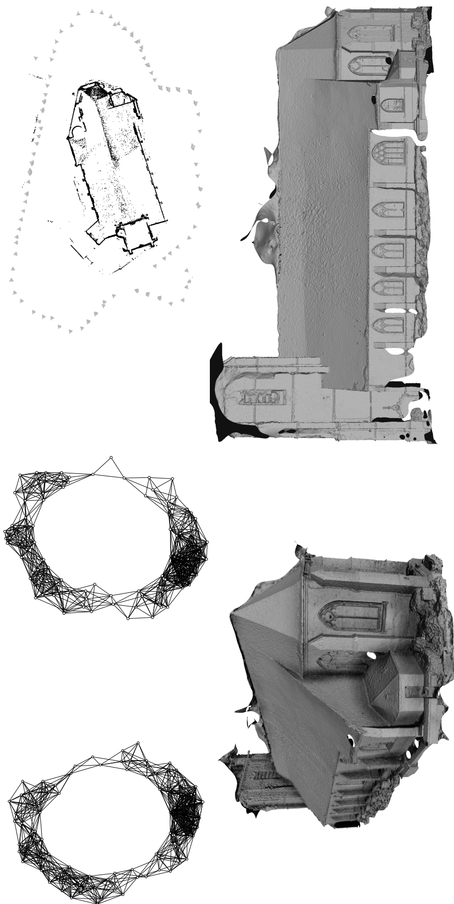
FIGURE 6.23 – AultP106. De gauche à droite et de haut et de bas : Le graph épipolaire G_E avant puis après inférence : G_{\mathcal{R}} . La structure et poses des caméras obtenues après calibration externe. Le maillage reconstruit à partir de notre calibration externe de l'église d'Ault. Temps de calibration (méthode globale : 20 min, méthode séquentielle : 3.5 h).
