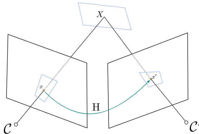
FIGURE 3.2 – La relation homographique établie une relation point à point entre les images d'une surface plane dans plans images.
