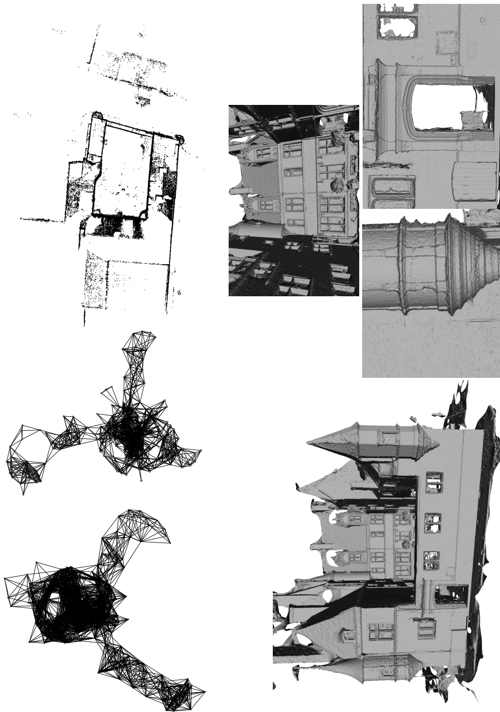
FIGURE 6.24 – HotelCujasP182. De gauche à droite et de haut en bas : Le graph épipolaire G_E avant puis après inférence : G_R . La structure obtenue après calibration externe. Vue avec recul et sur des détails du bâtiment sur le maillage reconstruit de l'hôtel Cujas (Bourges) à partir de notre calibration externe. Temps de calibration (méthode globale : 15 min, méthode séquentielle : 2 h).
