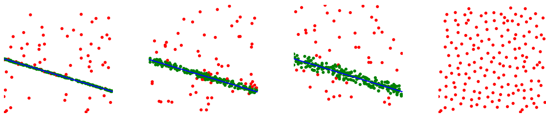
FIGURE 4.2 – Comportement d' AC-RANSAC pour une ligne ou un bruit gaussien de plus en plus grand est ajouté. En vert les données validées a contrario en rouge les données rejetées et en bleu le modèle identifié. On note, à droite, qu'en présence de bruit pur AC-RANSAC n'identifie aucun modèle, RANSAC aurait lui retourné une fausse hypothèse.
