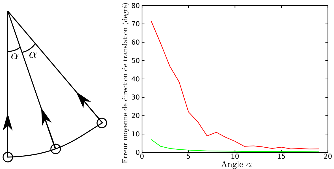
FIGURE 6.11 – A gauche la configuration de caméra utilisé pour l'expérience. A droite les erreurs moyennes de directions de translations pour des matrices essentielles (rouge) et pour notre tenseur tri-focal réduit (vert) en fonction de l'angle inter-caméra \alpha .
