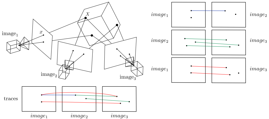
FIGURE 3.16 – Dans une série d’images non ordonnées ( image_1, image_2, image_3 ), des correspondances sont identifiées par par paire d’images (droite). Relier ces correspondances si elles partagent des points en commun permet d’identifier les traces (bas gauche). Note : L’analyse d’une série de paires 1 \rightarrow 2, 2 \rightarrow 3, 1 \rightarrow 3 permet de créer une correspondance entre l’image 1 et 3 qui ne serait pas identifiée par une analyse en séquence : 1 \rightarrow 2 \rightarrow 3 .
