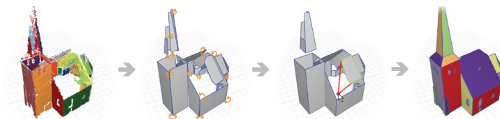
FIGURE 1.10 – Un aperçu de la chaîne semi-automatique de modélisation O-Snap. De gauche à droite : Un nuage de point bruité et incomplet est décomposé en une sélection de plans. Des relations d’adjacences de polygones proches sont identifiées afin de les connecter et de raffiner le modèle. L’utilisateur guide ensuite le processus automatique en rajoutant manuellement des relations d’adjacences. Un modèle à faible nombre de polygones représentant le nuage de point 3D peut ainsi être reconstruit.
