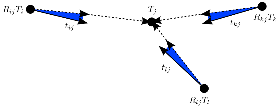
FIGURE 6.5 – Un ensemble de translations globales \{T_i\}_i sont recherchées en fonction des directions de translations relatives \mathbf{t}_{ij} par minimisation de la plus grande des erreurs angulaires observées (angles bleus). Pour lisibilité seules les contraintes que portent T_j sont représentées.
