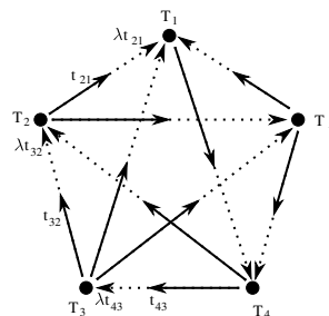
FIGURE 6.4 – Etant donné un ensemble de directions de translations relatives \mathbf{t}_{ij} , les positions globales T_i des caméras sont recherchées.
