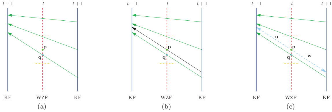
Figure 3: Les différents passage pour la méthode d'interpolation de DISCOVER. Le but est d'estimer le bloc centré en \mathbf{p} . Soit \mathbf{q} le point d'intersection le plus proche entre le champs de mouvement estimé et la TWZ I_t (a). Le vecteur en \mathbf{q} est déplacé afin qu'il passe en \mathbf{p} (b). Après le vecteur est scissionné (c).
