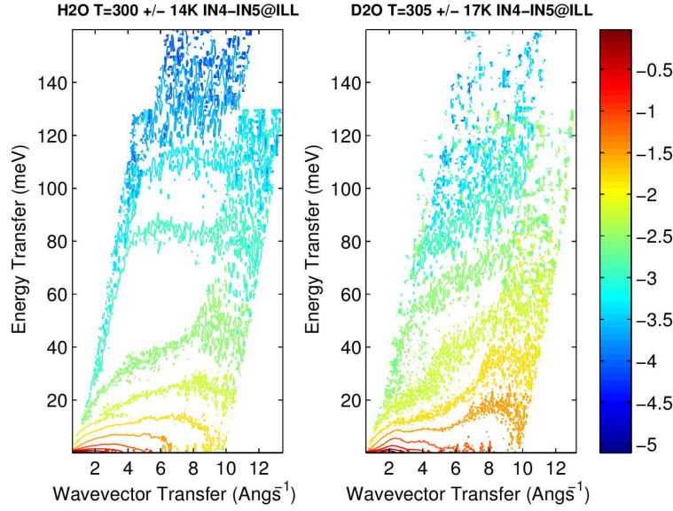
FIGURE 4.6 – Fonction \log_{10}(S_T^{sym}(q, \omega)) extraite des données expérimentales, pour l’eau légère (à gauche) et l’eau lourde (à droite)
