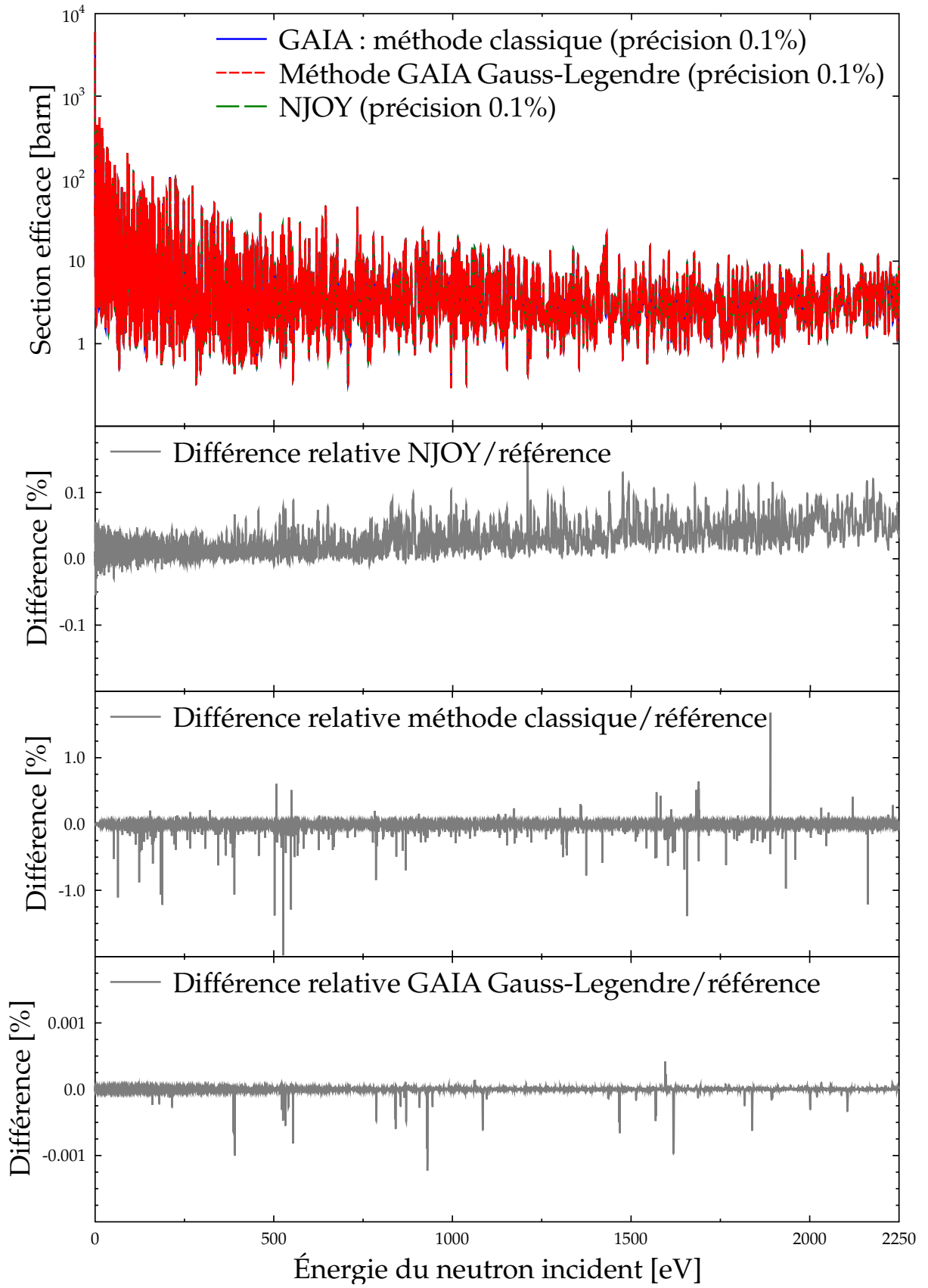
FIGURE 3.5 – Section de capture de ^{235}\text{U} , calculée à T = 293.6 K avec les deux méthodes et NJOY, pour une précision de 0.1 %
