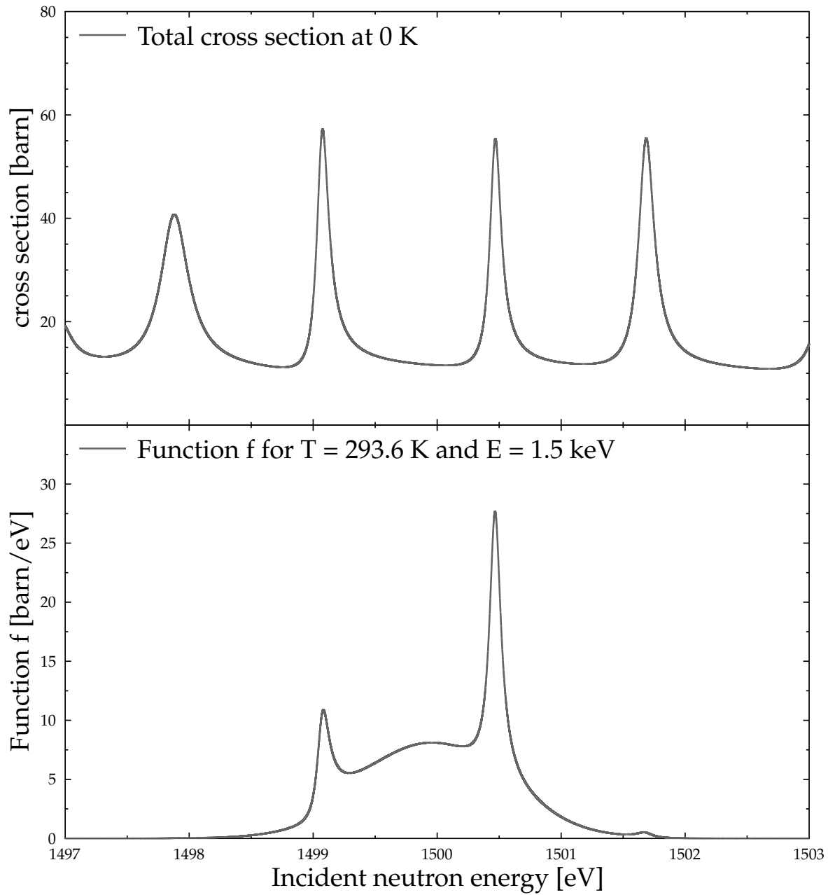
FIGURE 3.4 – Function f pour la section totale de ^{238}\text{U} , pour T = 293.6 K et E = 1.5 keV
