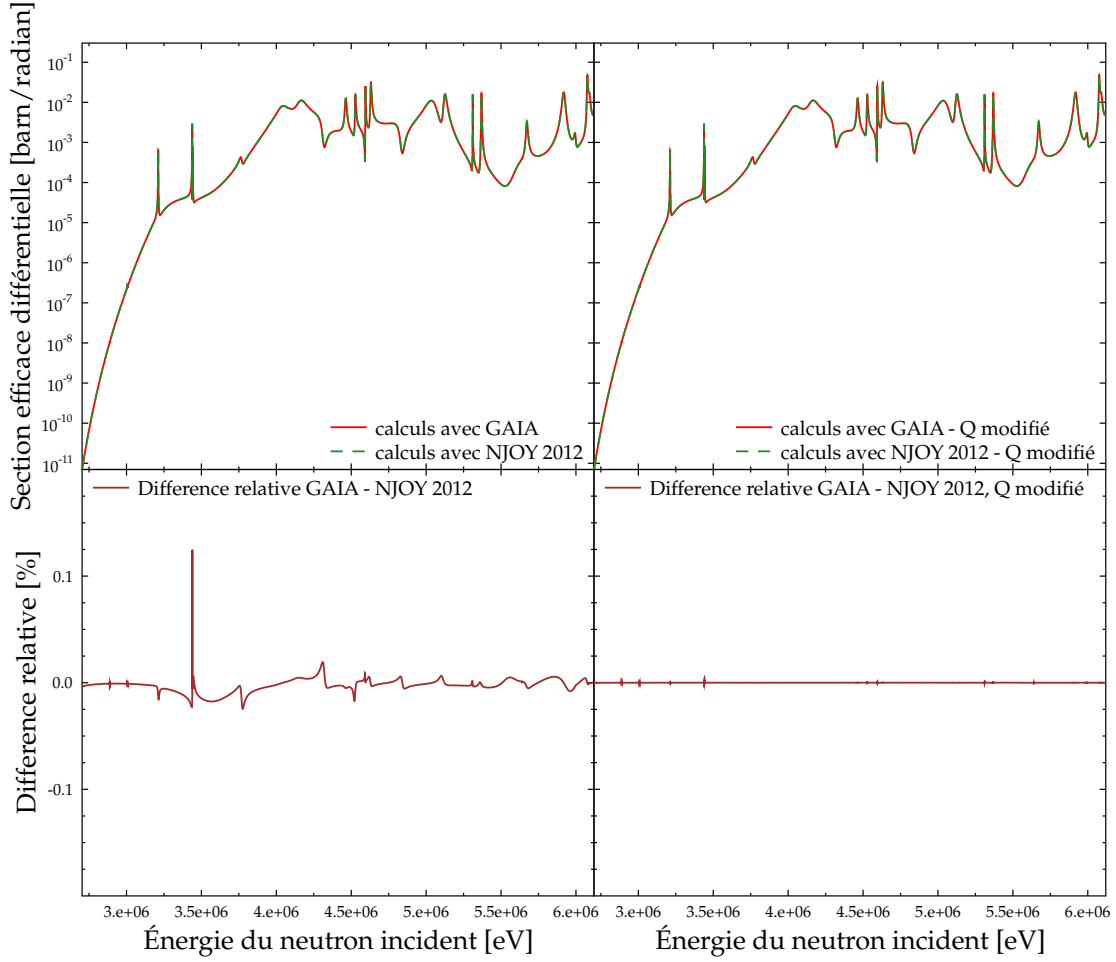
FIGURE 4.2 – Section efficace différentielle ( n, \alpha ) à 0 K du ^{16}\text{O} pour \theta = 60^\circ , reconstruite par GAIA et NJOY 2012, à gauche avec les valeurs de Q originelles et à droite avec les valeurs homogénéisées.
