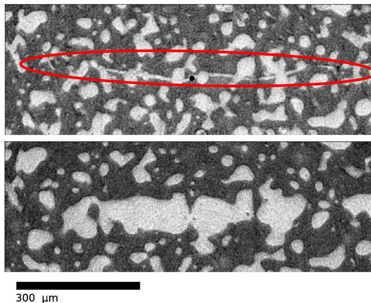
FIGURE 3.11 – Coupe tomographique, juste après une trempe suivie d’une remise à haute température, au début de l’expérience visi02 (haut). La phase riche en baryum est venue occuper préférentiellement la zone où une fissure s’était formée pendant la trempe (entourée en rouge). Cet événement a profondément influencé la suite du mûrissement (bas).
