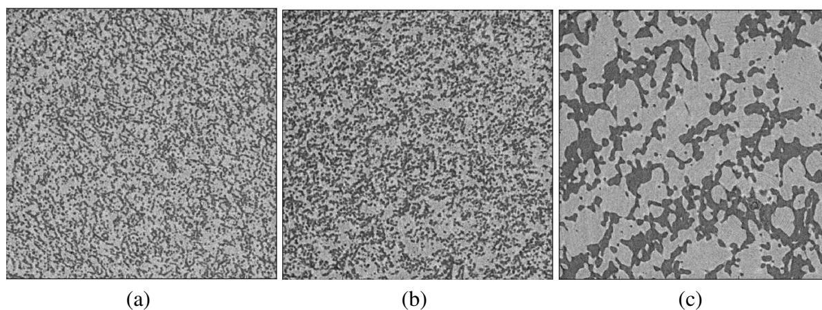
FIGURE A.3 – vbap_s1 . Coupes partielles (largeur 500 \mu\text{m} ) d'images reconstruites. (a) Après 20 minutes à 1050 ^{\circ}\text{C} , (b) après 60 minutes à 1050 ^{\circ}\text{C} , (c) après après 120 minutes à 1050 ^{\circ}\text{C} . Fraction volumique \Phi \approx 0.6 .
