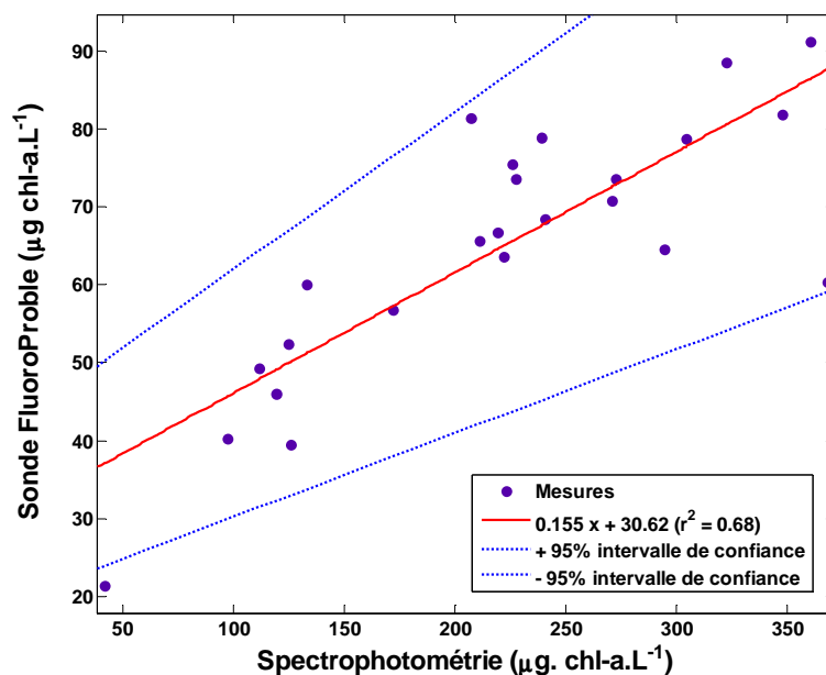
Figure 8.7 : Régression linéaire entre les mesures de la sonde Fluoroprobe (< 100 µg chl-a.L -1 ) et les mesures spectrophotométriques
