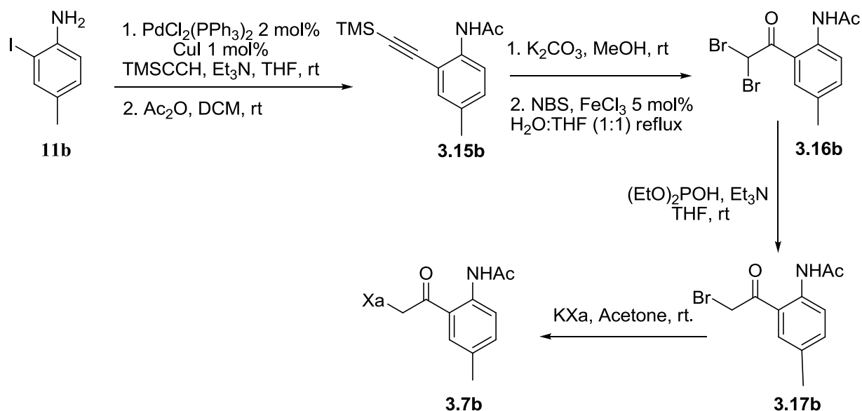
Scheme II-B9
