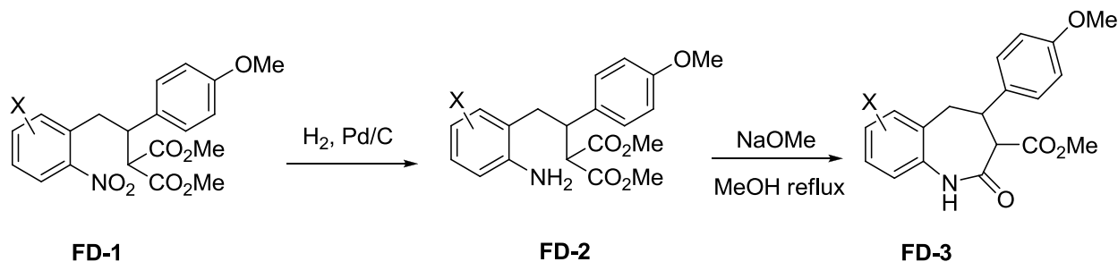
Scheme I-15
