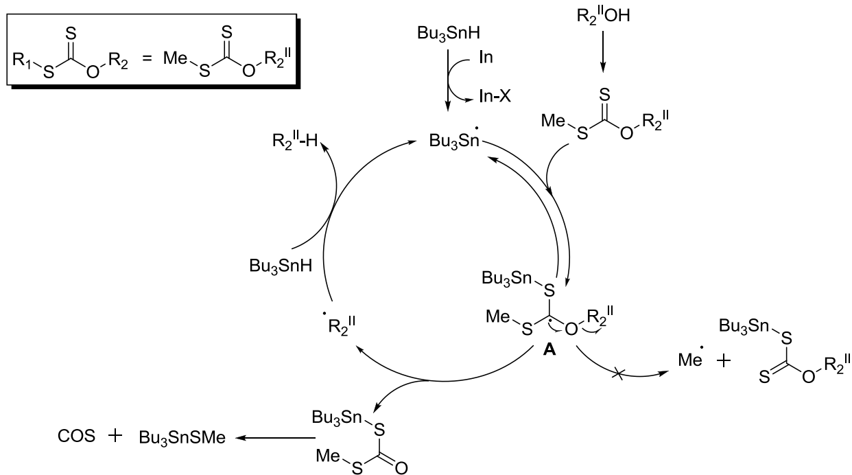
Scheme II-4
