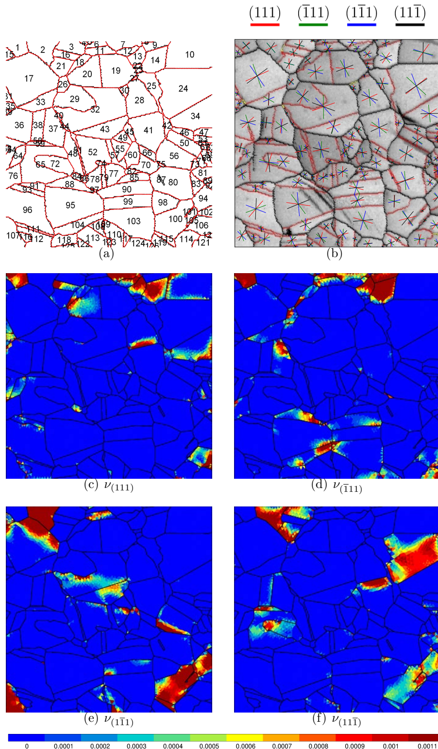
FIGURE IV.17 – Résultats de la région n°2 de l'éprouvette sollicitée en flexion plane : représentation (a) de la numérotation des grains, (b) des traces des plans de glissement et de la somme des glissements plastiques cumulés dans le plan : (c) (111), (d) ( \bar{1}\bar{1}1 ), (e) ( 1\bar{1}\bar{1} ) et (f) ( \bar{1}1\bar{1} ).
