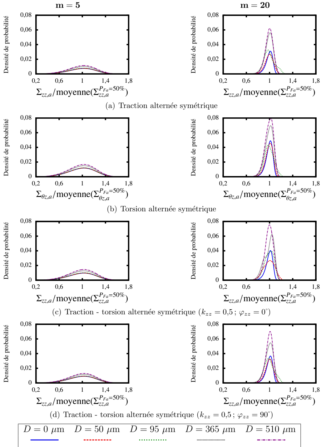
FIGURE V.17 – Distributions complètes de la limite de fatigue macroscopique \Sigma_{ij,a} décrite par la densité de probabilité f_{moy}(\Sigma_{ij,a}) obtenues avec un comportement des grains élastique cubique, pour différentes valeurs du paramètre de forme m , sollicitations et diamètres de défaut D .
