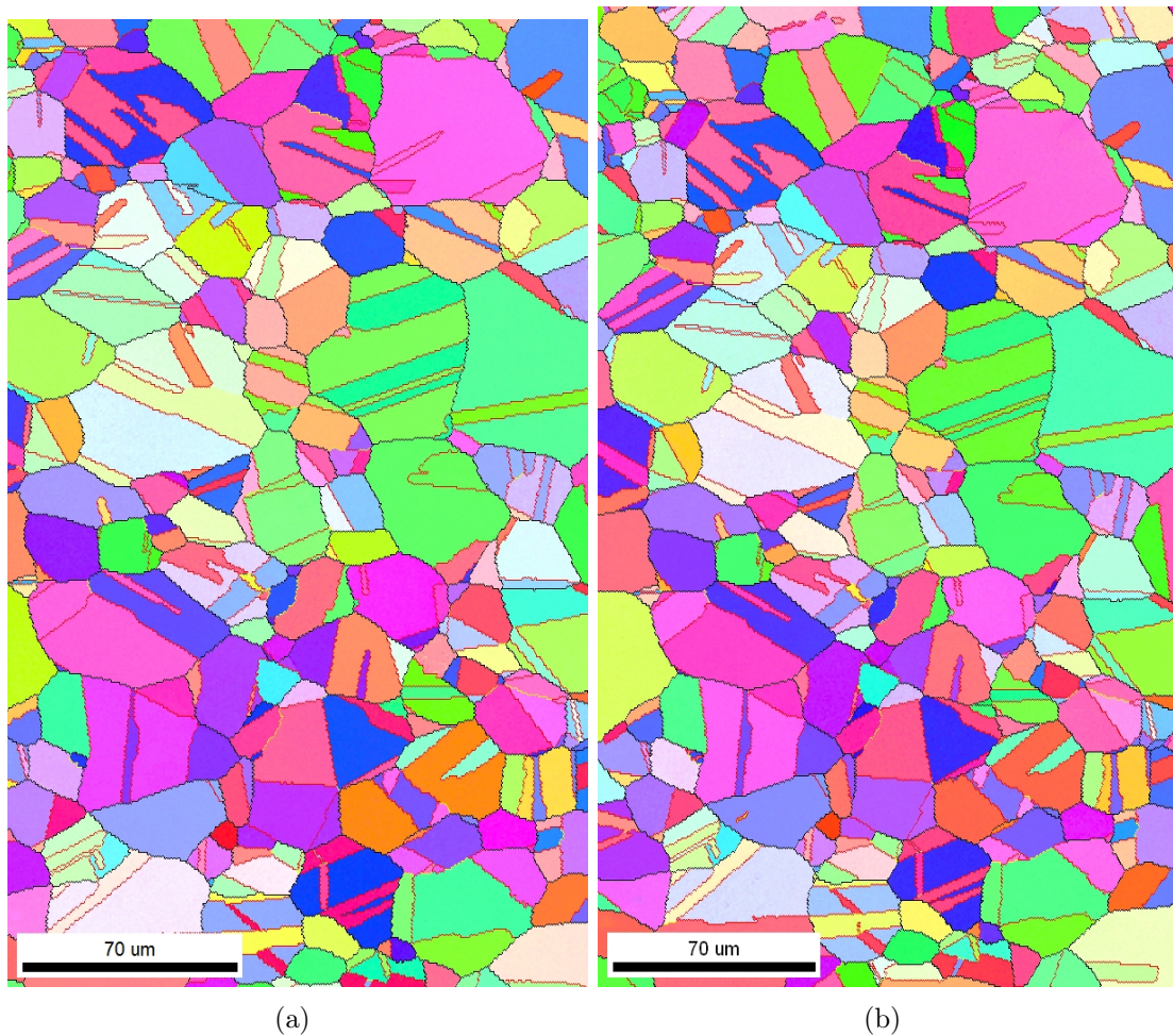
FIGURE E.1 – Cartographies d'orientation en figure de pôle inverse de la région n° 1 de l'éprouvette sollicitée en flexion plane : (a) avant sollicitation et (b) après sollicitation.
