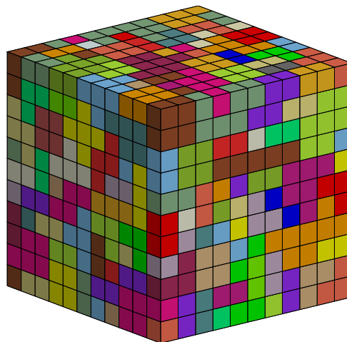
FIGURE III.16 – Maillage périodique d'un agrégat polycristallin de 300 grains discrétisés par 1331 éléments hexaédriques.
