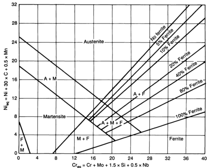
FIGURE I.1 – Diagramme de Schaeffler [1] rapporté par [2].
