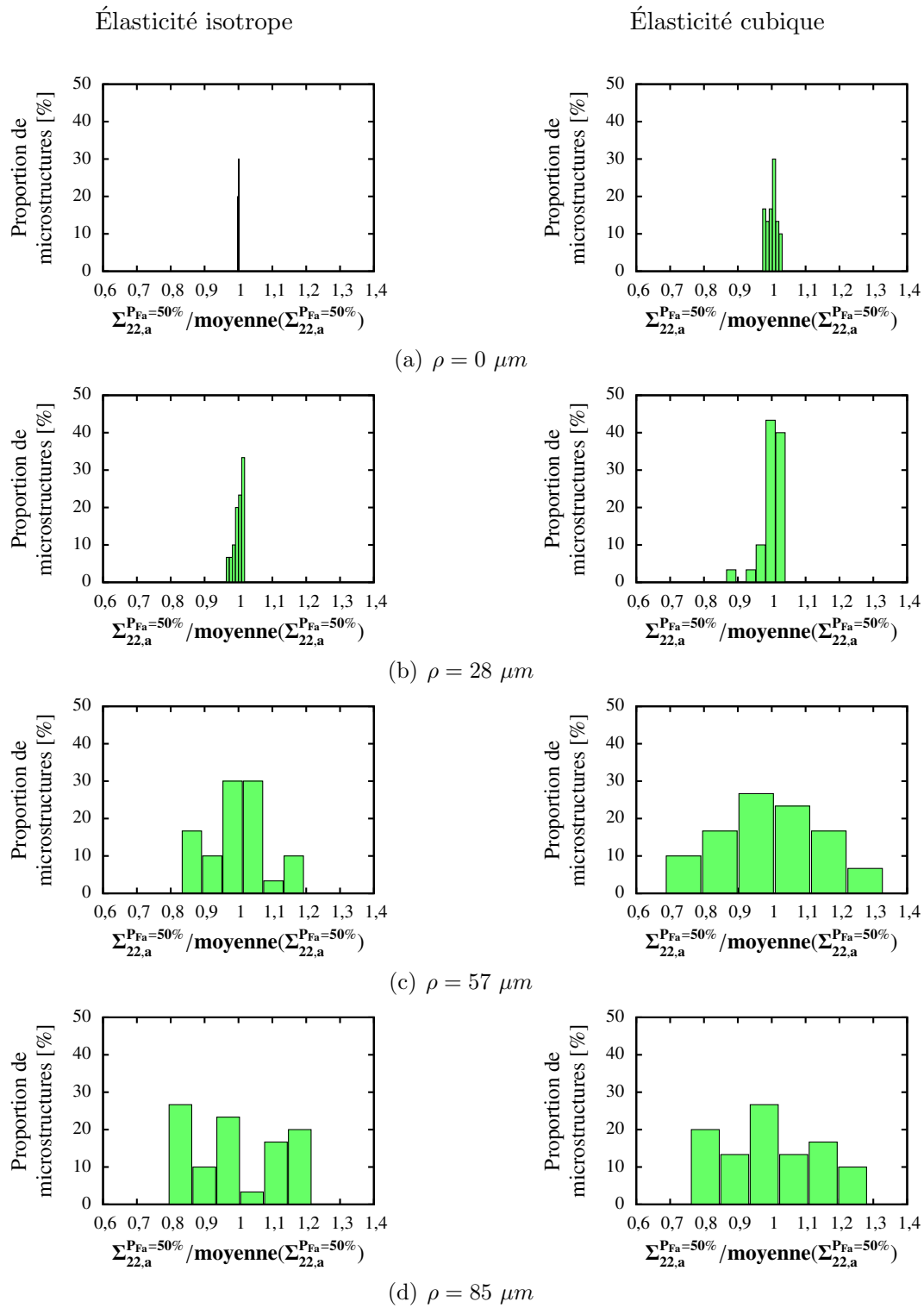
FIGURE II.33 – Histogrammes des limites de fatigue à P_{Fa} = 50\% des microstructures trouées sollicitées en traction alternée symétrique pour différents rayons de trou \rho et pour chaque modèle de comportement élastique.
