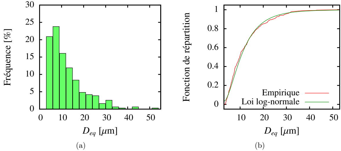
FIGURE IV.7 – Distribution de la taille de grain D_{eq} empirique : (a) densité empirique et (b) fonctions de répartition empirique et de loi de probabilité log-normale.
