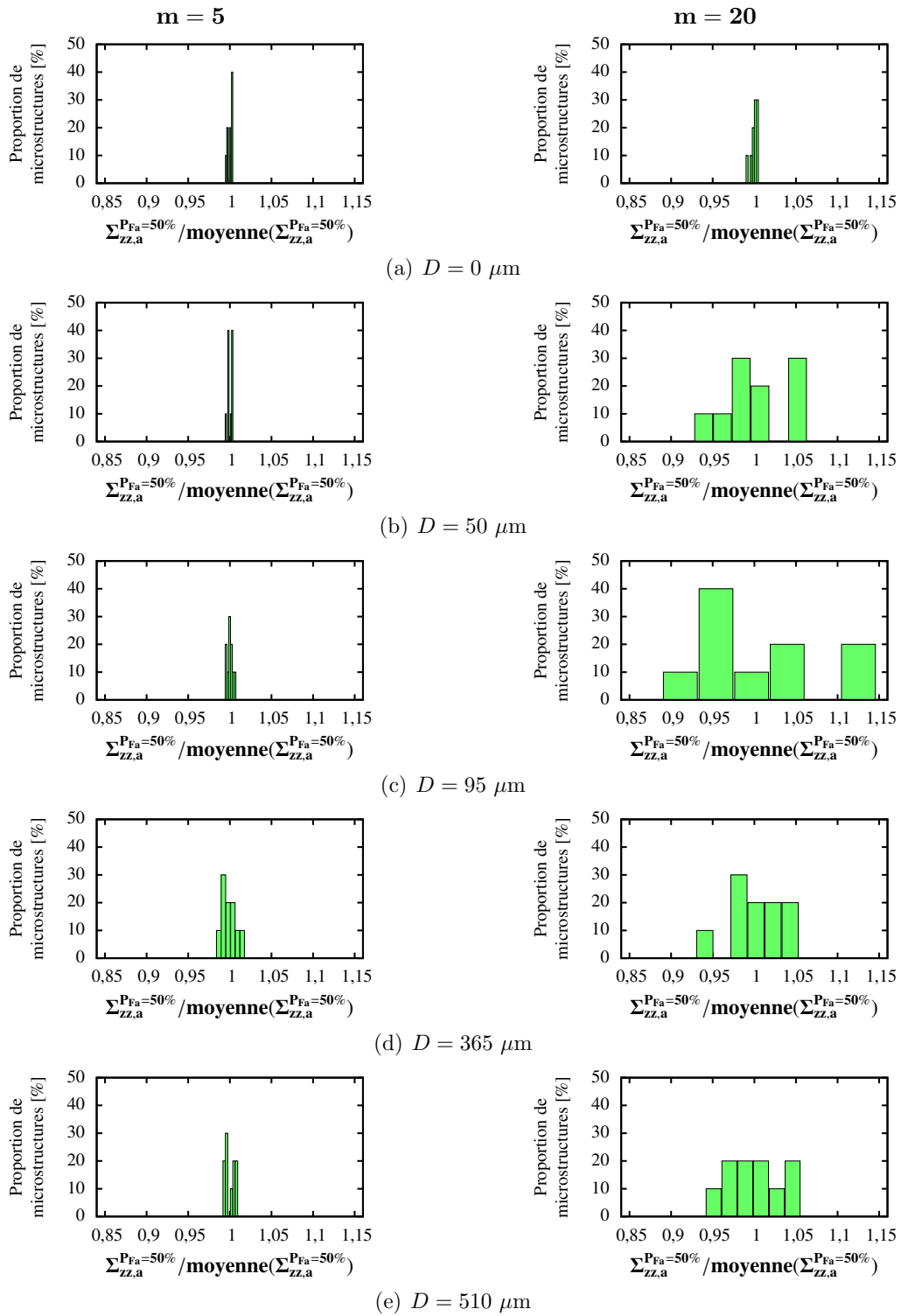
FIGURE V.16 – Histogrammes des limites de fatigue à P_{Fa} = 50\% des microstructures en 2D sollicitées en traction alternée symétrique obtenus avec un comportement des grains élastique cubique, pour différentes valeurs du paramètre de forme m et diamètre de trou D .
