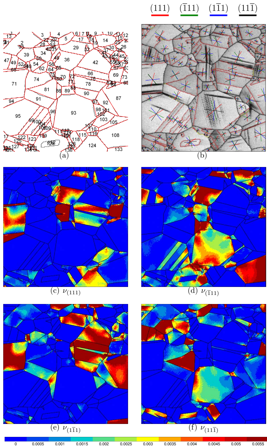
FIGURE IV.19 – Résultats de la région n°2 de l'éprouvette sollicitée en torsion : représentation (a) de la numérotation des grains, (b) des traces des plans de glissement et de la somme des glissements plastiques cumulés dans le plan : (c) (111) , (d) (\bar{1}\bar{1}1) , (e) (1\bar{1}\bar{1}) et (f) (11\bar{1}) .
