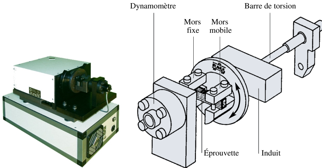
FIGURE IV.1 – Machine d'essai de fatigue électromécanique à résonance Rumul CrackTronic équipée du montage de flexion plane.
