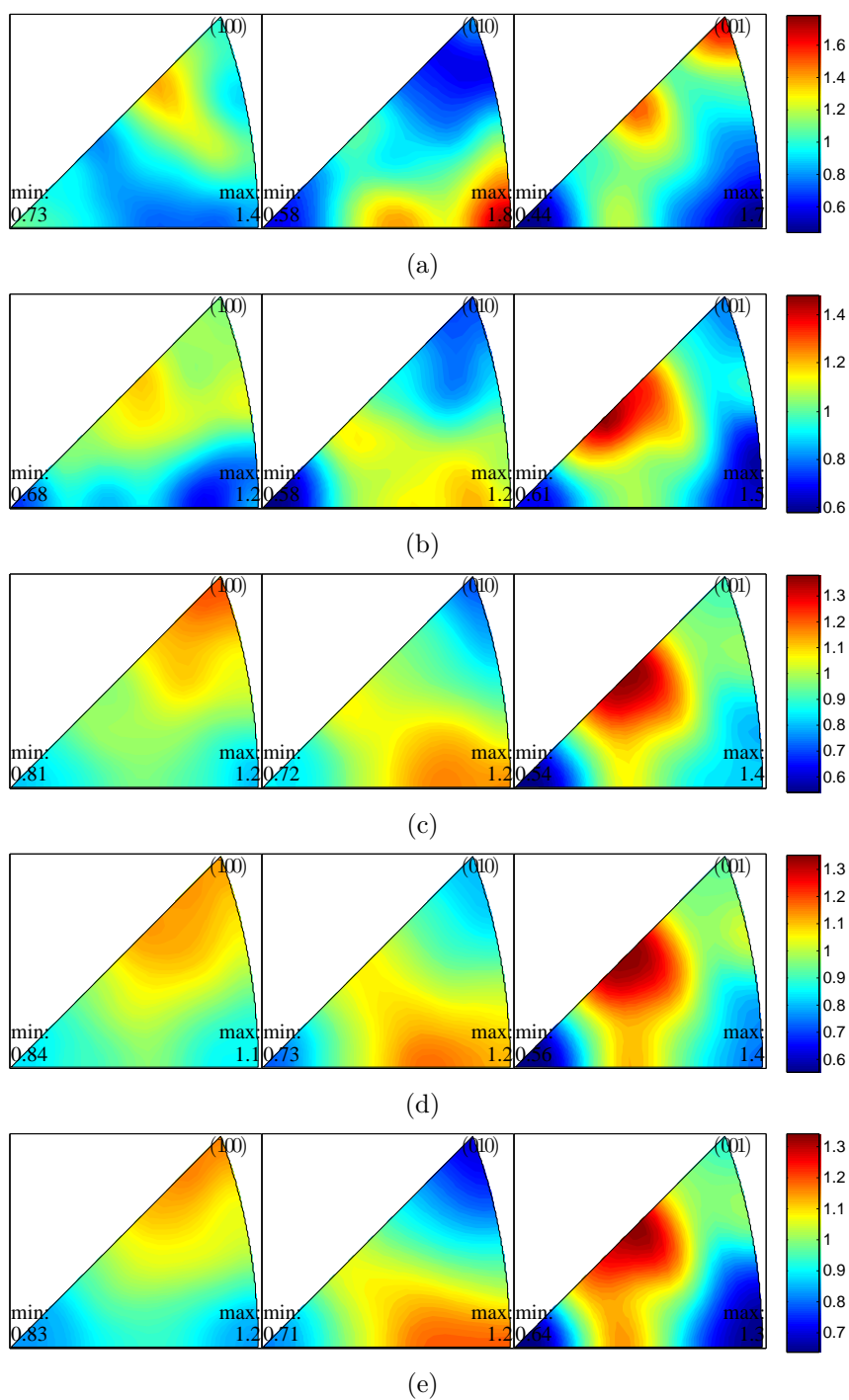
FIGURE A.12 – Figures de pôles inverses des axes x , y et z de l'échantillon obtenues à partir des jeux d'orientations pour N^* égal à : a) 300, b) 1000, c) 10000, d) 20000, e) 30000.
