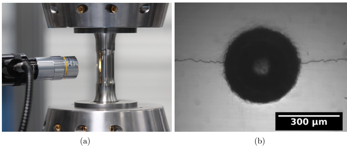
FIGURE III.23 – Observation de l'éprouvette tubulaire au vidéo-microscope : (a) montage du vidéo-microscope et (b) exemple d'observation au vidéo-microscope d'un défaut hémisphérique de 365 \mu\text{m} de diamètre.
