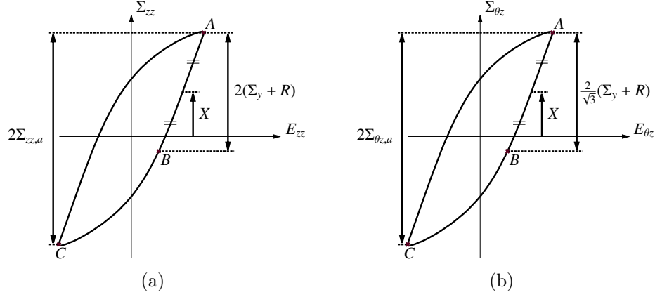
FIGURE III.9 – Schématisation d'un cycle de chargement (a) en traction-compression uniaxiale dans un diagramme \Sigma_{zz} - E_{zz} et (b) en torsion alternée dans un diagramme \Sigma_{\theta z} - E_{\theta z} .
