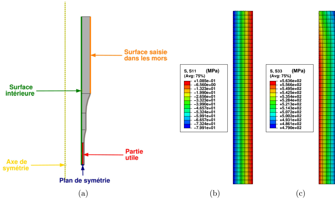
FIGURE III.20 – (a) Géométrie de l'éprouvette tubulaire dans le modèle EF et champs de contrainte dans la partie utile de l'éprouvette lors d'un essai de pression interne à P = 800 bars : (b) \Sigma_{rr} et (c) \Sigma_{\theta\theta} .
