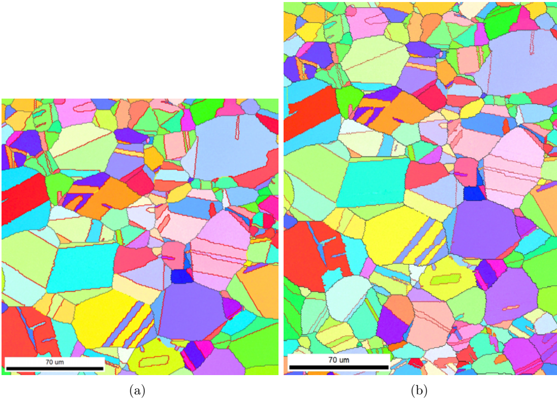
FIGURE E.4 – Cartographies d’orientation en figure de pôle inverse dans la région n° 2 de l’éprouvette sollicitée en torsion : (a) avant sollicitation et (b) après sollicitation.
