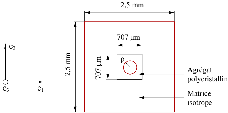
FIGURE II.14 – Géométrie des microstructures trouées.
