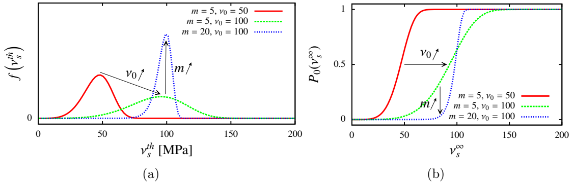
FIGURE I.5 – Illustration de la loi de probabilité de Weibull pour différentes valeurs des paramètres d'échelle \nu_0 et de forme m : (a) densité de probabilité et (b) fonction de répartition.
