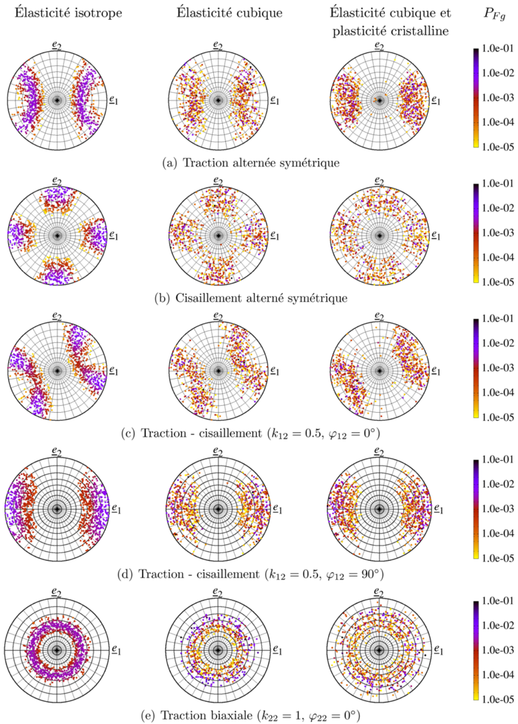
FIGURE II.7 – Projection stéréographique, dans le plan de normal \underline{e}_3 , du vecteur normal unitaire du plan de glissement le plus critique de chaque grain et probabilité de rupture P_{Fg} associée.
