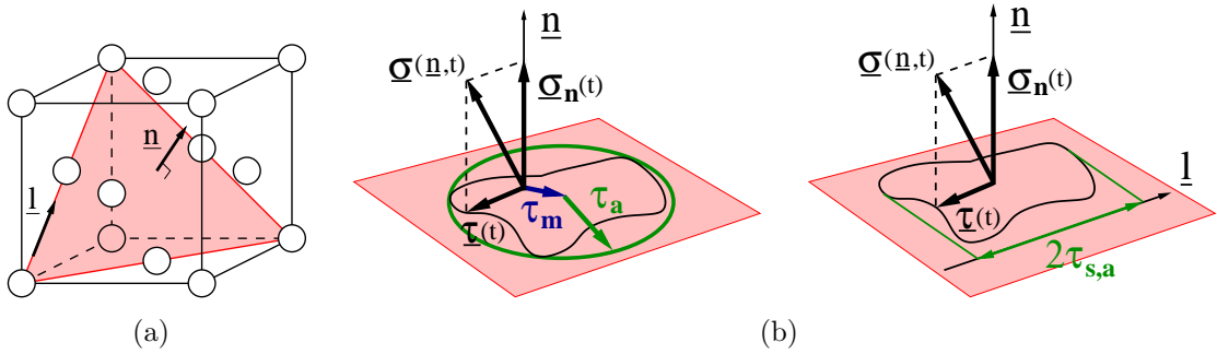
FIGURE II.2 – Représentation de quelques quantités mécaniques et vecteurs utilisées par les critères de fatigue : (a) normale au plan de glissement \underline{n} et direction de glissement \underline{l} dans une maille cubique à faces centrées et (b) vecteurs de contrainte \underline{\sigma} , de contrainte normale \underline{\sigma}_n et de cisaillement \underline{\tau} dans un plan de glissement.
