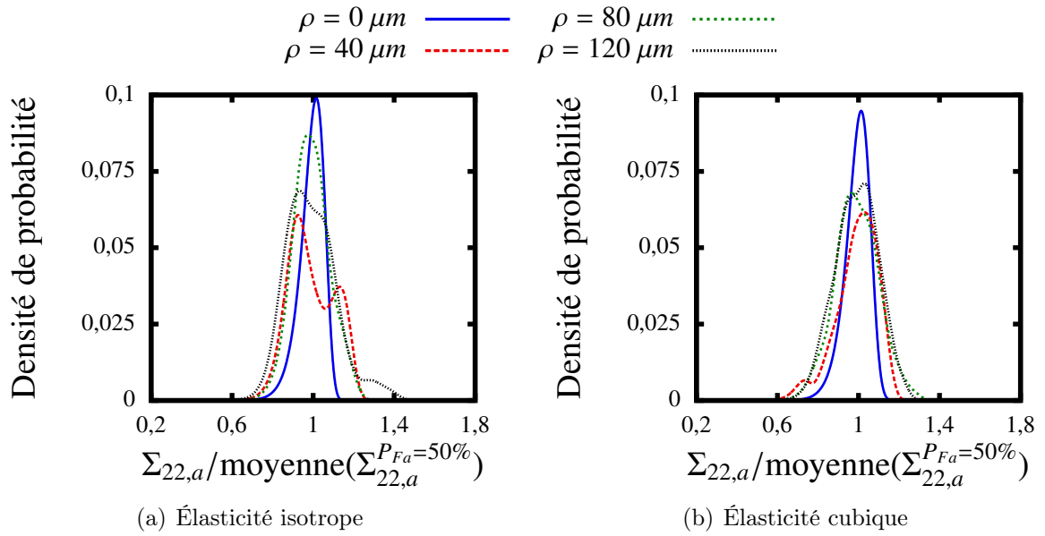
FIGURE II.25 – Distributions complètes de la limite de fatigue macroscopique \Sigma_{22,a} décrite par la densité de probabilité f_{moy} pour différents rayons d'entaille \rho et avec un comportement des grains : (a) élastique isotrope et (b) élastique cubique.
