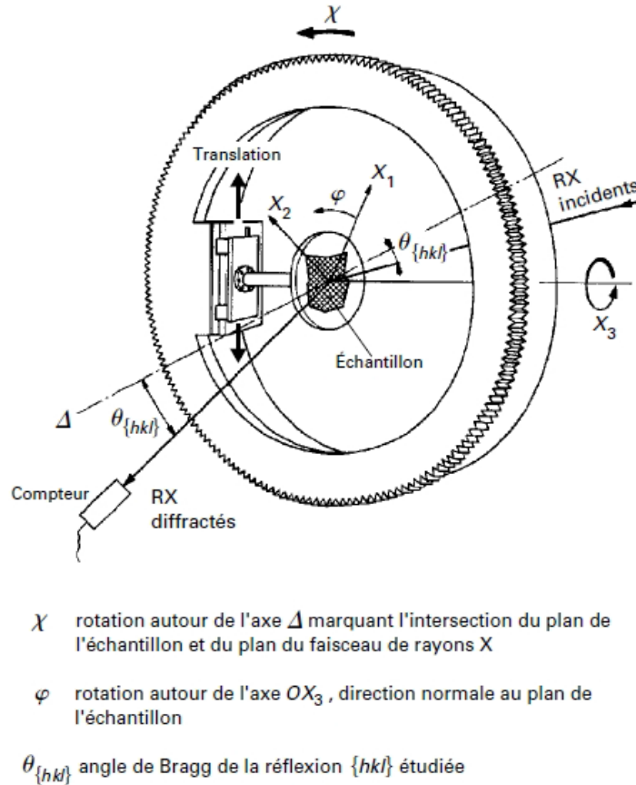
FIGURE A.6 – Montage en réflexion avec un goniomètre de texture [157]
