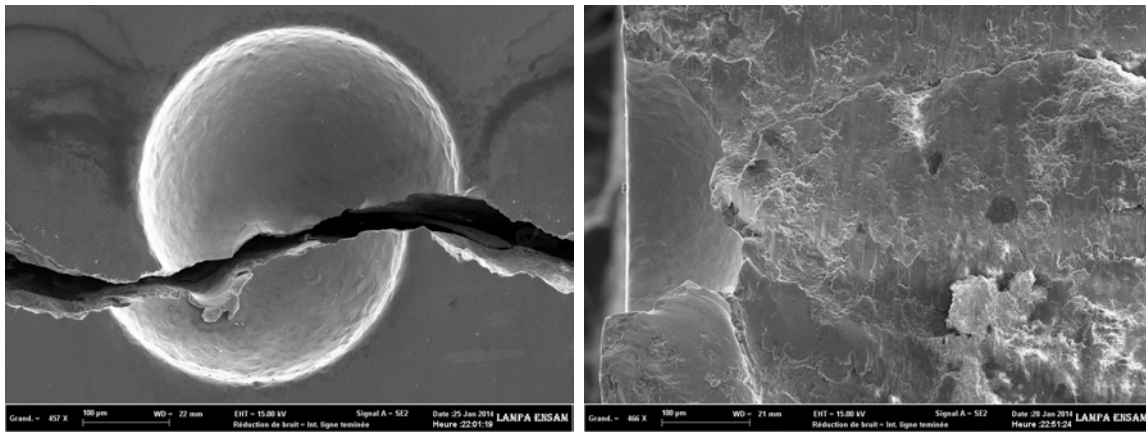
FIGURE III.33 – Micrographies du défaut et du faciès de rupture d'une éprouvette sollicitée en traction-torsion alternées symétriques déphasées ( k_{\theta z} = 0,5 et \varphi_{\theta z} = 90^\circ ) avec un défaut de diamètre D = 365 \mu\text{m} .
