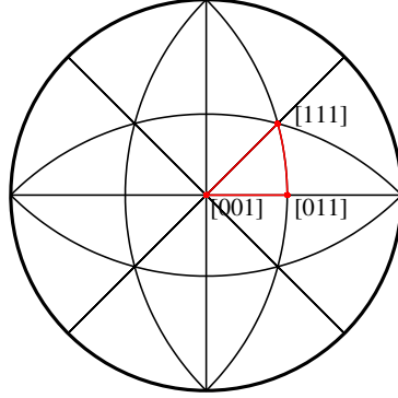
FIGURE A.4 – Symétries dans les figures de pôles inverses pour les réseaux cubiques.
