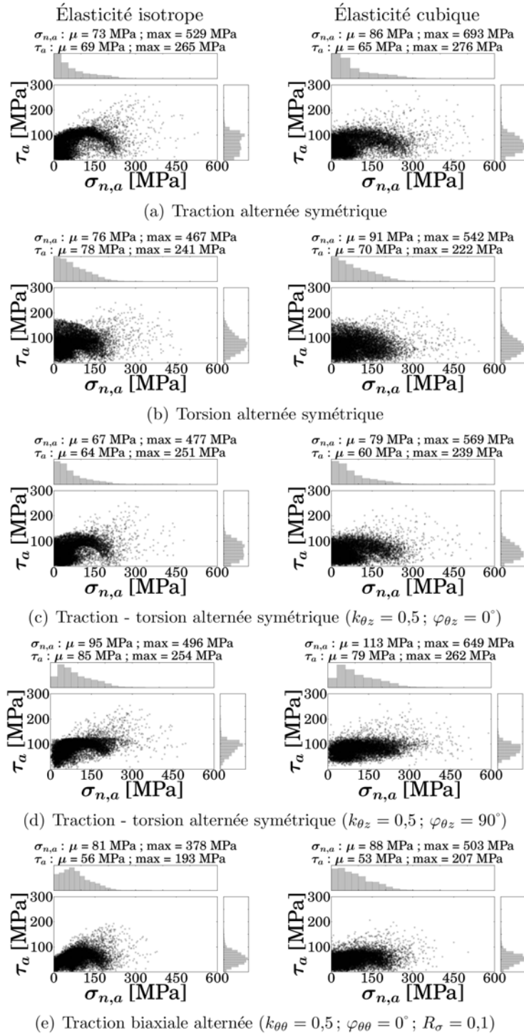
FIGURE V.8 – Réponses mécaniques, en termes de \tau_a - \sigma_{n,a} , de chaque plan de glissement obtenues à partir des simulations par EF sur les microstructures en 2D présentant un trou de diamètre D = 365 \mu\text{m} sollicitées, au niveau de la limite de fatigue moyenne, par différents types de chargement.
