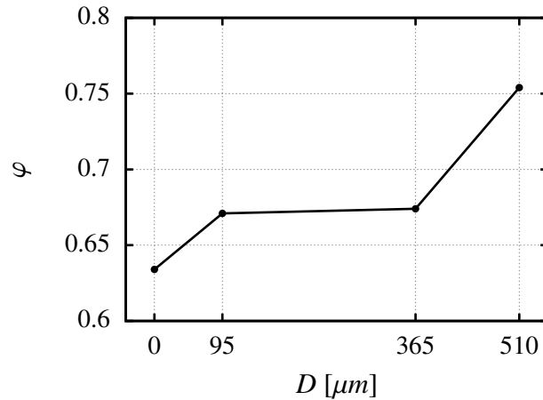
FIGURE III.38 – Évolution du rapport \varphi observé expérimentalement sur l'acier austénitique 316L en fonction du diamètre D du défaut.
