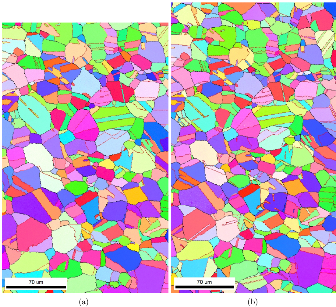
FIGURE E.3 – Cartographies d'orientation en figure de pôle inverse dans la région n° 1 de l'éprouvette sollicitée en torsion : (a) avant sollicitation et (b) après sollicitation.
