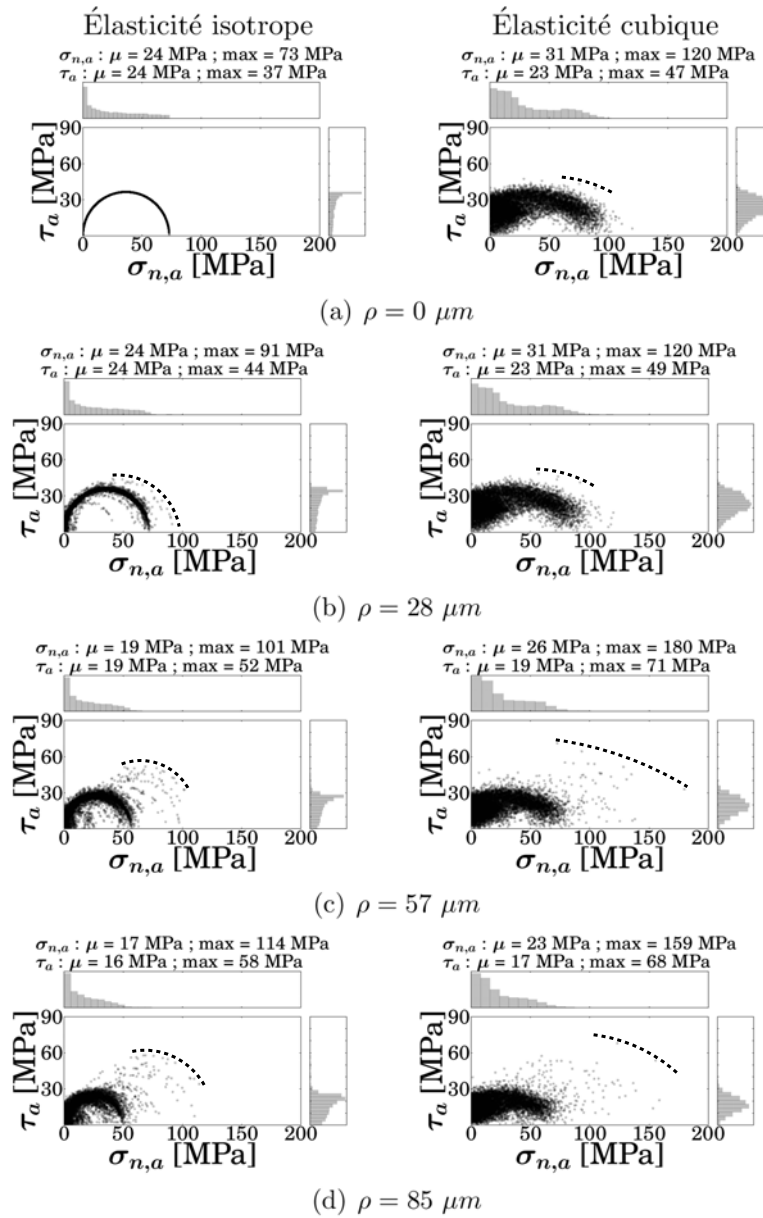
FIGURE II.26 – Réponses mécaniques, en termes de \tau_a - \sigma_{n,a} , de chaque plan de glissement obtenues à partir des simulations par EF sur les microstructures trouées sollicitées en traction alternée symétrique à la limite de fatigue moyenne. Les lignes pointillées indiquent l'enveloppe maximale des points.
