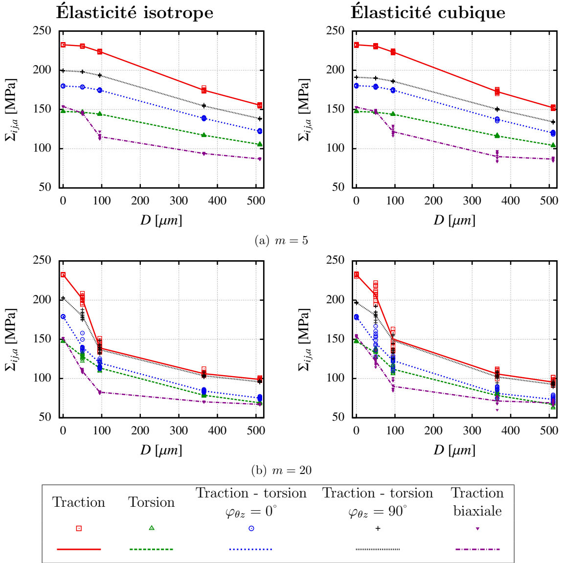
FIGURE V.15 – Limites de fatigue macroscopiques à P_{Fa} = 50\% de chaque microstructure (points) et moyenne de ces limites de fatigue (ligne) pour différentes sollicitations, pour différents diamètres de trou D et pour chaque modèle de comportement élastique.
