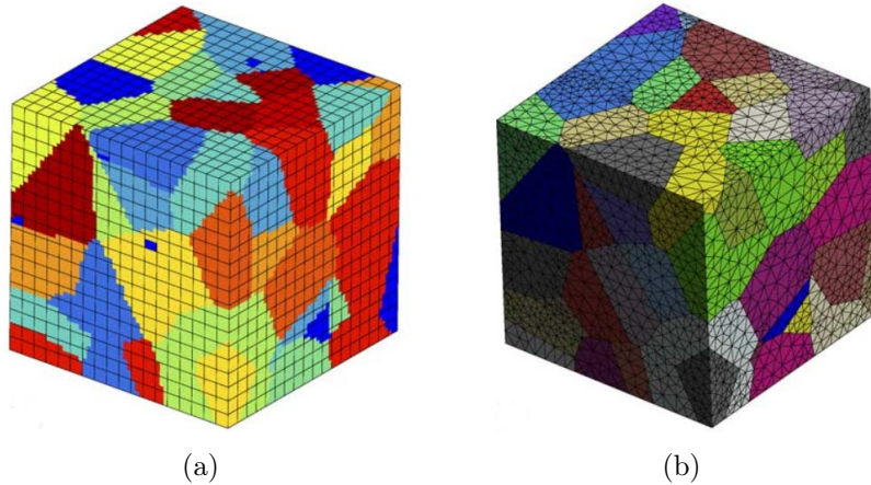
FIGURE I.7 – Exemple de maillage d'un agrégat polycristallin : (a) maillage régulier et (b) maillage libre [3].
