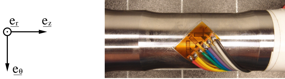
FIGURE III.3 – Éprouvette tubulaire instrumentée d'une rosette à 3 jauges d'extensométrie à 45°.
