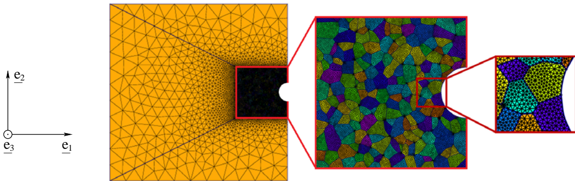
FIGURE II.13 – Exemple de maillage d'une matrice et d'un agrégat polycristallin entaillé de 200 grains en 2 dimensions.
