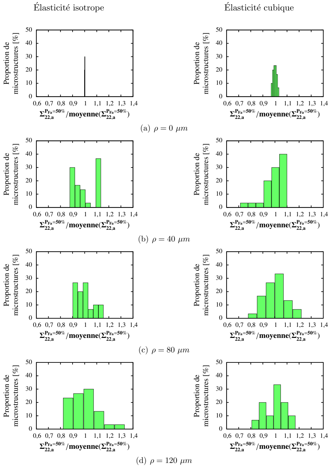
FIGURE II.22 – Histogrammes des limites de fatigue à P_{Fa} = 50\% des microstructures entaillées pour différents rayons d'entaille \rho et pour chaque modèle de comportement élastique.
