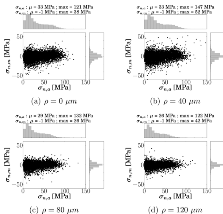
FIGURE II.18 – Réponses mécaniques, en termes de \sigma_{n,m} - \sigma_{n,a} , de chaque plan de glissement obtenues à partir des simulations par EF sur les microstructures entaillées, utilisant le modèle de plasticité cristalline, sollicitées en traction alternée symétrique à la limite de fatigue moyenne. Les lignes pointillées indiquent l'enveloppe maximale des points.
