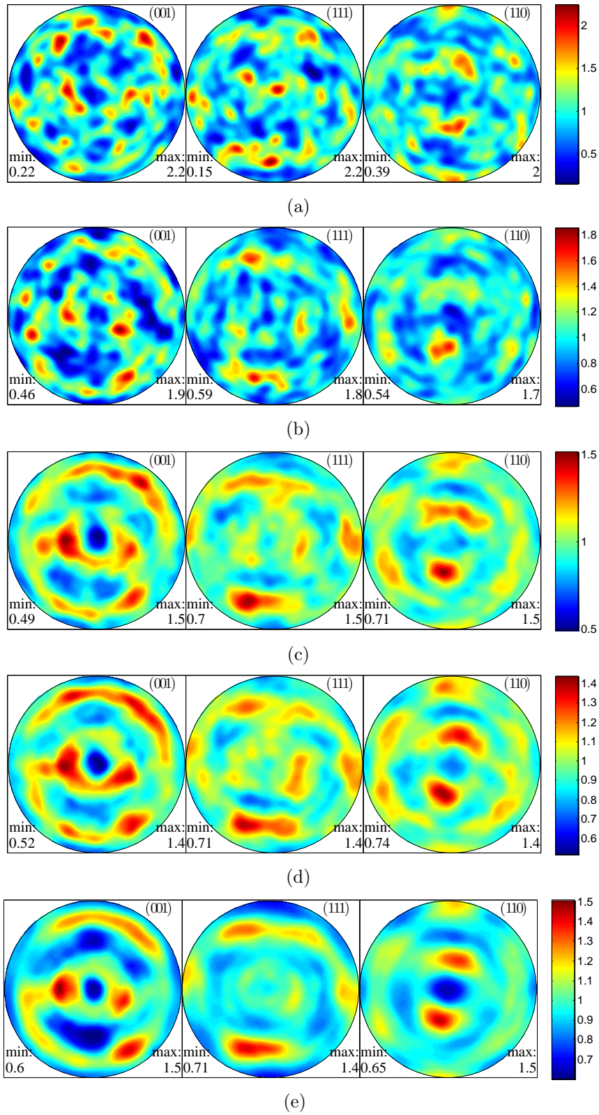
FIGURE A.11 – Figures de pôles \{200\} , \{111\} et \{220\} obtenues à partir des jeux d'orientations pour N^* égal à : a) 300, b) 1000, c) 10000, d) 20000, e) 30000.
