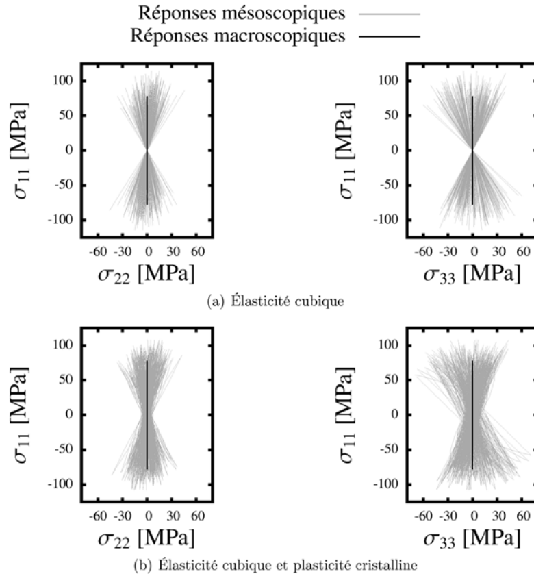
FIGURE II.5 – Comparaison entre les réponses \sigma_{11} - \sigma_{22} et \sigma_{11} - \sigma_{33} macroscopiques et mésoscopiques d'un agrégat polycristallin sollicité à la limite de fatigue en traction alternée symétrique pour : (a) l'élasticité cubique seule et (b) l'élasticité cubique avec la plasticité cristalline.
