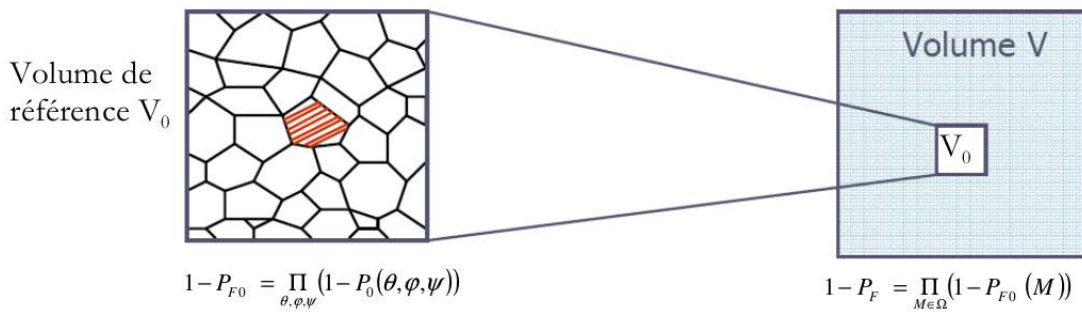
FIGURE I.6 – Application de l'hypothèse du maillon le plus faible sur le volume de la structure V .
