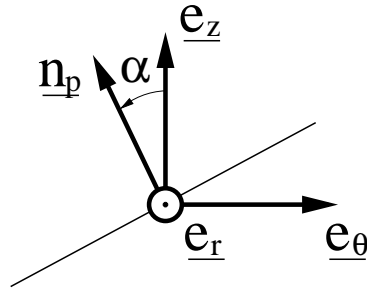
FIGURE III.27 – Orientation du plan de propagation de la fissure macroscopique dans le repère cylindrique de l'éprouvette.
