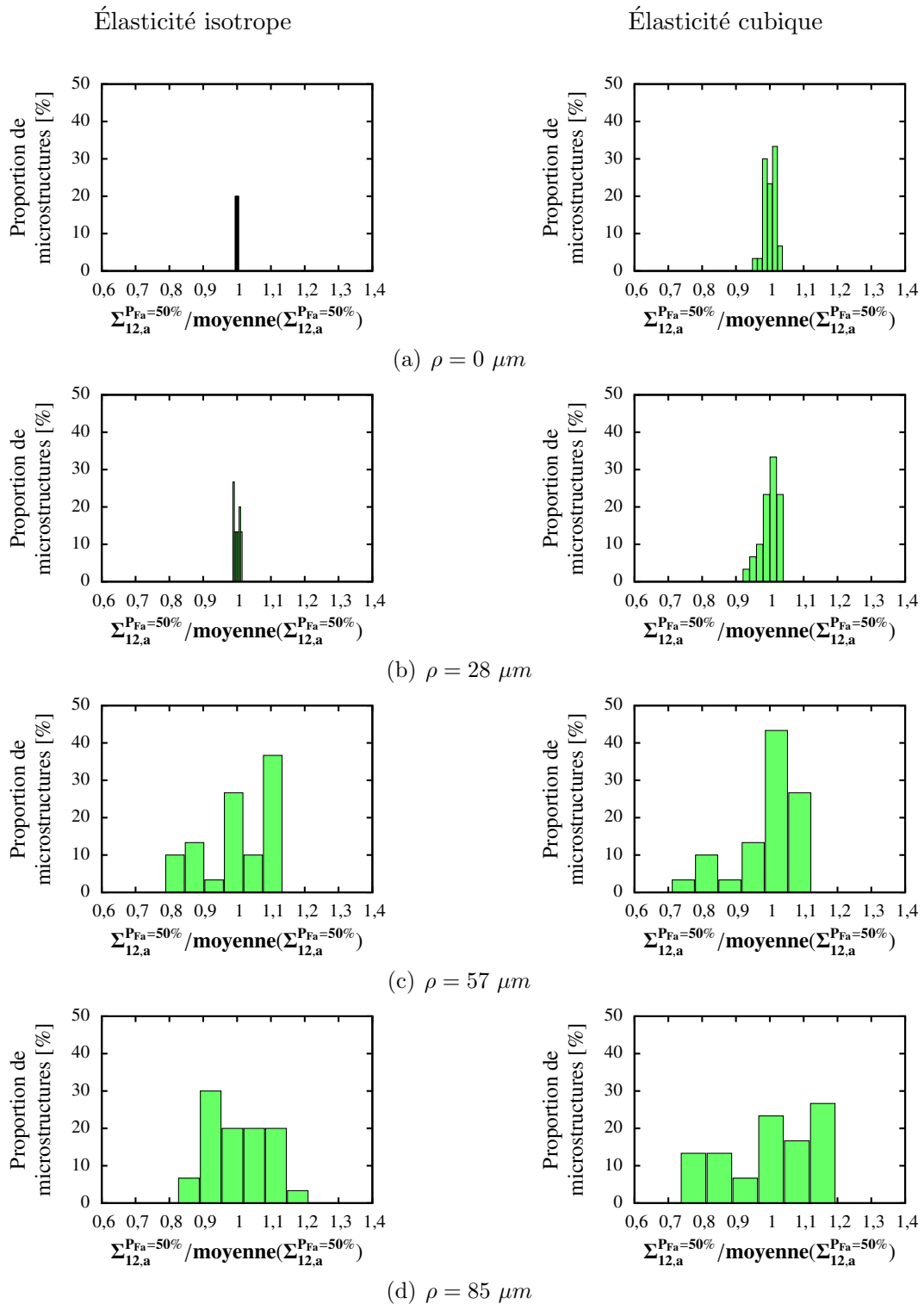
FIGURE II.34 – Histogrammes des limites de fatigue à P_{Fa} = 50\% des microstructures trouées sollicitées en cisaillement alterné symétrique pour différents rayons de trou \rho et pour chaque modèle de comportement élastique.
