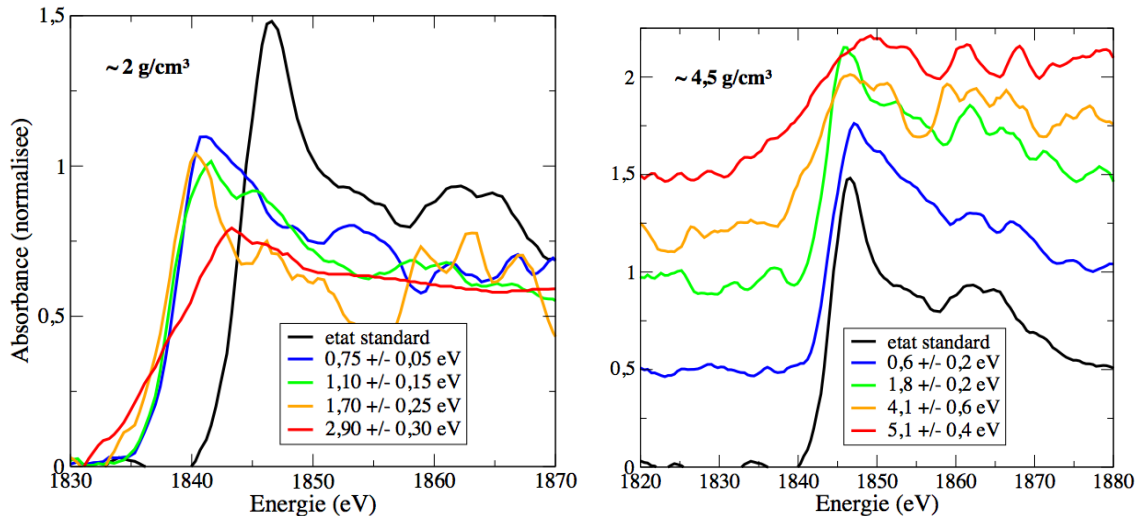
FIGURE 3.20: Illustration de l'influence de la température sur le flanc K de la silice le long des isochores 2 \text{ g/cm}^3 (à gauche) et 4,5 \text{ g/cm}^3 (à droite). Les spectres à 4,5 \text{ g/cm}^3 ont été décalés verticalement par soucis de lisibilité.
