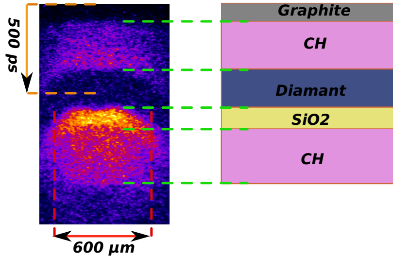
FIGURE 3.7: Image typique du diagnostic d'émission propre utilisé pour suivre temporellement l'émission en face arrière de la cible choquée, ici de type « détente ». Exception faite de la première couche de graphite choisie opaque pour permettre de protéger les systèmes optiques de l'émission directe du laser de puissance, il est possible de suivre précisément l'émission des quatre autres couches transparentes et ainsi d'en déduire la vitesse moyenne du choc dans chacune de ces couches.
