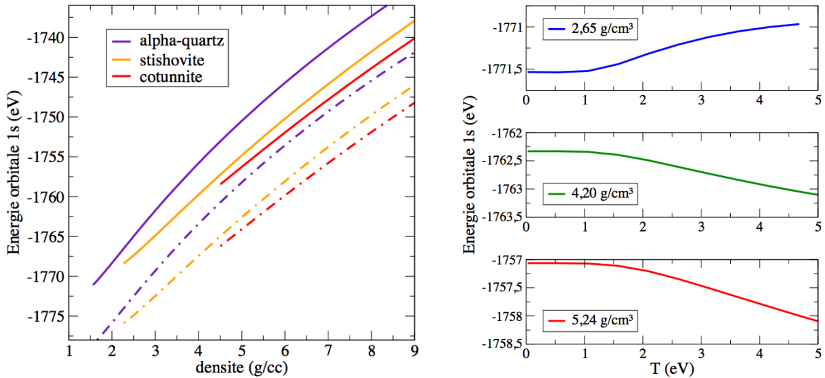
FIGURE 2.7: Evolution de l'énergie de l'orbitale 1s de l'atome de silicium en fonction de la densité (à gauche) et de la température (à droite). Ces calculs ont été réalisés avec un pseudo-potential « tous-électrons », ici en utilisant l'approximation LDA (trait plein) ou GGA (trait pointillé), et montrent l'influence à la fois de la densité et de la température, mais aussi de la phase, sur l'orbitale de coeur.
