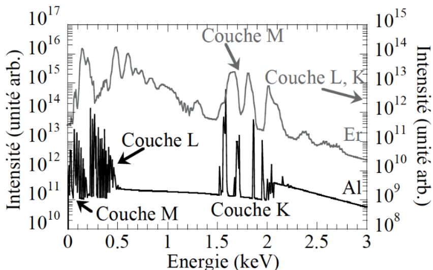
FIGURE 1.17: Comparaison des spectres d'émission de plasma d'Aluminium ( Z = 13 ) et d'Erbium ( Z = 68 ), obtenus avec le code Averroes - Transpec , pour T_e = 400 eV et N_e = N_c = 1,7 \cdot 10^{21} e - /cm -3 [76].
