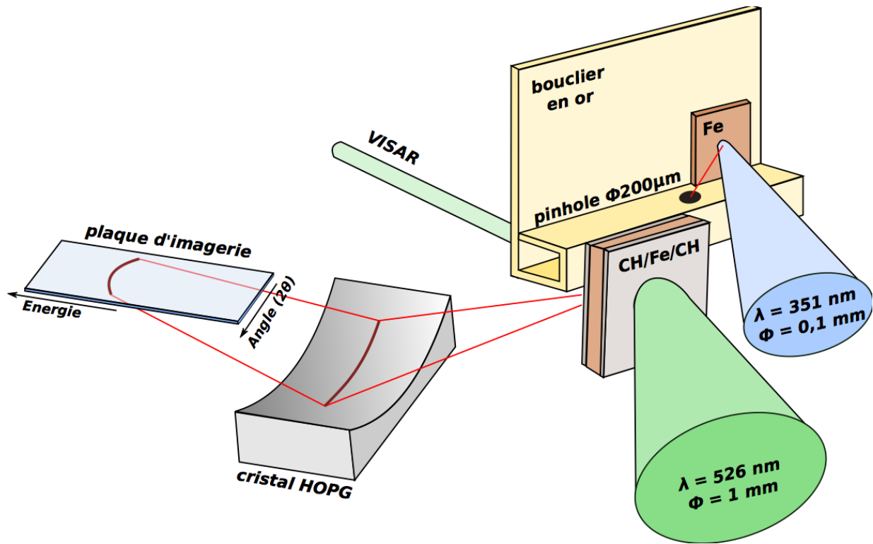
FIGURE 6.13: Disposition des diagnostics dans l'enceinte d'expérience GEKKO XII pour les expériences de diffraction X en réflexion. La taille de l'enceinte permet d'utiliser le cristal cylindrique HOPG au premier ordre et de collecter du signal diffracté sur une plage angulaire de 24^\circ . La diffraction se faisant en face arrière de la cible principale, l'épaisseur de cette dernière, associée à un délai entre la sonde et la pompe bien choisis, permet de sonder le fer dans un état choqué relativement homogène, même avec une sonde de durée proche de 1,6\ \text{ns} . Les protections entourant le cristal et le protégeant des radiations provenant du laser de compression ne sont pas représentées ici par souci de clarté.
