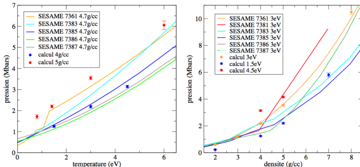
FIGURE 3.8: Un choix était à faire parmi de nombreuses EOS du \text{SiO}_2 : seule l'EOS 7361 semble être en accord avec les résultats de nos calculs ab initio , à la fois le long de l'isochore 4,7 g/cm 3 (à gauche) et le long de l'isotherme 3 eV (à droite).
