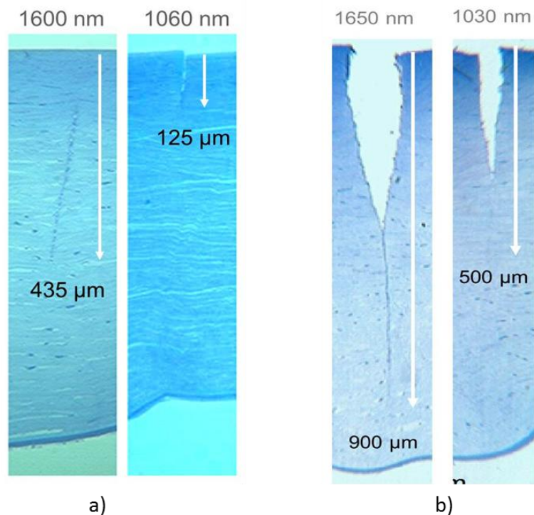
Figure 5-6 Comparaison directe des découpes à 1600 nm et 1000 nm, en utilisant la source OPA avec une énergie de 1 \mu\text{J} et une ouverture numérique de 0,4 a) et comparaison directe des découpes à 1650 nm et 1030 nm en utilisant la source OPG avec une énergie de 2 \mu\text{J} et une ouverture numérique de 0,56 b).
