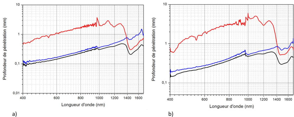
Figure 3-25 Profondeur de pénétration pour les différentes composantes en fonction de la longueur d'onde pour deux échantillons de sclère de pleine épaisseur (environ 600 µm), immergé dans une solution contenant 75% de glycérol et 25% de solution saline a) et immergé dans une solution à 100 % de glycérol b).
