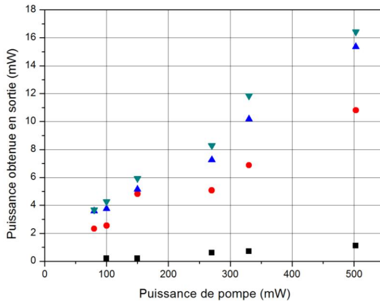
Figure 4-17 Puissance obtenue en sortie du cristal en configuration OPG (carré noir), en configuration OPA avec injection de la totalité du signal généré au 1 er étage (cercle rouge), en configuration OPA avec injection du signal généré au 1 er étage filtré à 1600 nm +/- 25 nm (triangle bleu pointant vers le haut) et en configuration OPA avec injection du signal généré au 1 er étage filtré à 1600 nm +/- 5 nm (triangle vert vers le bas).
