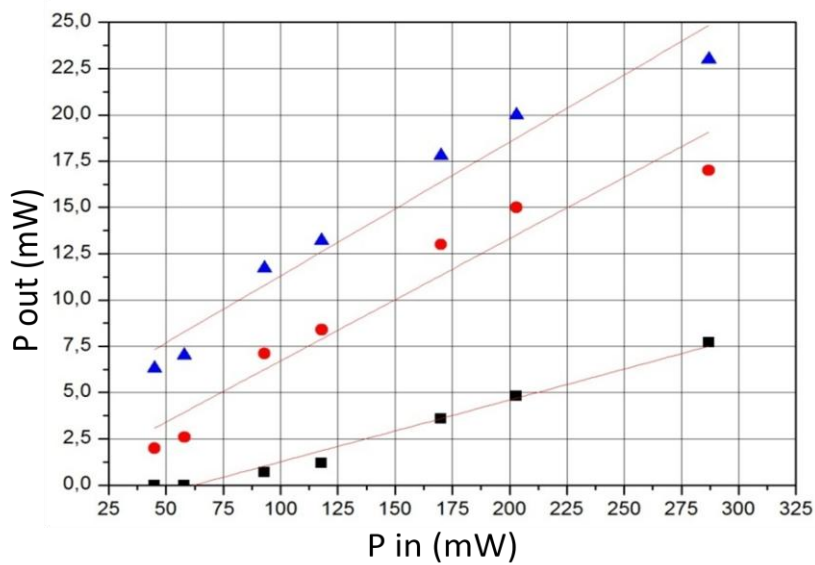
Figure 4-16 Puissance mesurée en sortie du cristal amplificateur : en configuration OPG (carrés noirs), en pompant avec un signal filtré à 1650 nm +/- 25 nm (points rouges) et sans filtrage du bras initiateur des photons (triangles bleus).
